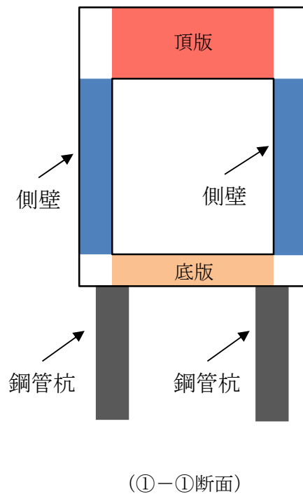
図 2.16-1 緊急時対策所用発電燃料油貯蔵タンク基礎の照査位置図
