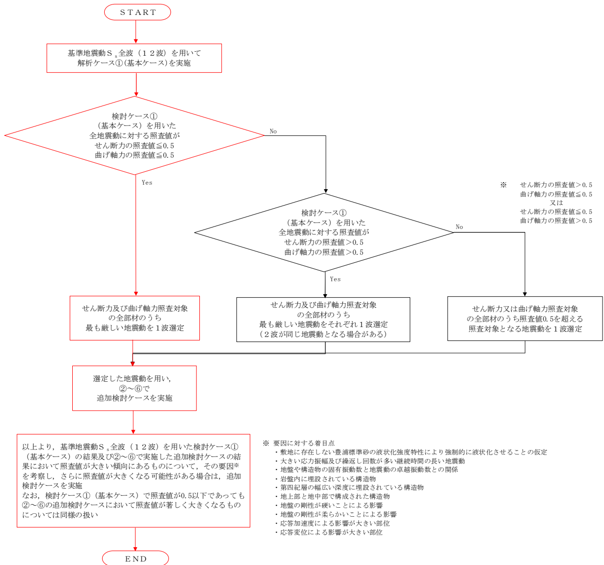
図 2.14-2 地震動選定フロー (②-②断面 (鋼製管))
