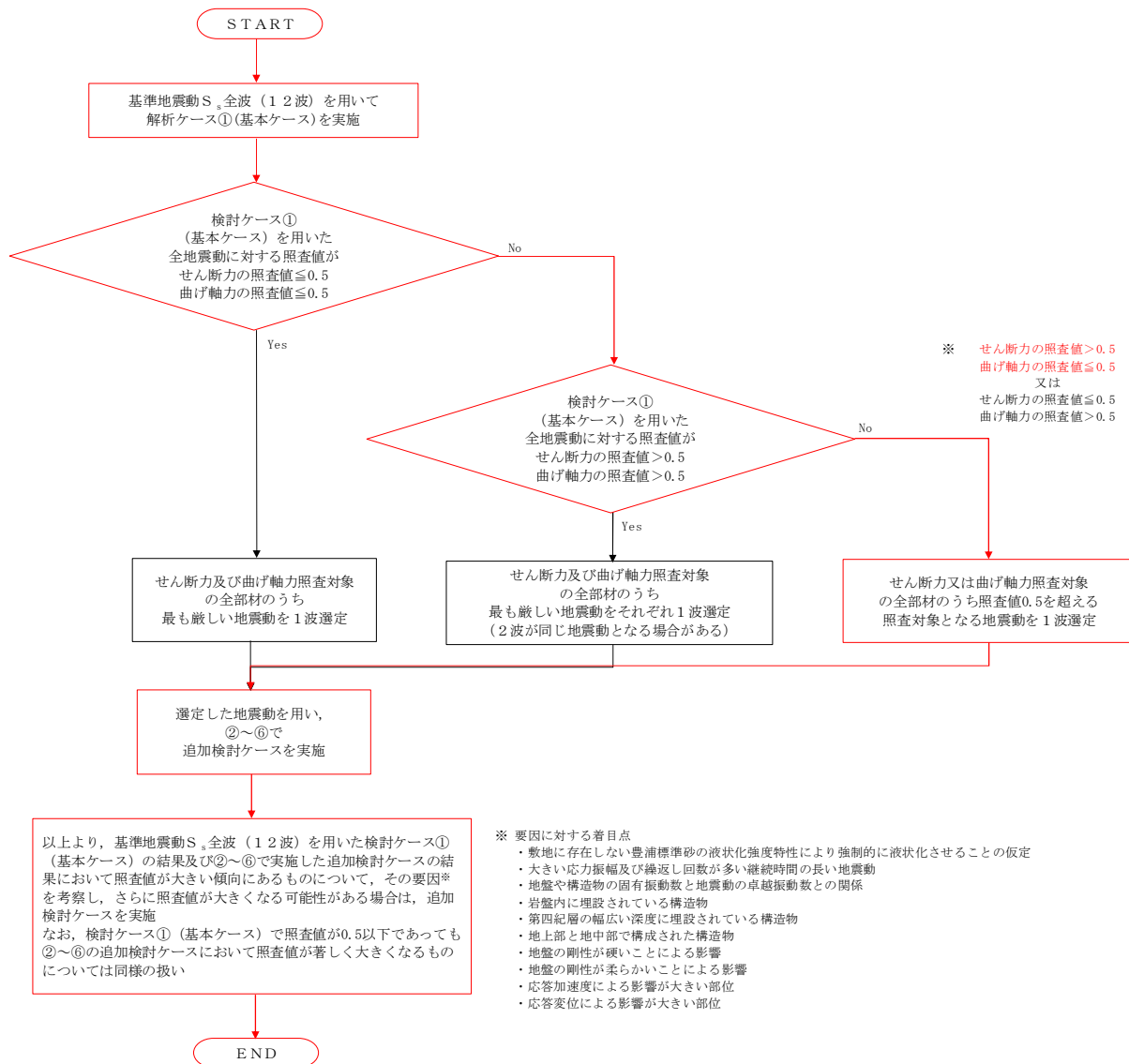
図 2.1-7 地震動選定フロー (⑥-⑥断面 (鋼管杭))
