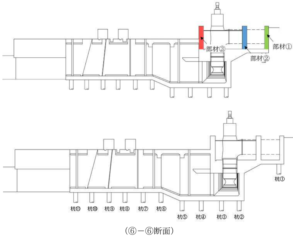
図 2.1-1(2) 取水構造物の照査位置図
