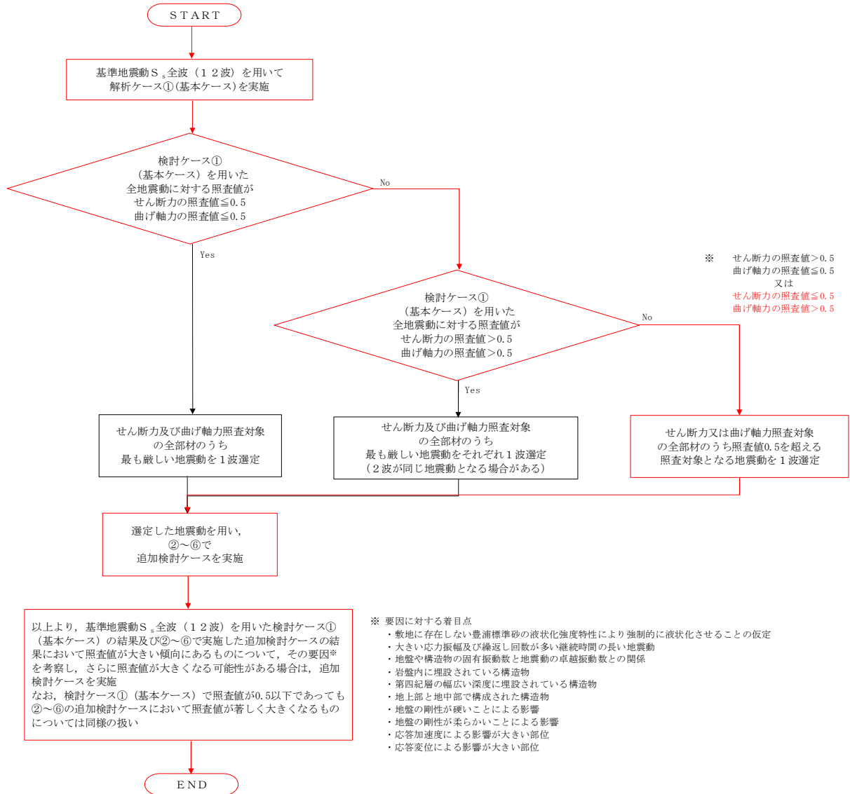
図 2.16-5 地震動選定フロー (①-①断面 (鋼管杭))
