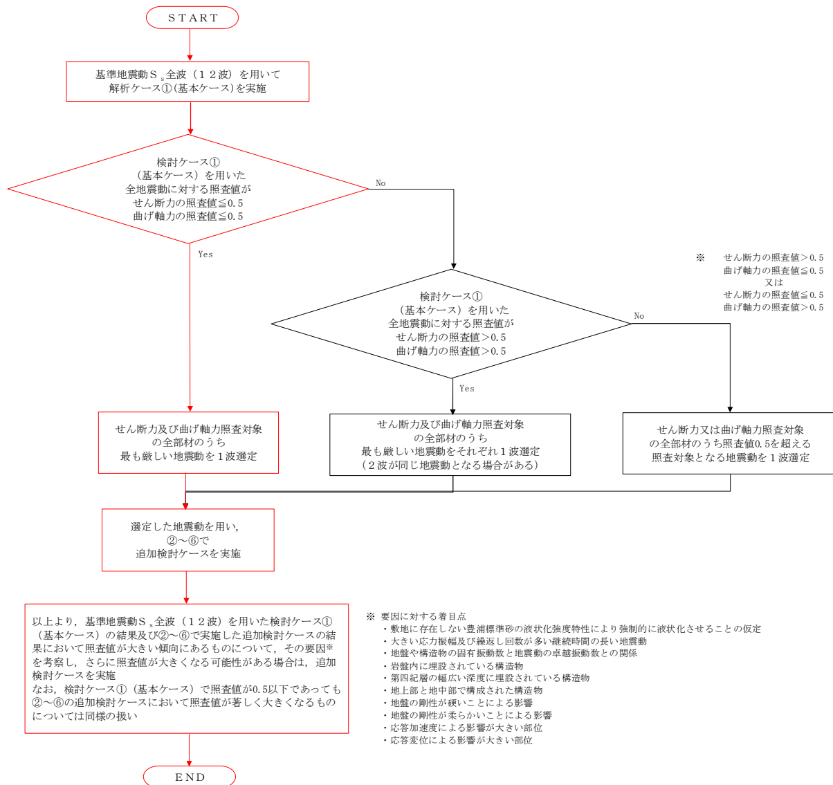
図 2.17-5 地震動選定フロー (①-①断面(鋼管杭))
