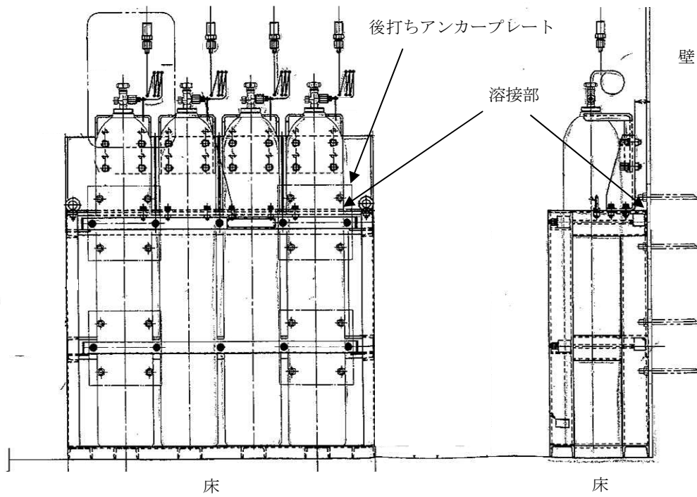
図2-2 ボンベ設備（壁掛床置形）
