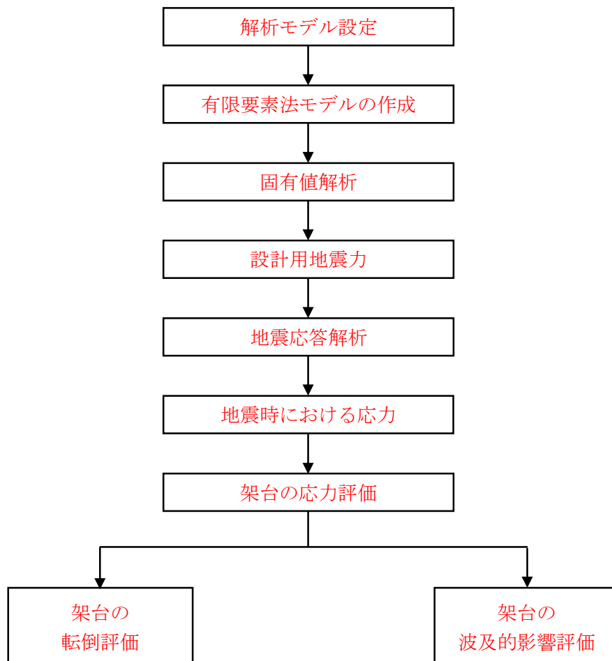
図 4-10 その他設備の架台の耐震評価フロー
