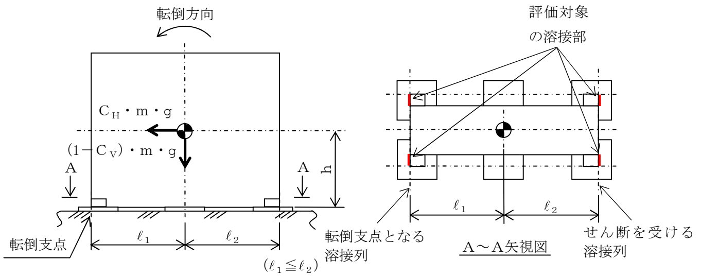
図(5.2) 計算モデル (短辺方向転倒-2 (1 - C_V) < 0 の場合)
