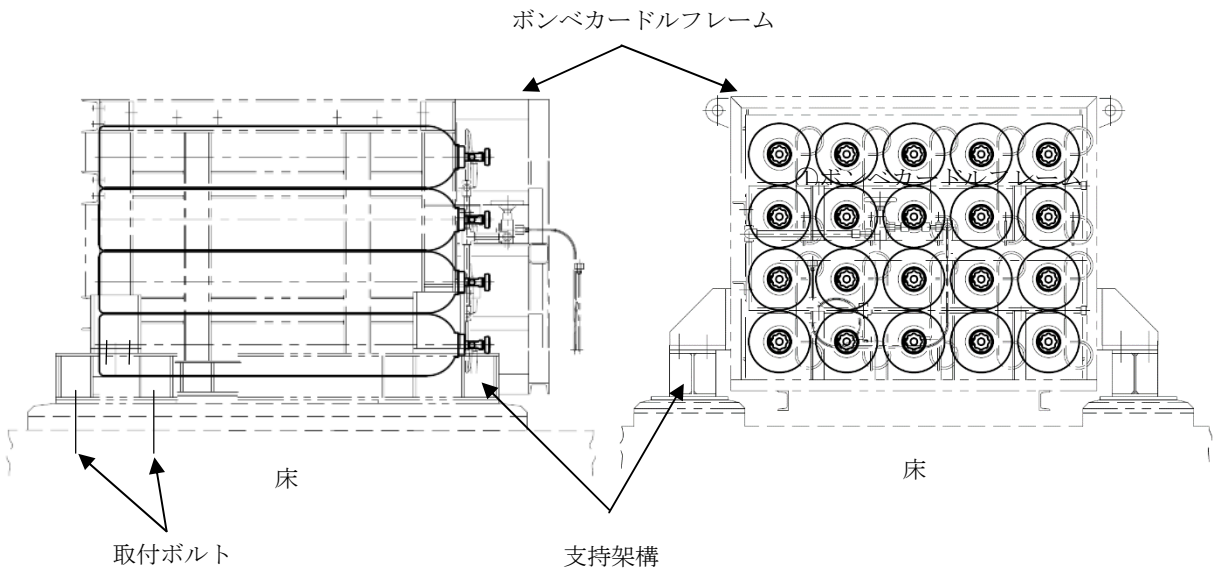
図2-4 ポンベ設備 (カード形)
