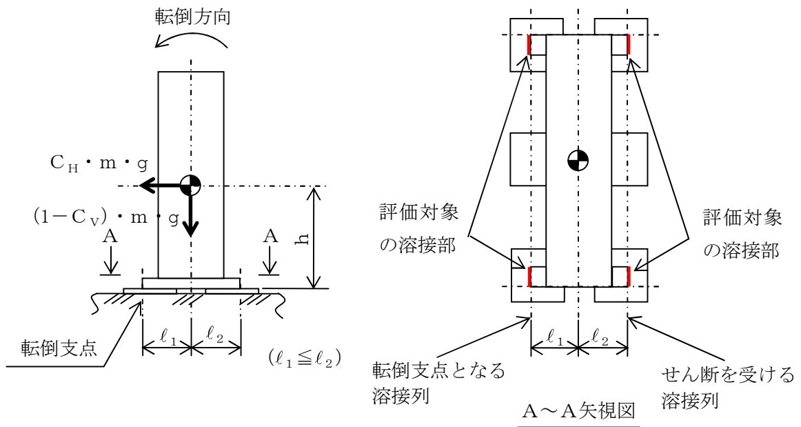
図(5).1 計算モデル (短辺方向転倒-1 (1 - C_V) \geq 0 の場合)
