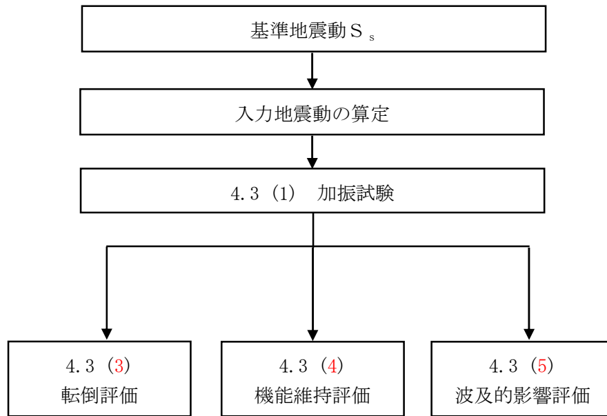
図4-9 その他設備の耐震評価フロー
