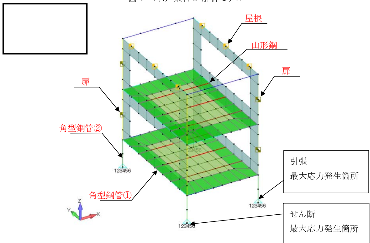
図 4-1(5) 架台 5 解析モデル
