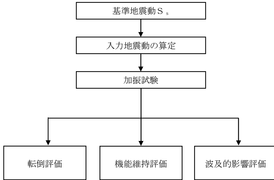
図 2-5 その他設備の耐震評価フロー
