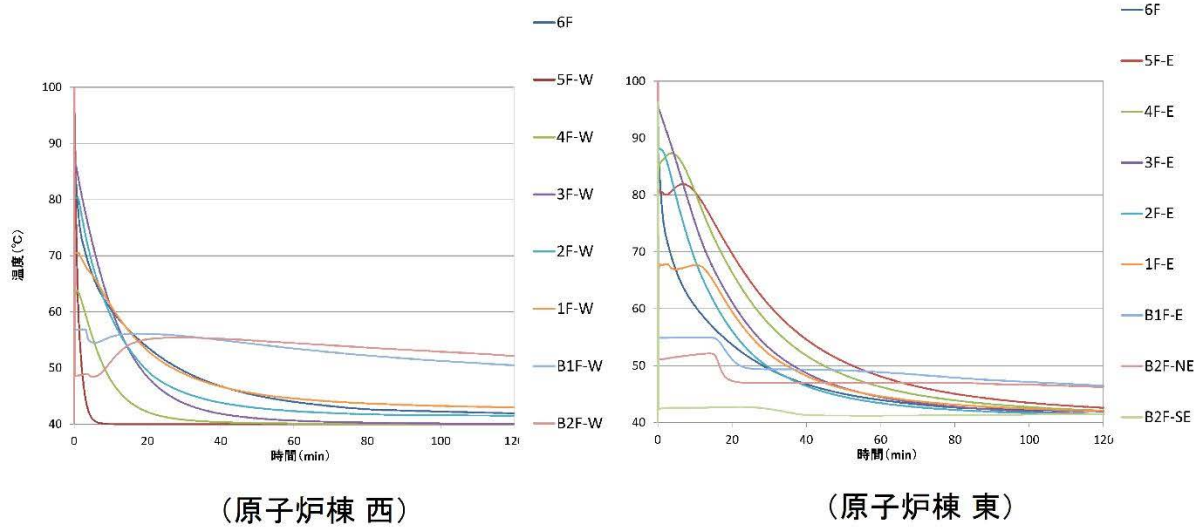
第9図 対策後の温度状況比較
