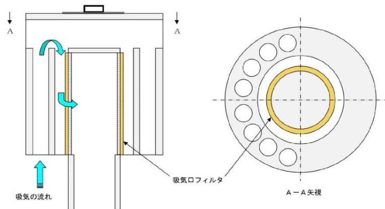
非常用ディーゼル発電機（高圧炉心スプレー系ディーゼル発電機を含む。）吸気フィルタ（既設）
