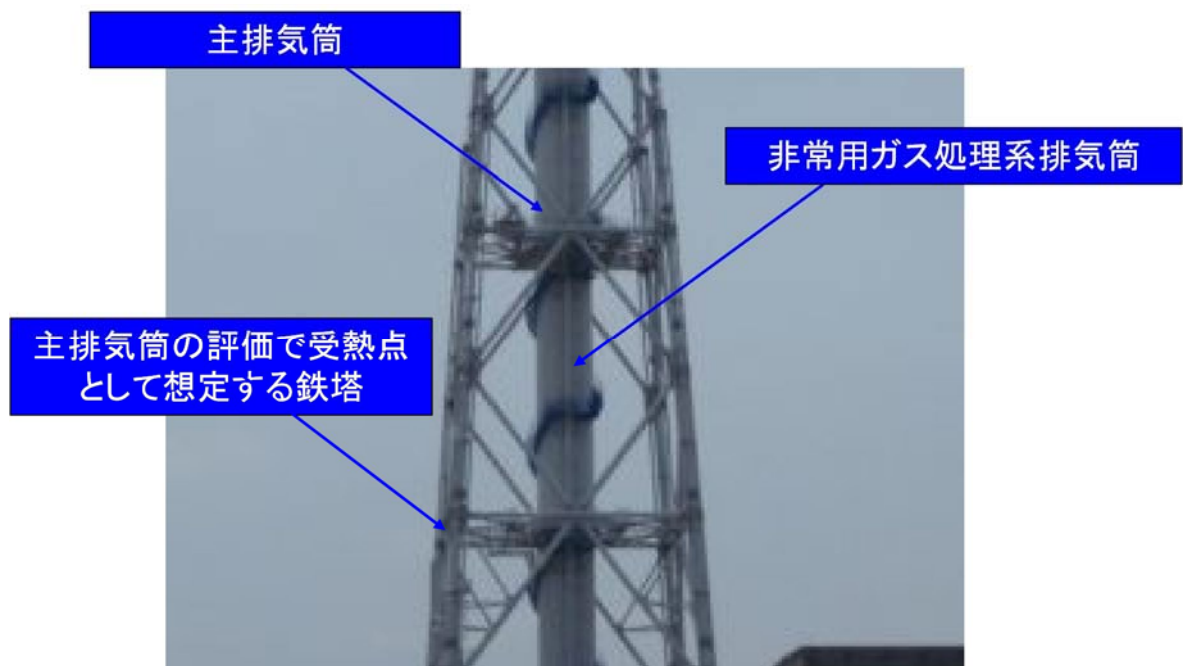
第 2-4 図 非常用ガス処理系排気筒と主排気筒の位置
