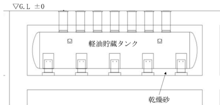
第1図 軽油貯蔵タンクの地下化イメージ
