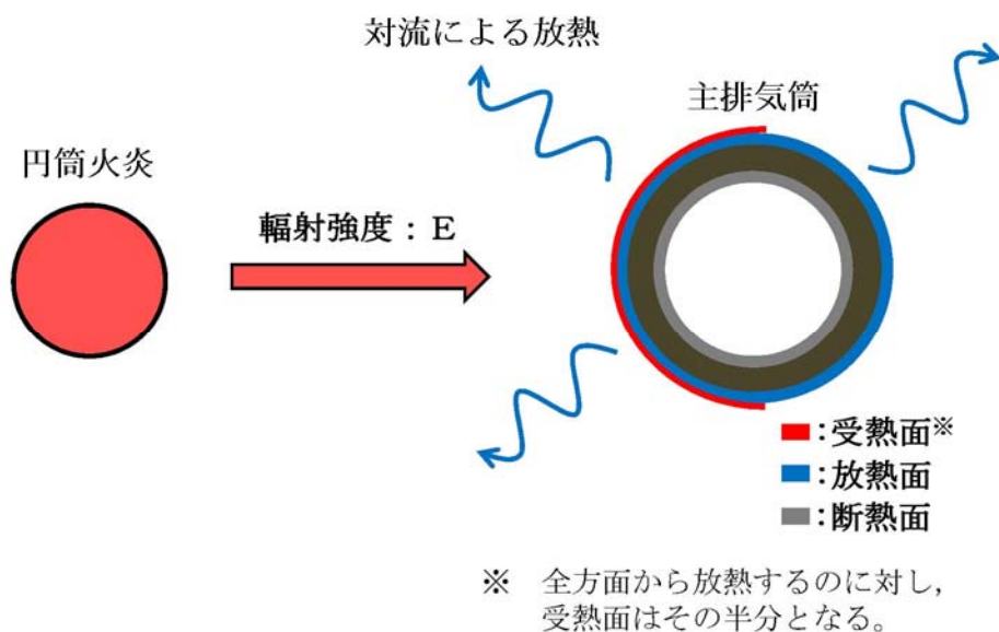
第 4. 1. 2. 4-2 図 主排気筒の評価概念図
