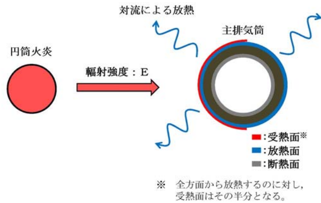
第 2. 2. 4-2 図 主排気筒の評価概念図
