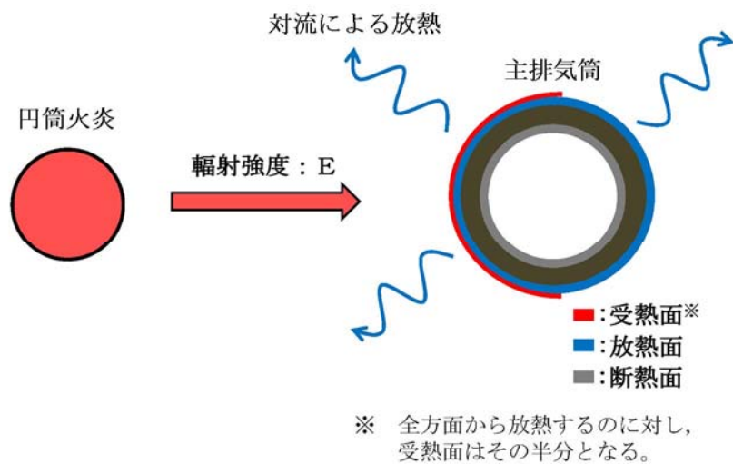
第 2.1.3.3-2 図 主排気筒の評価概念図
