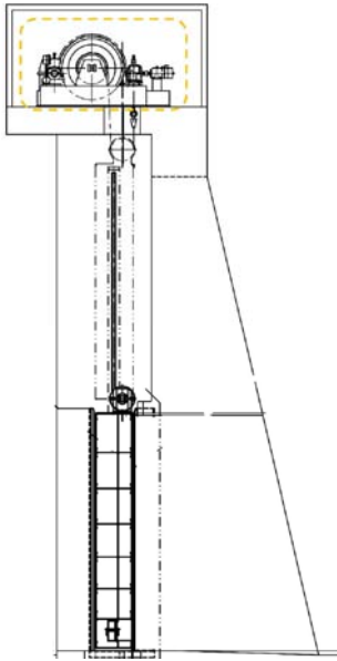
第 2.6-1 図 評価対象施設の外形図
