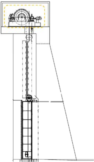
第 4.3.2.6-1 図 評価対象施設の外形図
