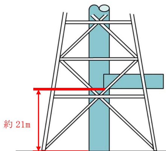
第 1 図 主排気筒下部の構造
