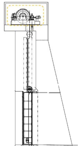
第 3. 2. 4-1 図 評価対象施設の外形図
