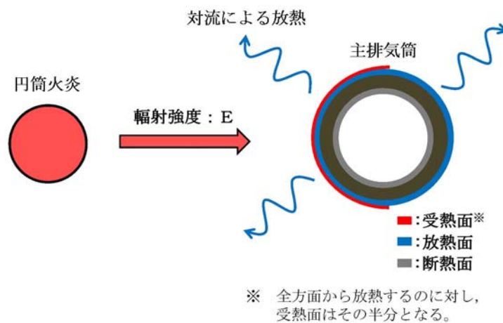
第 2.3-2 図 主排気筒の評価概念図
