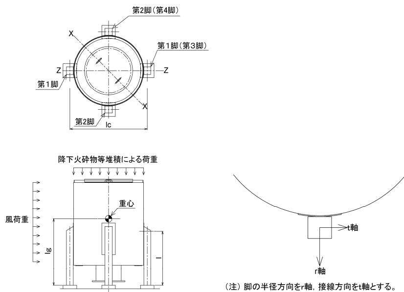
第 3 図 ディーゼル発電機吸気口 モデル図
