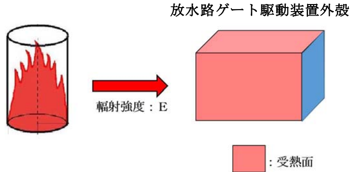
第 3. 2. 4-2 図 放水路ゲートの評価概念図
