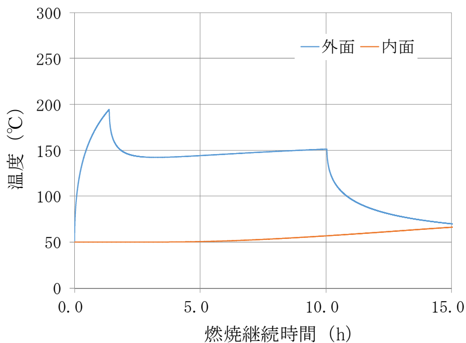
第 5.7-4 図 航空機火災と主要変圧器火災の重畳評価結果 (対象：タービン建屋)
