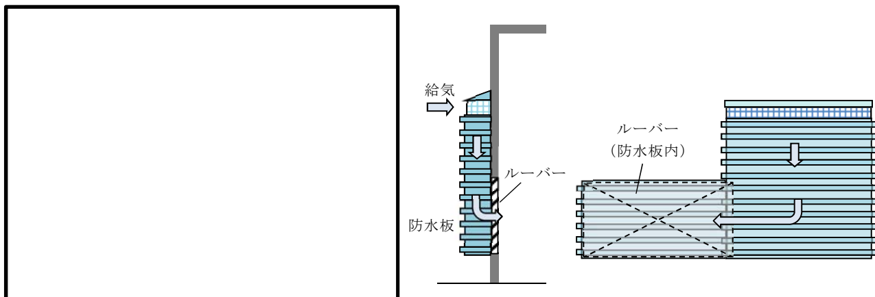
第2図 ディーゼル駆動消火ポンプ室給気口
