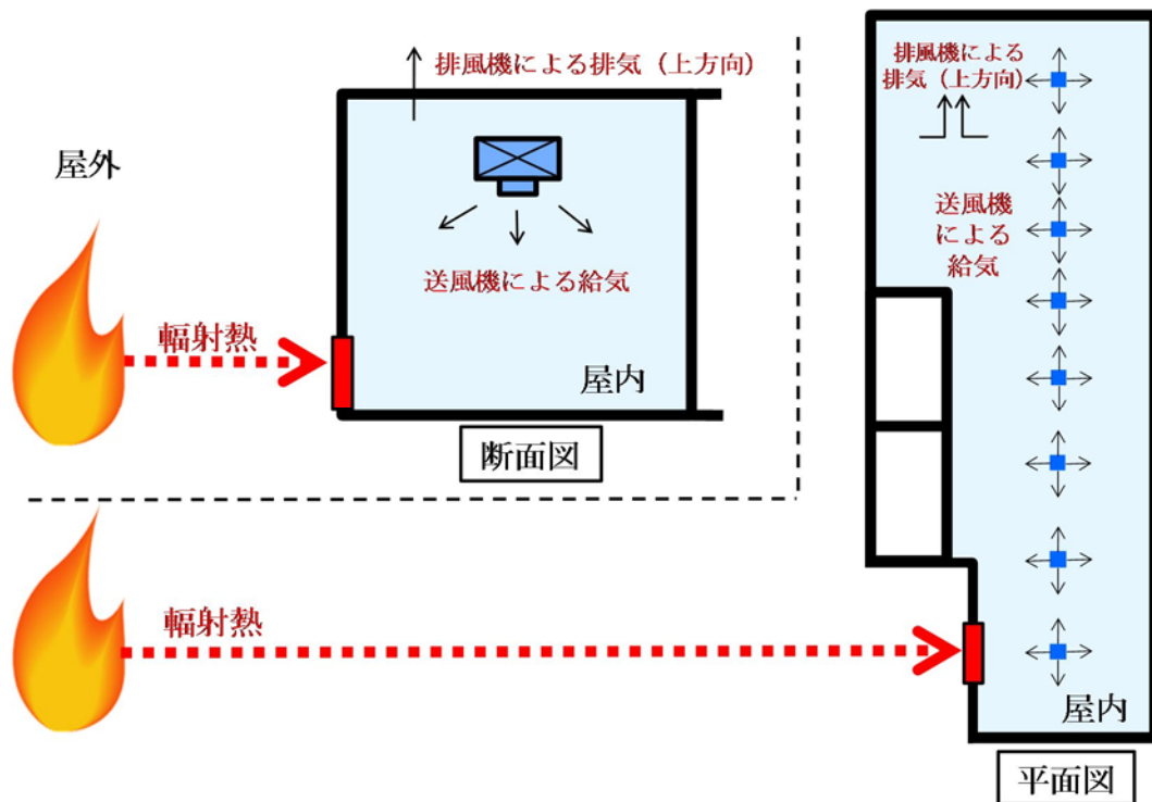
第 5.6.1.2-2 図 電気室内の給排気の概念図
