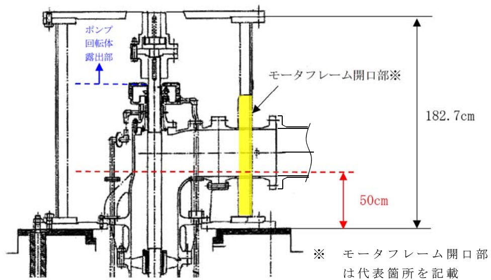
第 1 図 残留熱除去系海水系ポンプ
