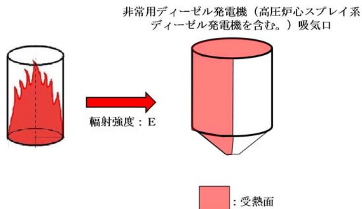
第2.2.3-2図 非常用ディーゼル発電機（高圧炉心スプレー系ディーゼル発電機を含む。）吸気口の評価概念図
