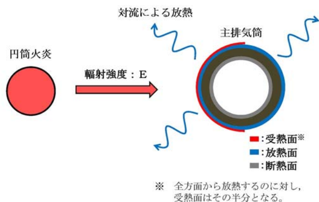
第 4.3.2.3-2 図 主排気筒の評価概念図
