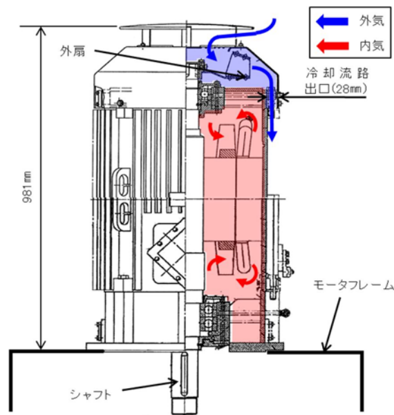
第 8 図 非常用ディーゼル発電機（高圧炉心スプレイ系ディーゼル発電機を含む。）用海水ポンプ電動機の冷却方式
