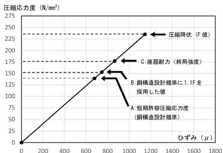
第 2 図 F 値 \times 1.1 を適用し算定した強度と座屈耐力の比較例
