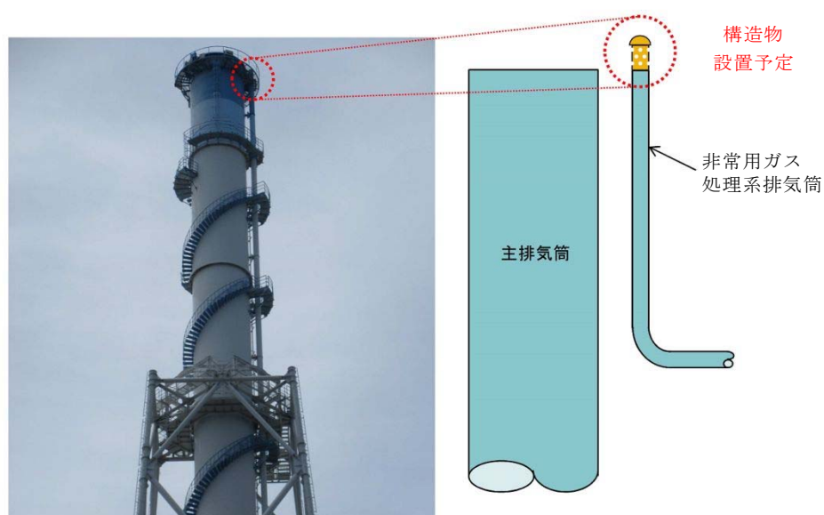
第 2 図 非常用ガス処理系排気筒 概略図
