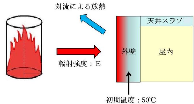
第 2.1.3.3-1 図 建屋外壁の評価概念図
