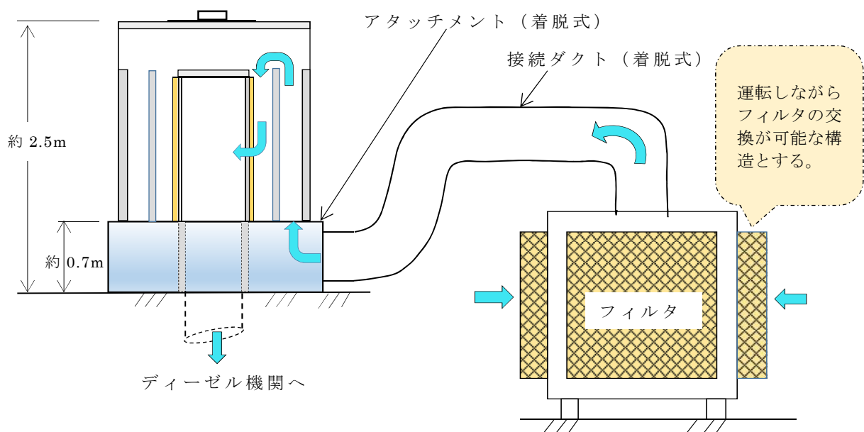
非常用ディーゼル発電機（高圧炉心スプレー系ディーゼル発電機を含む。）吸気フィルタ（既設）へ着脱式フィルタを取付け
