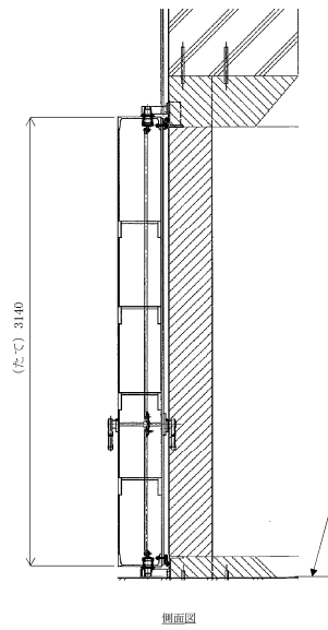
側面図
