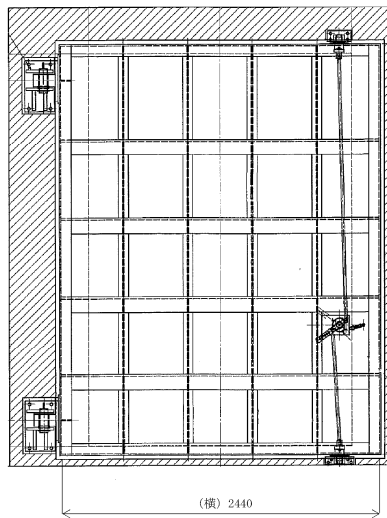
正面図
