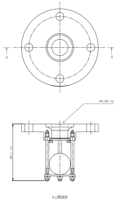
図 3-20 緊急用海水ポンプグランド dren 排出口逆止弁の構造図
