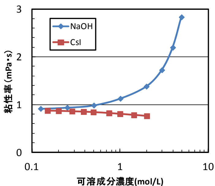
第 1 図 NaOH と CsI が水に溶解した場合の粘性率の変化 ( 25^\circ\text{C} )
