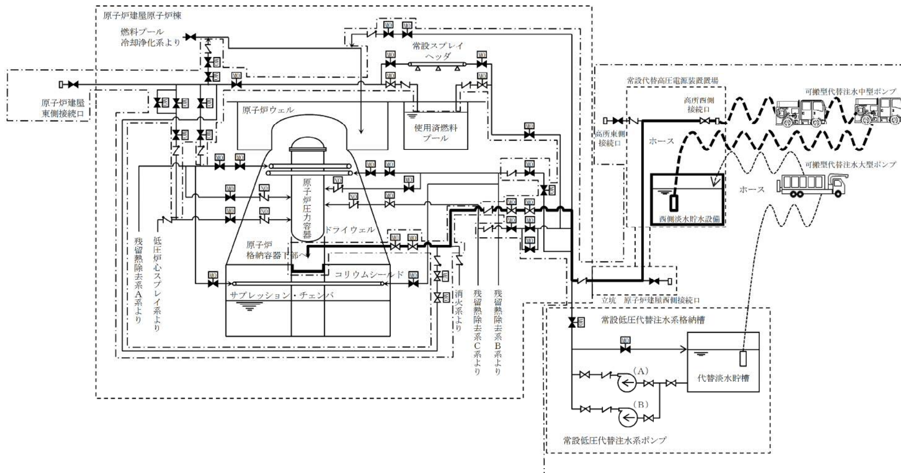
第1図 格納容器下部注水系（可搬型）によるペデスタル（ドライウエル部）への注水
