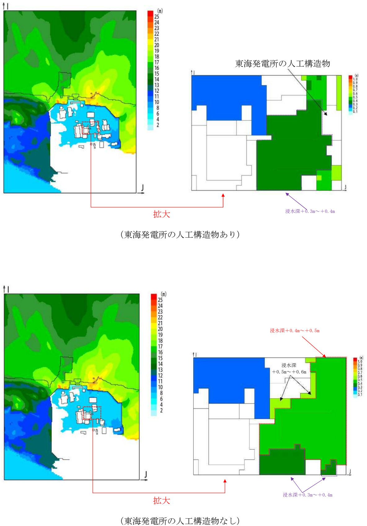
図 4-3 防潮堤内側の入力津波設定における浸水深の東海発電所の人工構造物の影響確認
