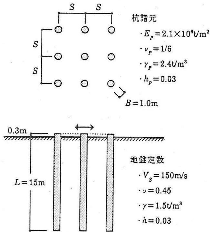
図2.1.2-3 解析モデル及び解析諸元
