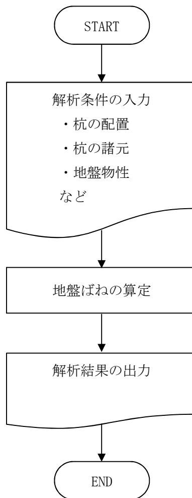
図2.1.2-2 解析フローチャート
