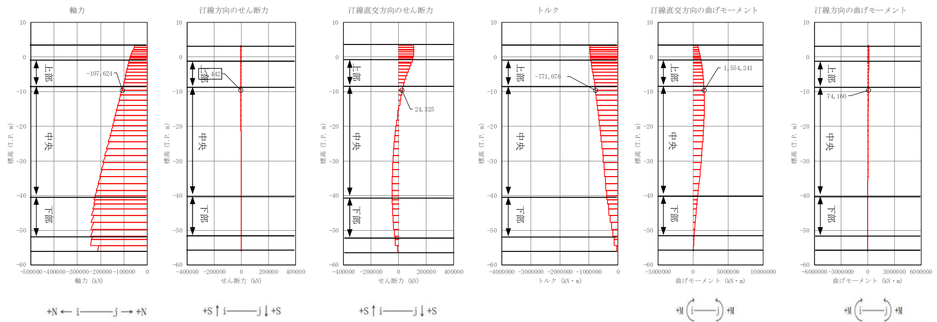
図 4.1-5 (3) 地中連続壁基礎においてせん断力照査結果が最も厳しい断面力 ①-①断面 (津波時：基準津波，北-中央，地盤バネ 1)
