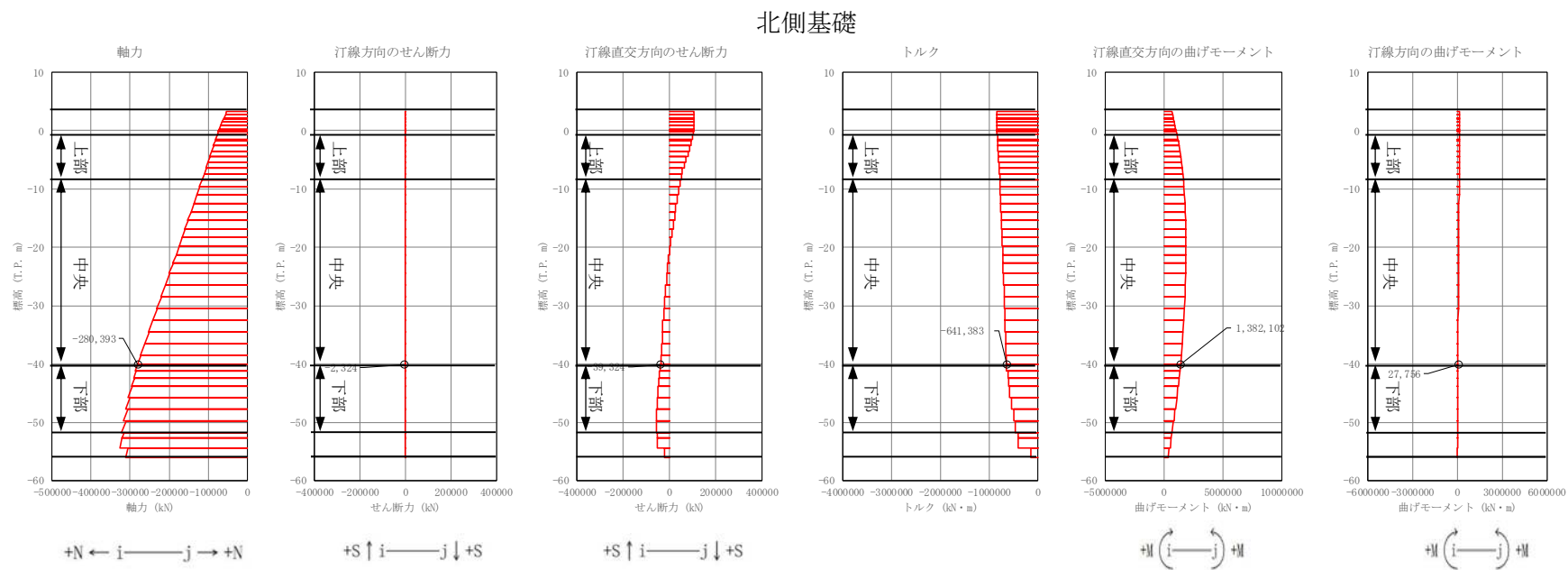
図 4.1-4 (4) 地中連続壁基礎において鉄筋の曲げ軸力照査結果が最も厳しい断面力
