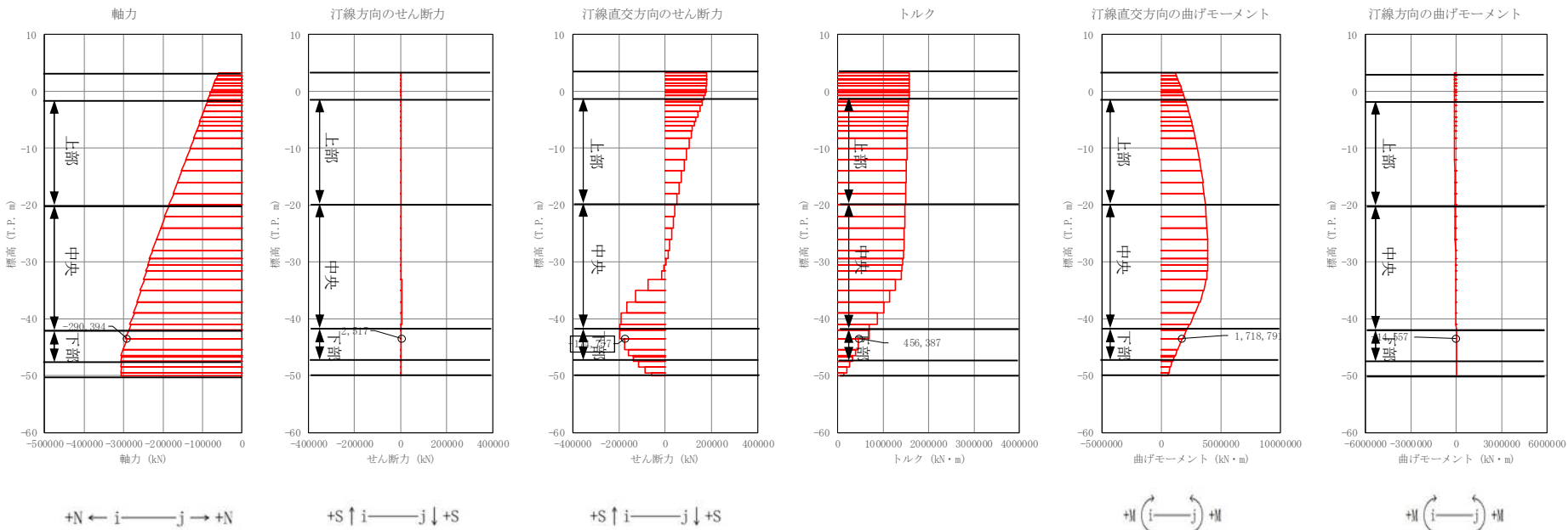
図 4.1-5 (16) 地中連続壁基礎においてせん断力照査結果が最も厳しい断面力 ③-③断面 (津波時: T.P. +24 m 津波, 南-下部, 地盤バネ 2)
