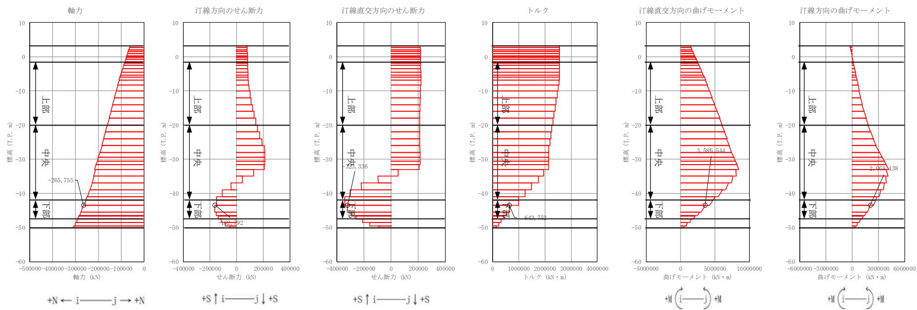
図 4.2-10 (16) 地中連続壁基礎においてせん断力照査結果が最も厳しい断面力
