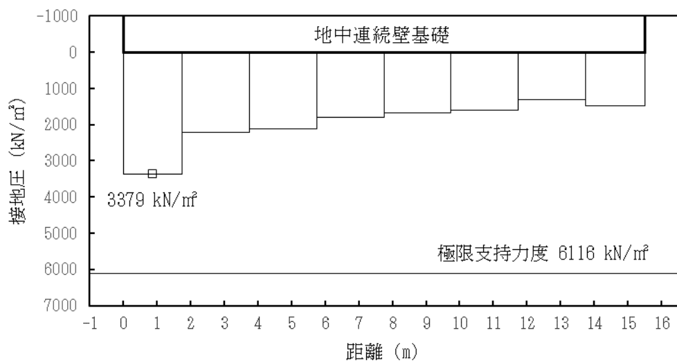
図 4.2-22 (24) 接地圧分布図 (②-②断面) (T. P. +24 m 津波時) (検討ケース⑥: 地盤物性のばらつきを考慮 (+1 \sigma ) して 非液状化の条件を仮定した解析ケース)
