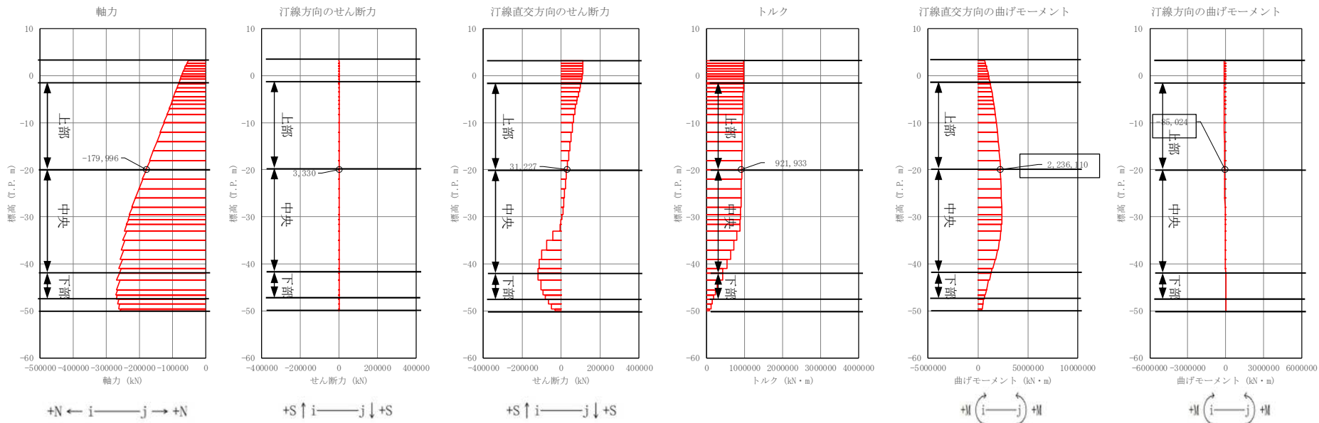
図 4.1-3 (1) 地中連続壁基礎においてコンクリートの曲げ軸力照査結果が最も厳しい断面力 ①-①断面, ③-③断面, (津波時: 基準津波, 上部, 地盤バネ 2)
