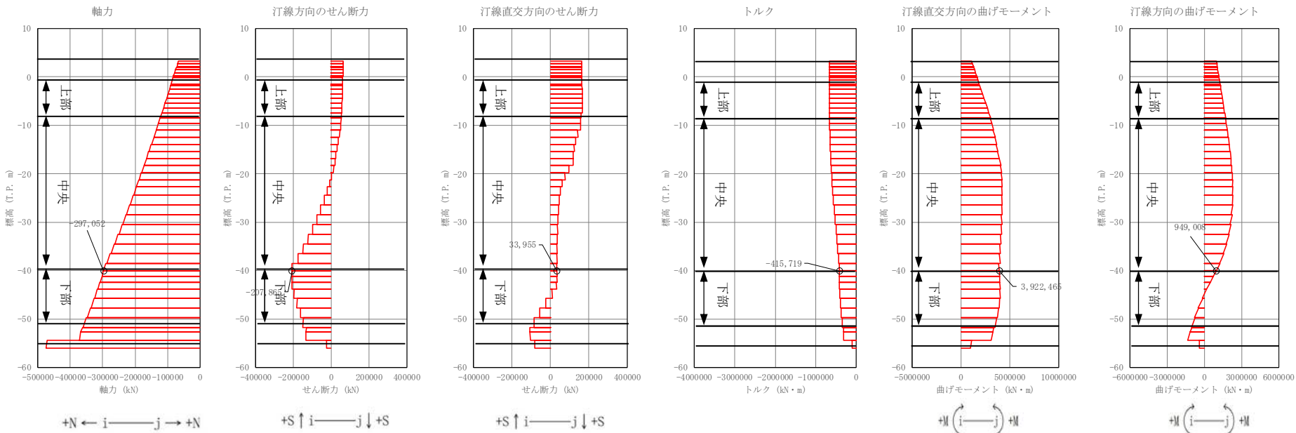
図 4.2-10 (11) 地中連続壁基礎においてせん断力照査結果が最も厳しい断面力 ①-①断面（重疊時：T.P. +24 m 津波，北-中央，地盤バネ 5）
