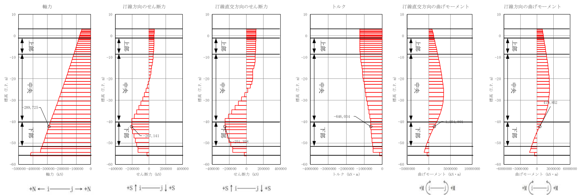
図 4.2-10 (8) 地中連続壁基礎においてせん断力照査結果が最も厳しい断面力 ②-②断面 (重疊時：基準津波，北-下部，地盤バネ 5)
