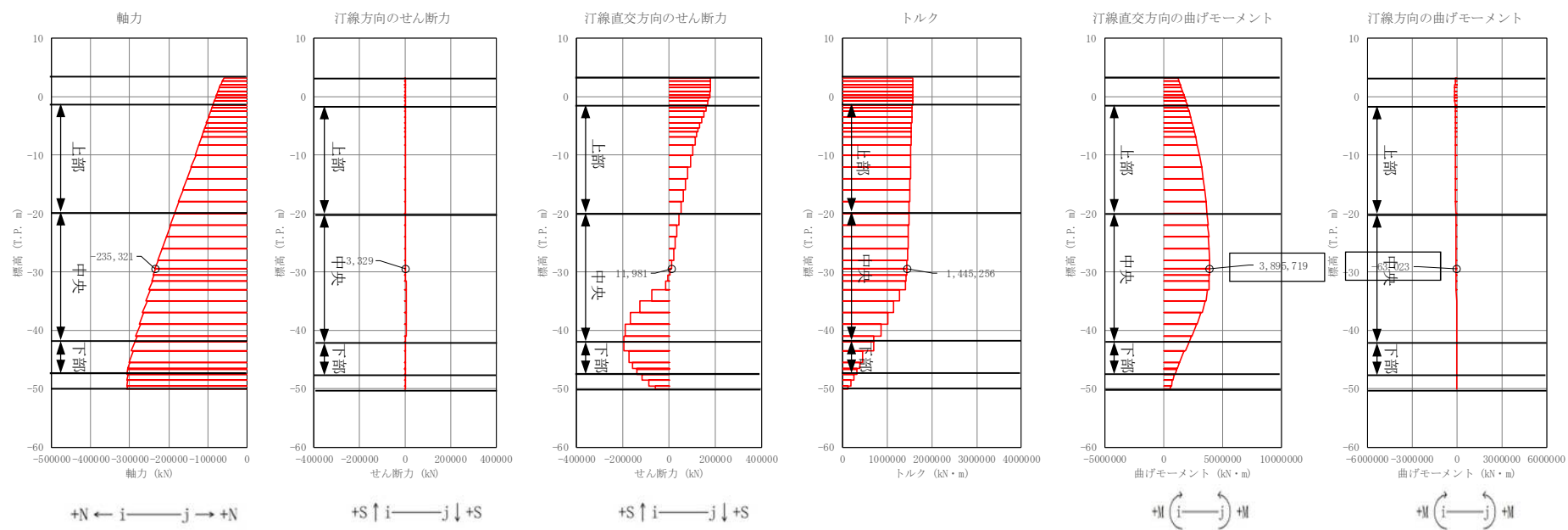
図 4.1-3 (7) 地中連続壁基礎においてコンクリートの曲げ軸力照査結果が最も厳しい断面力 ①-①断面, ③-③断面 (津波時 : T.P. +24 m 津波, 南-中央, 地盤バネ 2)
