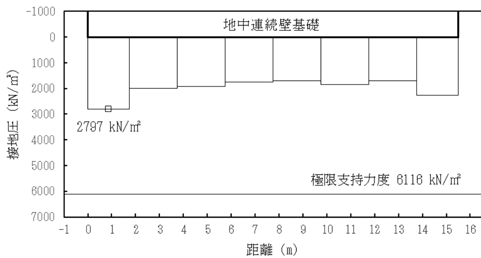
図 4.2-22 (14) 接地圧分布図 (②-②断面) (基準津波時) (検討ケース②: 地盤物性のばらつきを考慮 (+1σ) した解析ケース)
