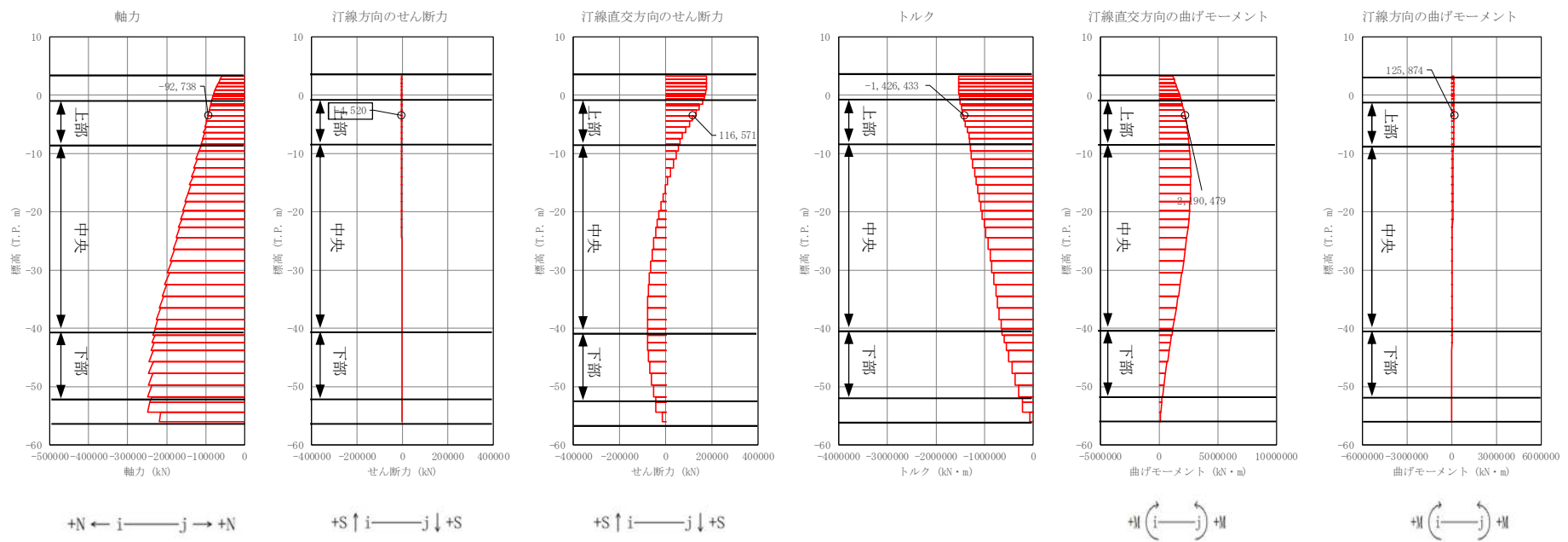
図 4.1-5 (9) 地中連続壁基礎においてせん断力照査結果が最も厳しい断面力 ①-①断面 (津波時 : T.P. +24 m 津波, 北-上部, 地盤バネ 1)
