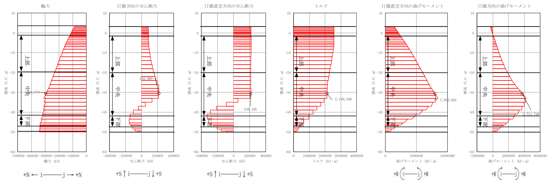
図 4.2-10 (13) 地中連続壁基礎においてせん断力照査結果が最も厳しい断面力
