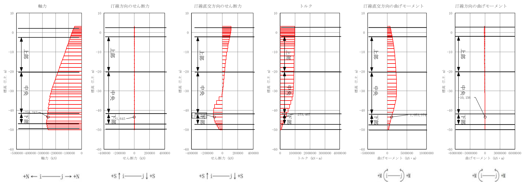
図 4. 1-5 (7) 地中連続壁基礎においてせん断力照査結果が最も厳しい断面力
