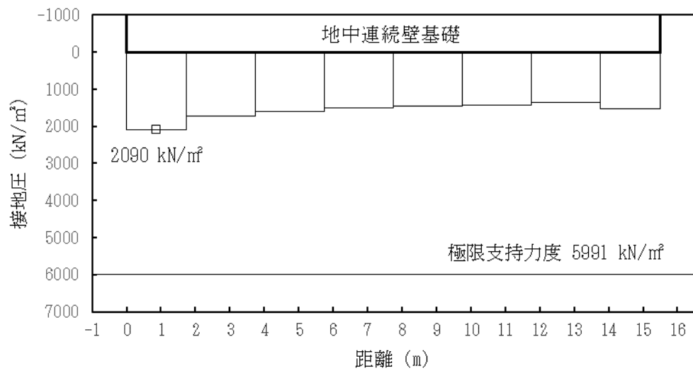
図 4.2-22 (4) 接地圧分布図 (③-③断面) (基準津波時) (検討ケース④：敷地に存在しない豊浦標準砂の液状化強度特性により 地盤を強制的に液状化させることを仮定した解析ケース)
