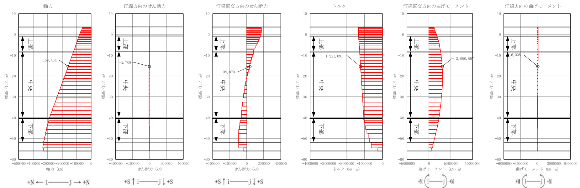
図 4.1-4 (6) 地中連続壁基礎において鉄筋の曲げ軸力照査結果が最も厳しい断面力 ①-①断面, ②-②断面 (津波時: T.P. +24 m 津波, 北-中央, 地盤バネ 2)
