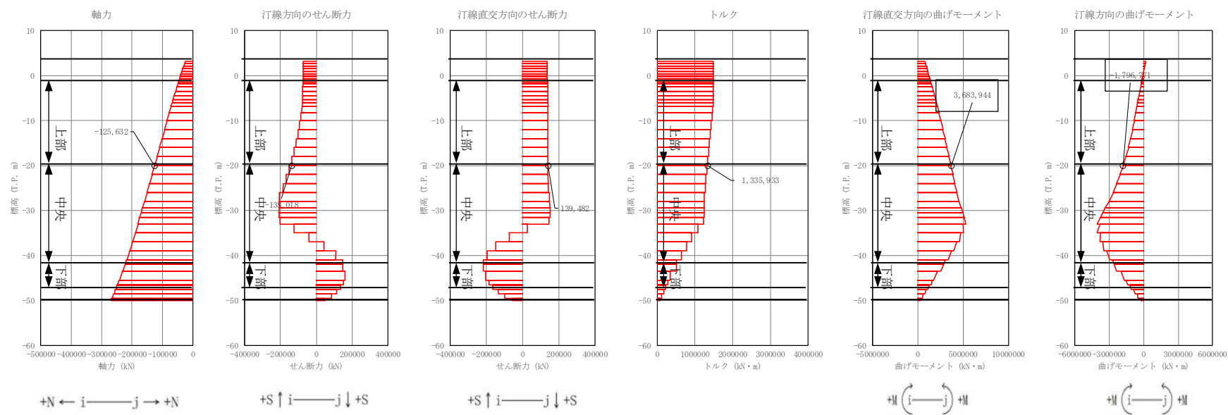
図 4.2-9 (1) 地中連続壁基礎において鉄筋の曲げ軸力照査結果が最も厳しい断面力 ①-①断面, ③-③断面 (重疊時: 基準津波, 上部, 地盤バネ 4)
