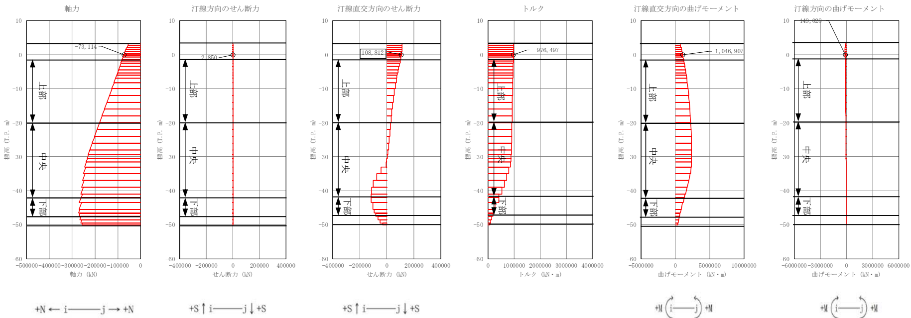
図 4.1-5 (5) 地中連続壁基礎においてせん断力照査結果が最も厳しい断面力 ③-③断面 (津波時：基準津波，南-上部，地盤バネ 2)
