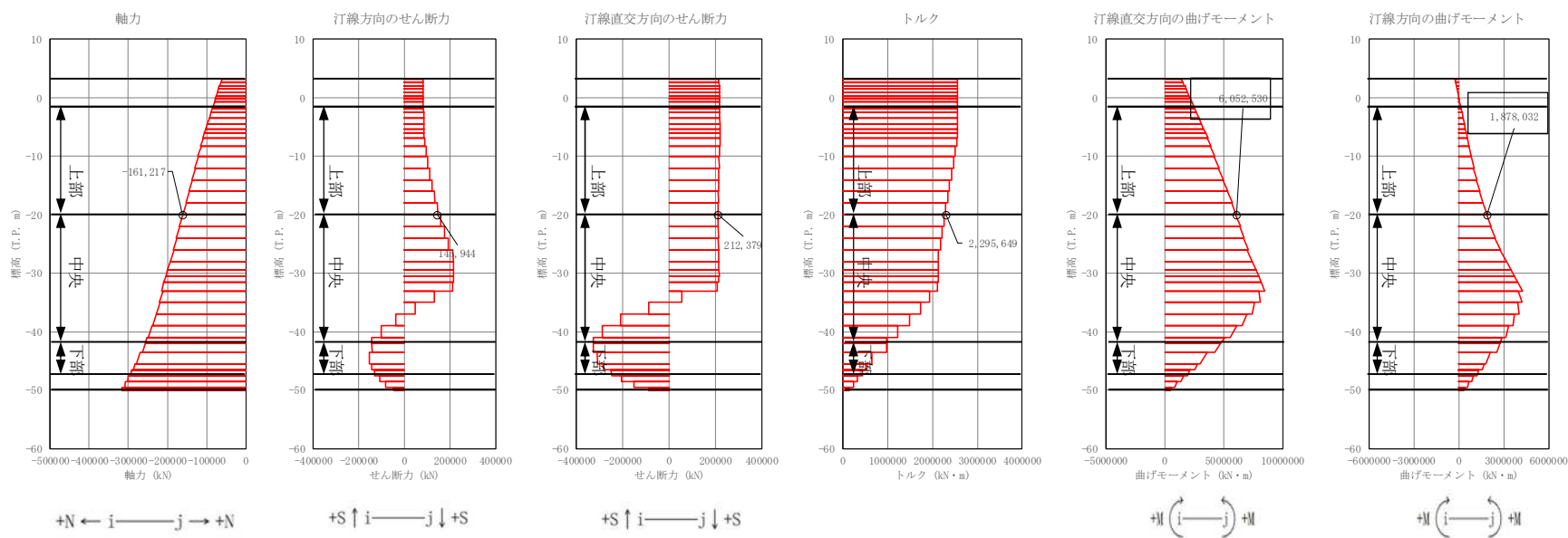
図 4.2-8 (5) 地中連続壁基礎においてコンクリートの曲げ軸力照査結果が最も厳しい断面力
