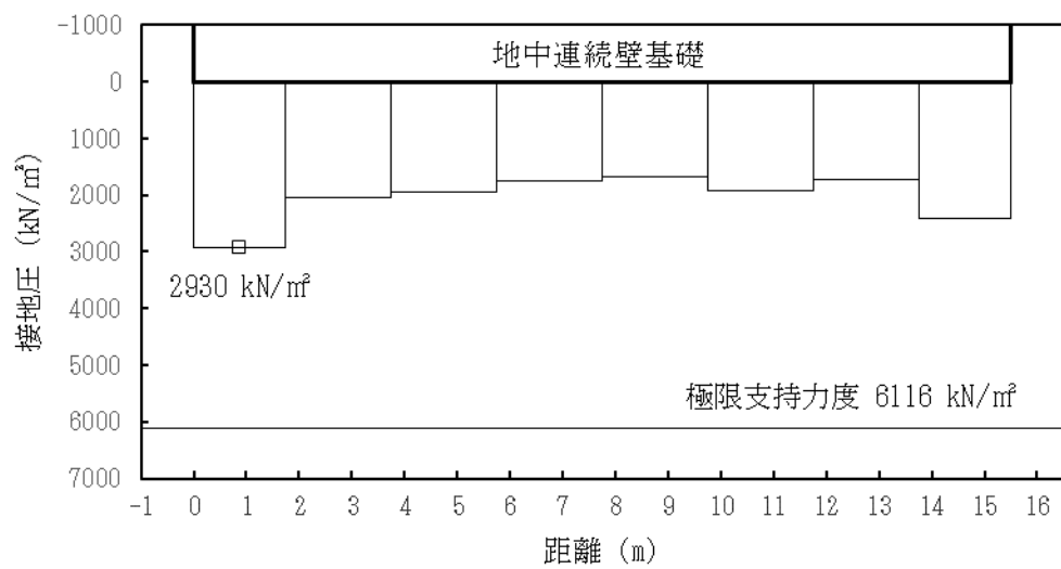
図 4.2-22 (16) 接地圧分布図 (②-②断面) (基準津波時) (検討ケース④: 敷地に存在しない豊浦標準砂の液状化強度特性により 地盤を強制的に液状化させることを仮定した解析ケース)
