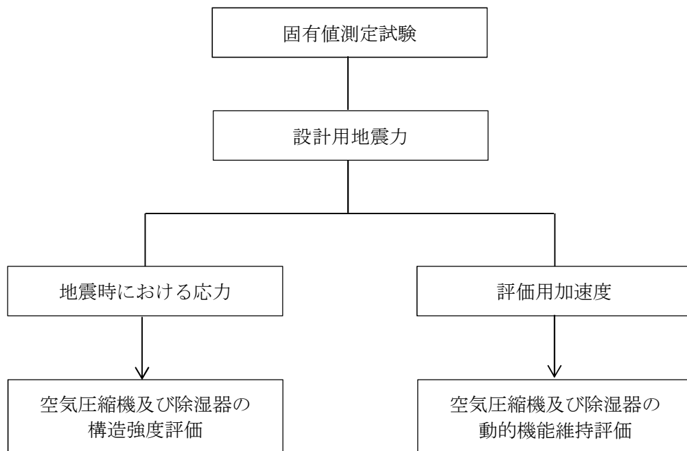
図 1-1 使用済燃料プール監視カメラ用空冷装置（空気圧縮機及び除湿器）の耐震評価フロー
