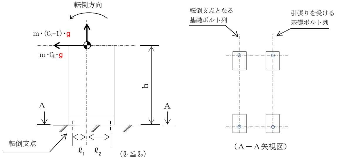
図 1-2 使用済燃料プール監視カメラ用空冷装置（空気圧縮機及び除湿器） 計算モデル（短辺方向転倒）
