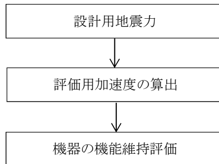
図 2-1 使用済燃料プール監視カメラ用空冷装置(冷却器)の耐震評価フロー
