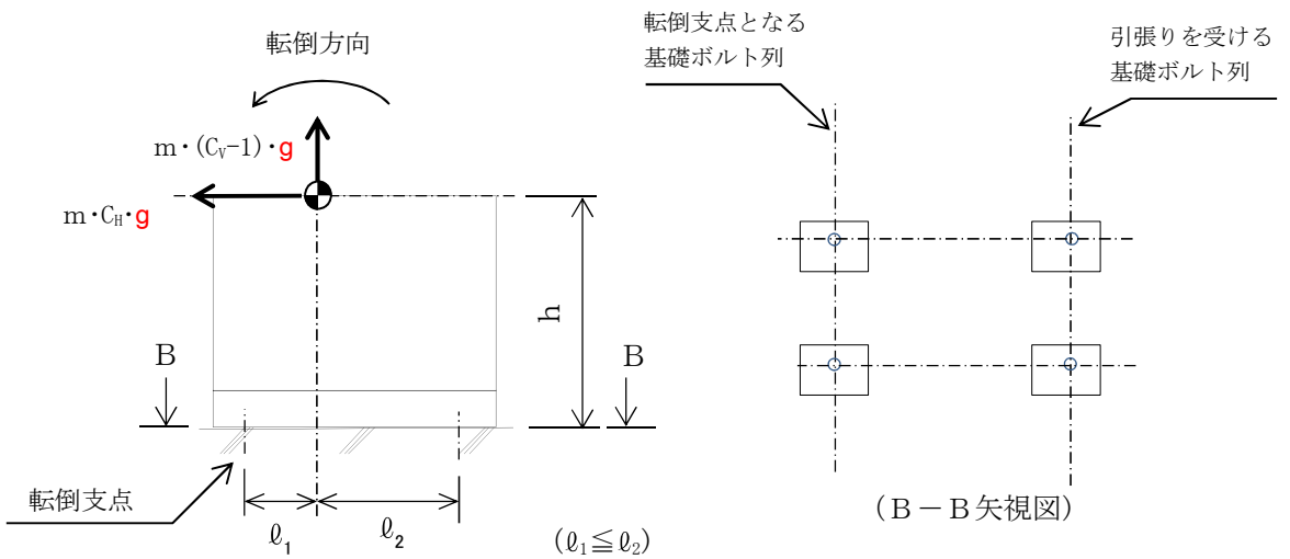
図 1-3 使用済燃料プール監視カメラ用空冷装置（空気圧縮機及び除湿器） 計算モデル（長辺方向転倒）
