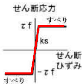
図7 杭軸方向ばねの力学特性
