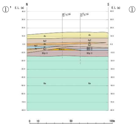
①—①' 断面
