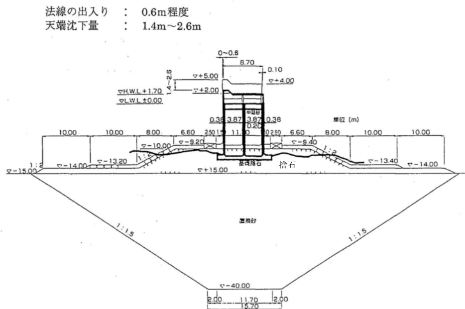
図2 検討対象断面（神戸港第七防波堤）*
