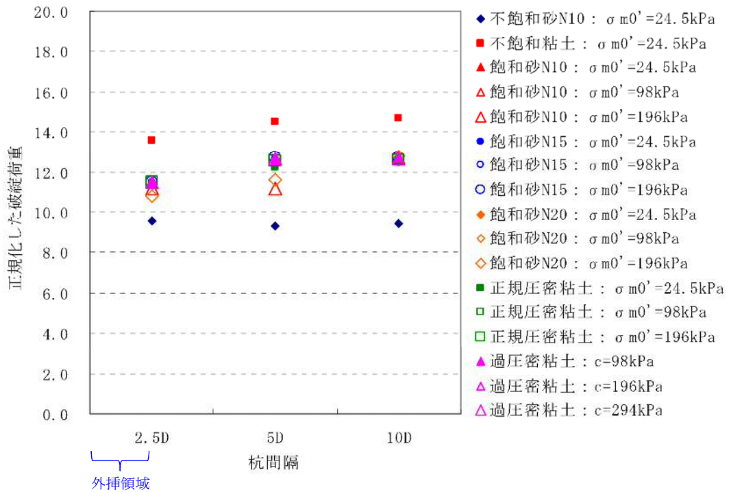
図 4-11-9 単調載荷時の（破綻荷重／初期せん断強度 \tau_{m0} ）の分布
