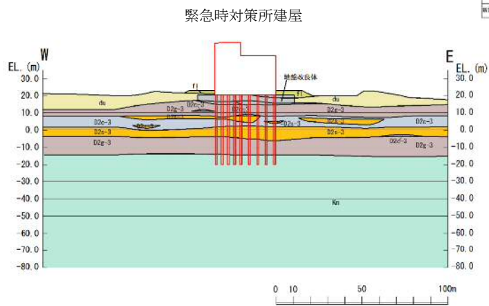
(4) 緊急時対策所周辺断面 (D-D 断面)
