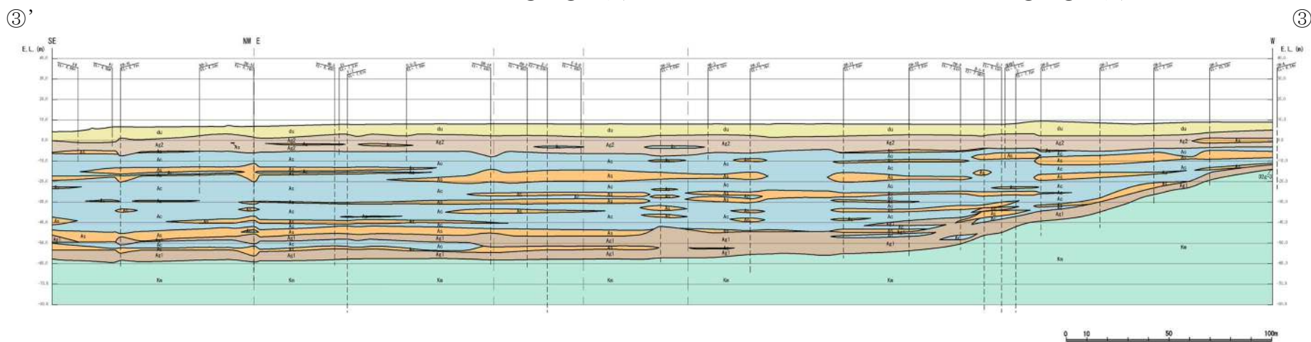
③—③' 断面
