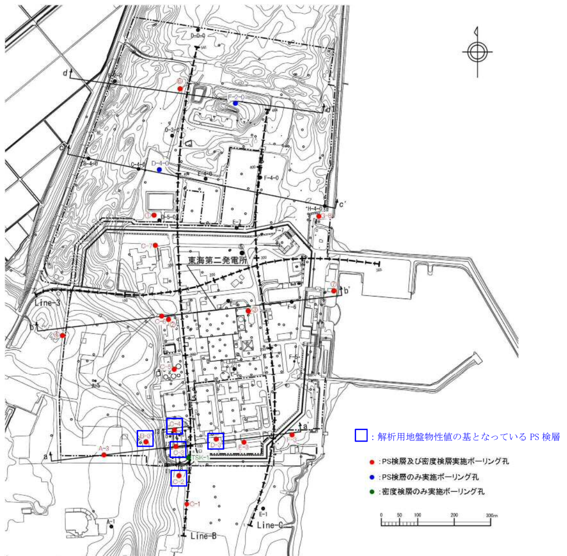
図 6.3-5 PS 検層実施位置図（敷地の地質・地質構造検討用）
