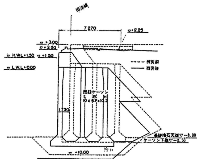
図3 検討対象断面（神戸港第七防波堤）*
