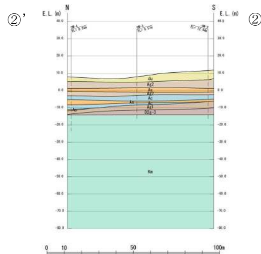
②—②' 断面
