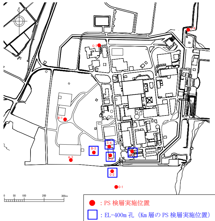
図 6.2-1 PS 検層実施位置図
