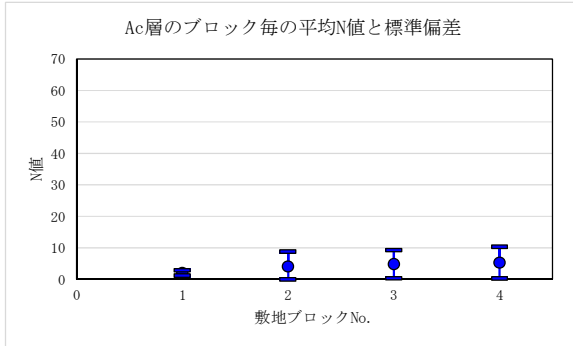
(ブロック区分とN値の採取位置) 図 6.3-2 (4) 各ブロックにおけるN値の比較結果 (Ac層)
