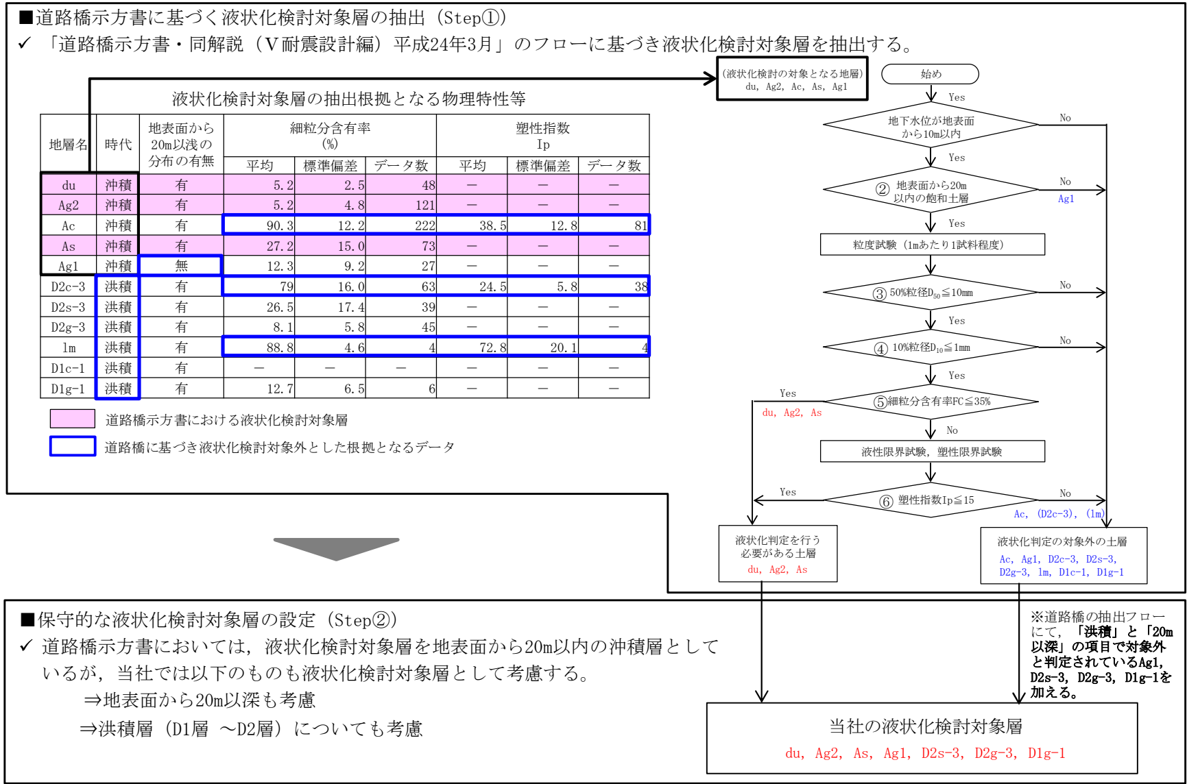
図 4.2-3 液状化検討対象層抽出方針
