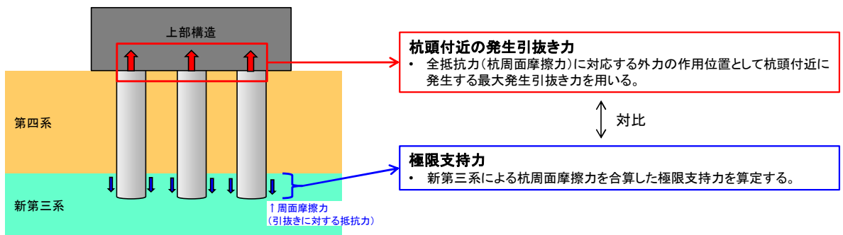
図3 引抜き力に対する杭基礎の支持力評価
