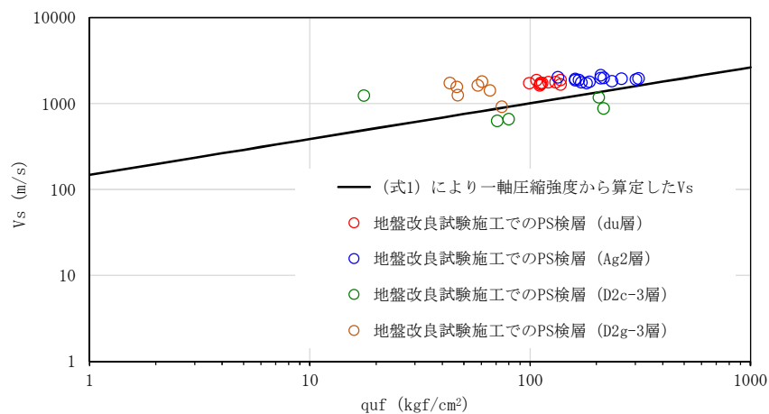
図 2 (式 1) と PS 検層結果の比較
