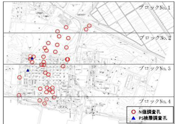
(ブロック区分とN値の採取位置) 図 6.3-2 (8) 各ブロックにおけるN値の比較結果 (D2g-3層)
