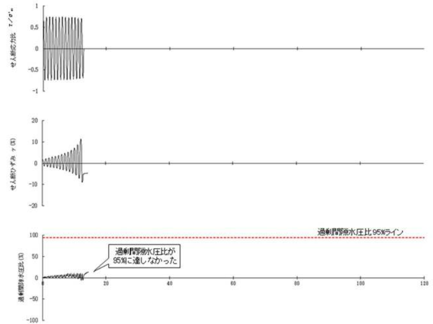
液状化強度試験における各計測値
