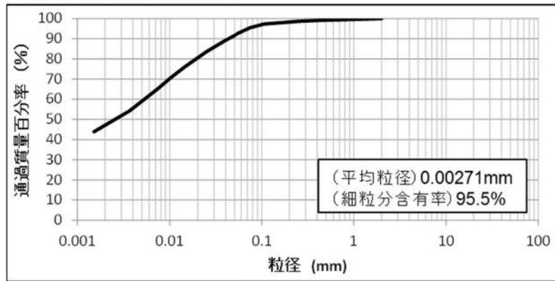
試料の粒径加積曲線
