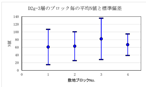
(ブロック区分とN値の採取位置) 図 6.3-2 (8) 各ブロックにおけるN値の比較結果 (D2g-3層)
