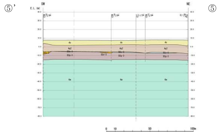
⑤—⑤' 断面
