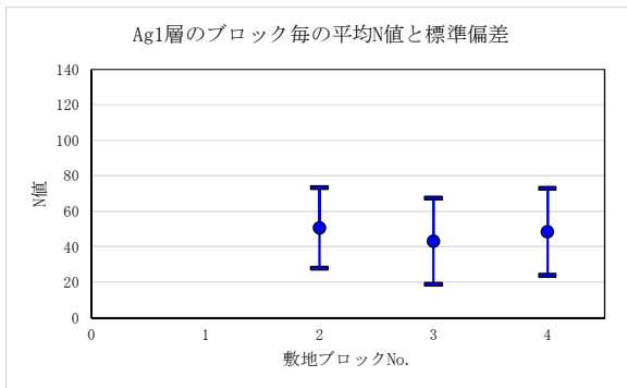
(ブロック区分とN値の採取位置) 図 6.3-2 (5) 各ブロックにおけるN値の比較結果 (Ag1層)
