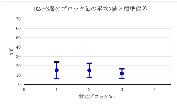
(ブロック区分とN値の採取位置) 図 6.3-2 (7) 各ブロックにおけるN値の比較結果 (D2c-3層)
