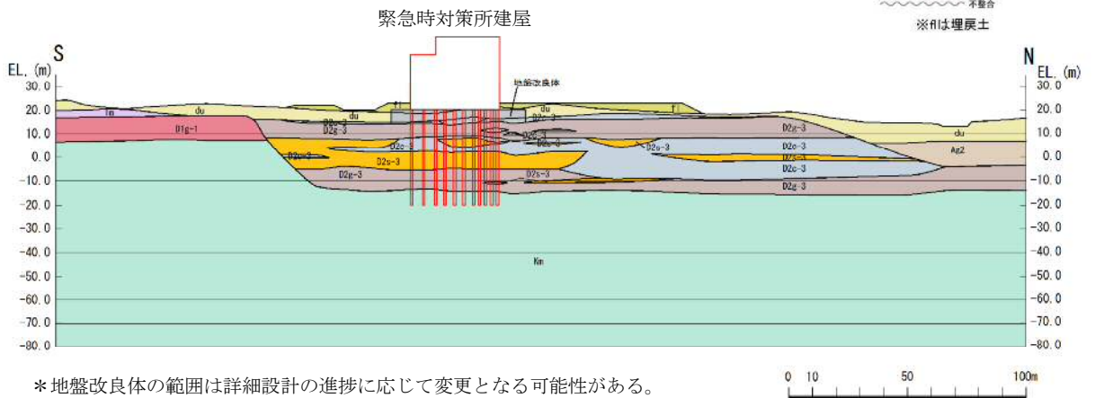
(3) 緊急時対策所周辺断面 (C-C 断面)
