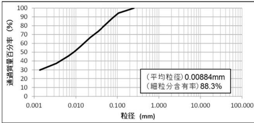
試料の粒径加積曲線
