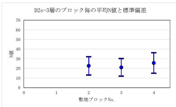
(ブロック区分とN値の採取位置) 図 6.3-2 (6) 各ブロックにおけるN値の比較結果 (D2s-3層)
