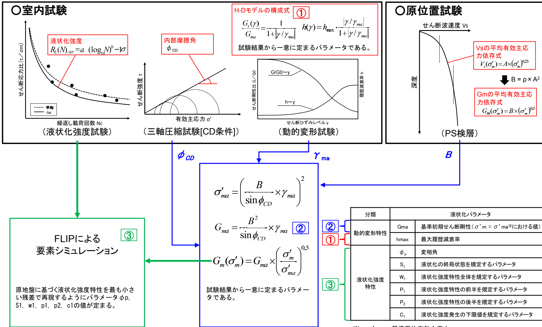
図 4.2-9 液状化パラメータ設定の流れ
