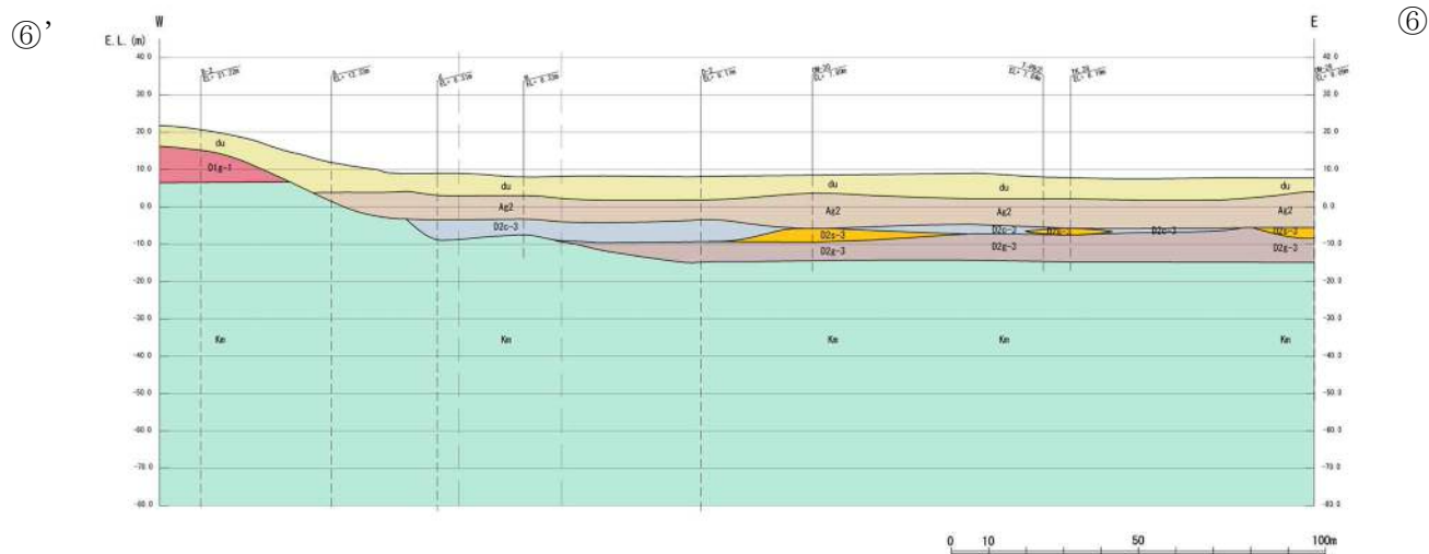
⑥—⑥' 断面
