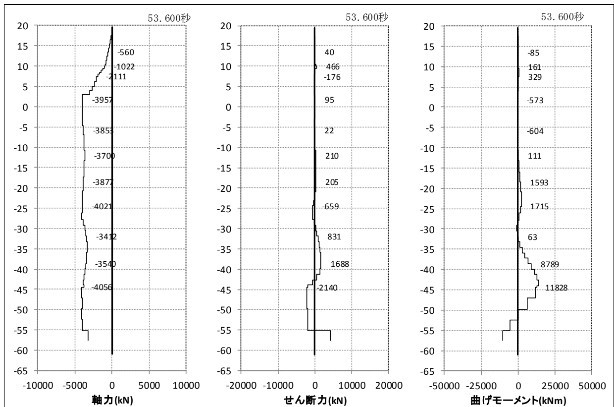
ケース 1 (杭-地盤相互作用ばね)
