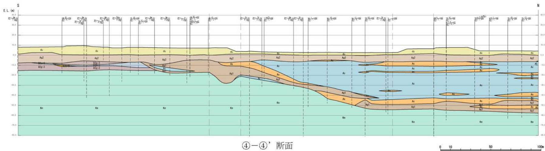
图 3.1-3 (5) 地質断面图 (5/6)
