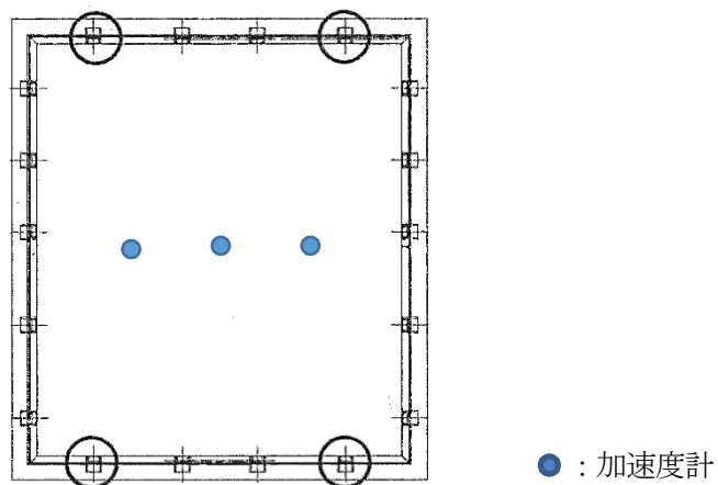
第5図 計測機器取付位置図
