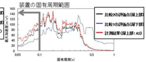
図 3-2 扉開 上部測定結果 (試験 No. 9)
