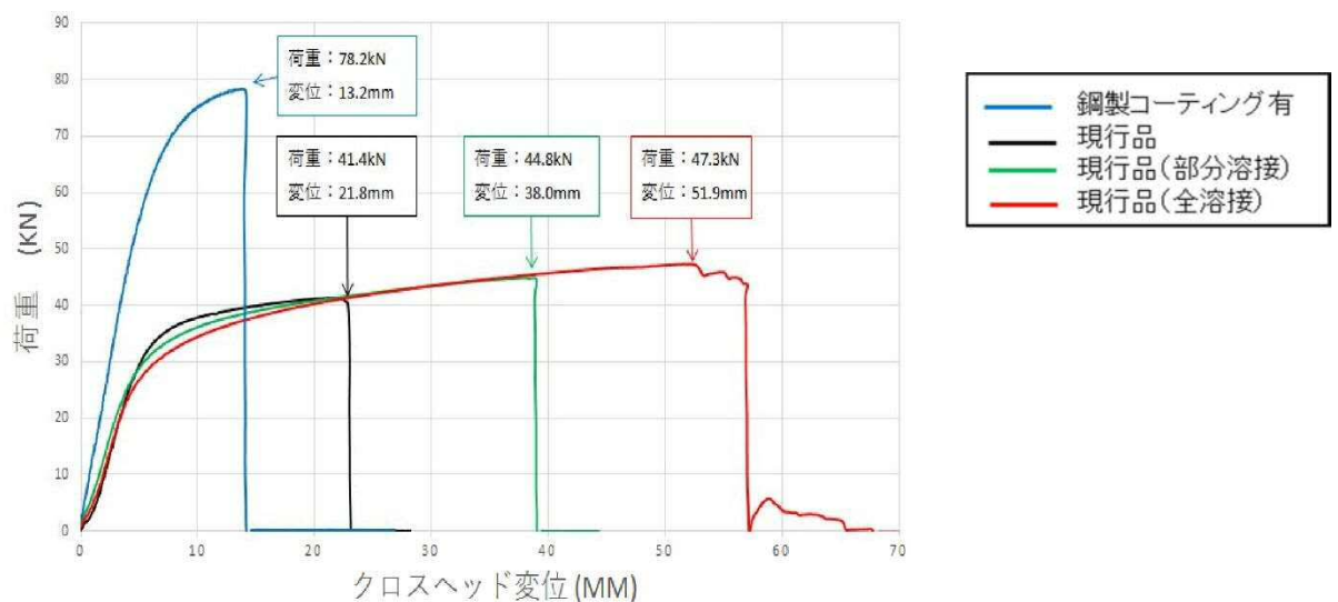
図 4-13 チェーンの引張り試験結果（荷重－変位線図）
