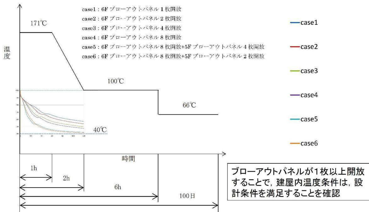
図 3-2 主蒸気管破断時の原子炉棟内温度の解析結果
