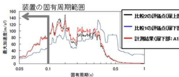
図 3-1 扉開 下部測定結果 (試験 No. 9)
