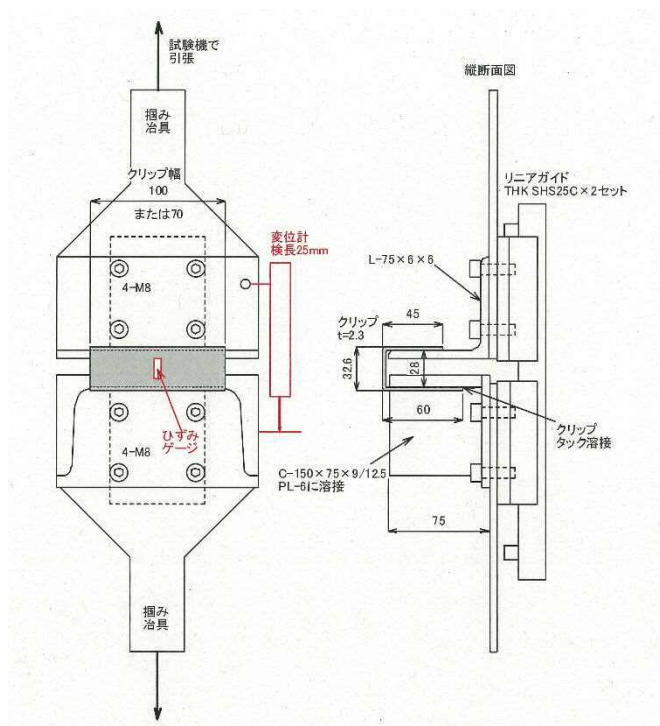
図 4-1 クリップの引張試験概要図
