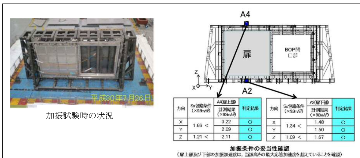
図 2-1 門がない状態での加振試験時の状況
