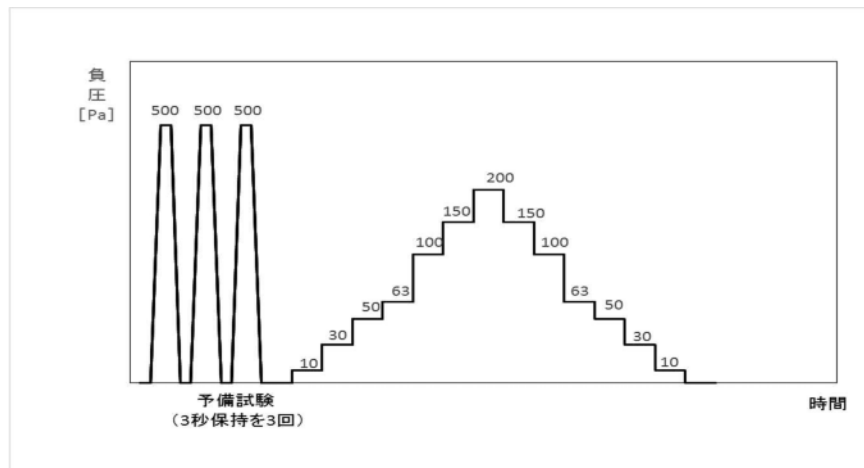
図 5-3 負圧試験線図
