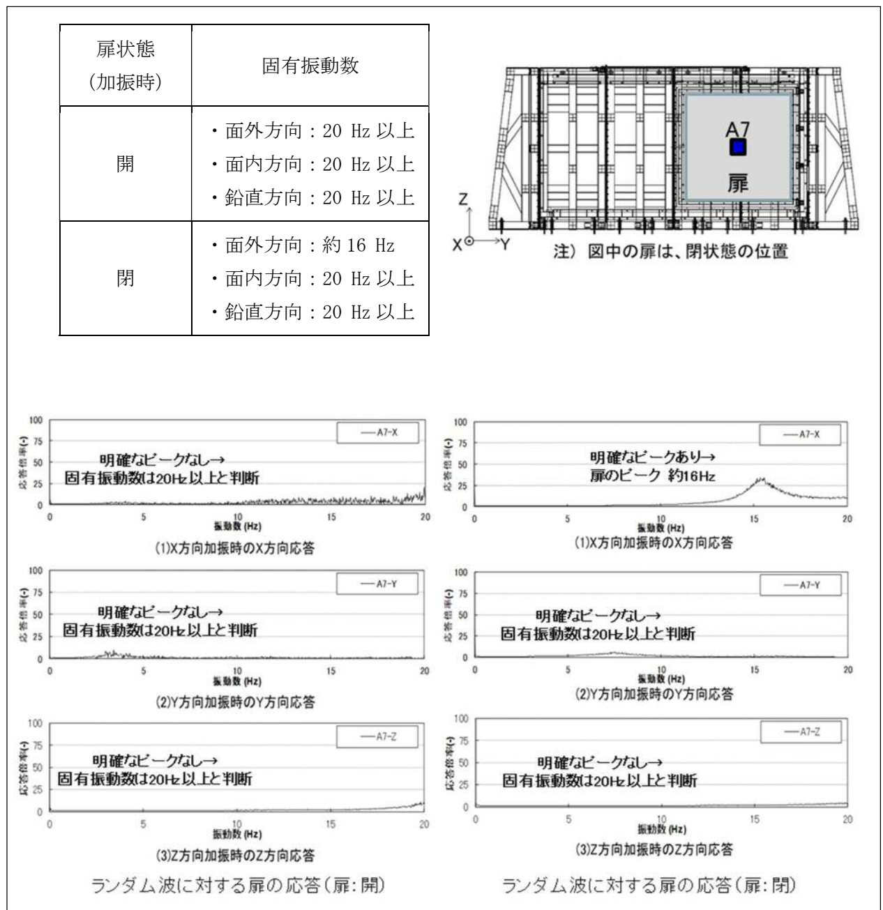
図 2-1 固有振動数
