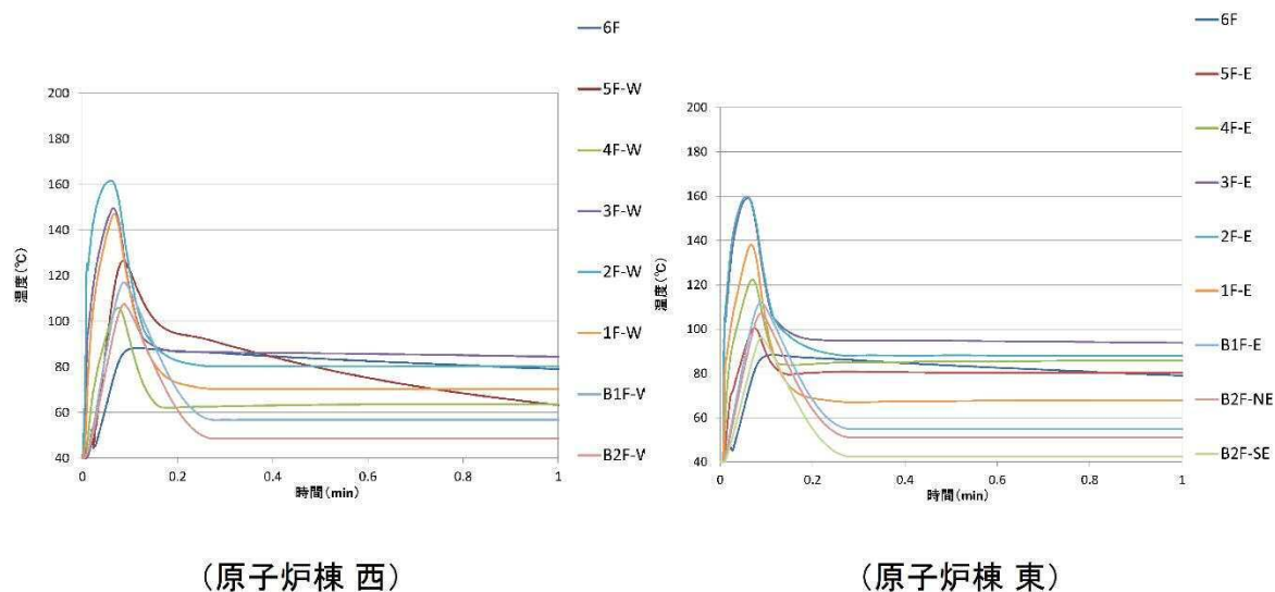
図 3-5 対策後の温度状況比較 (最高温度)
