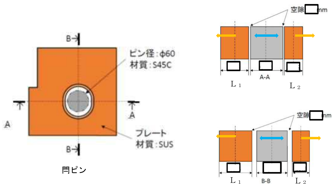
図3-1 門ピン及び門受フレーム
