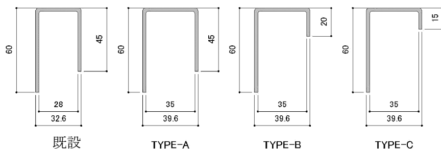
試験用クリップ形状
