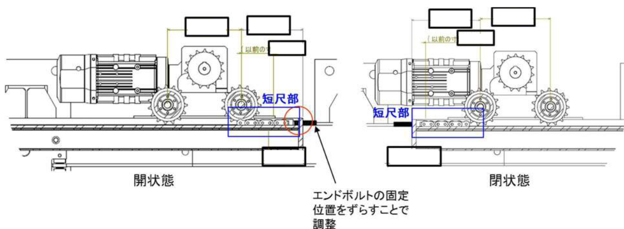
図 2-10 チェーンの短尺部
