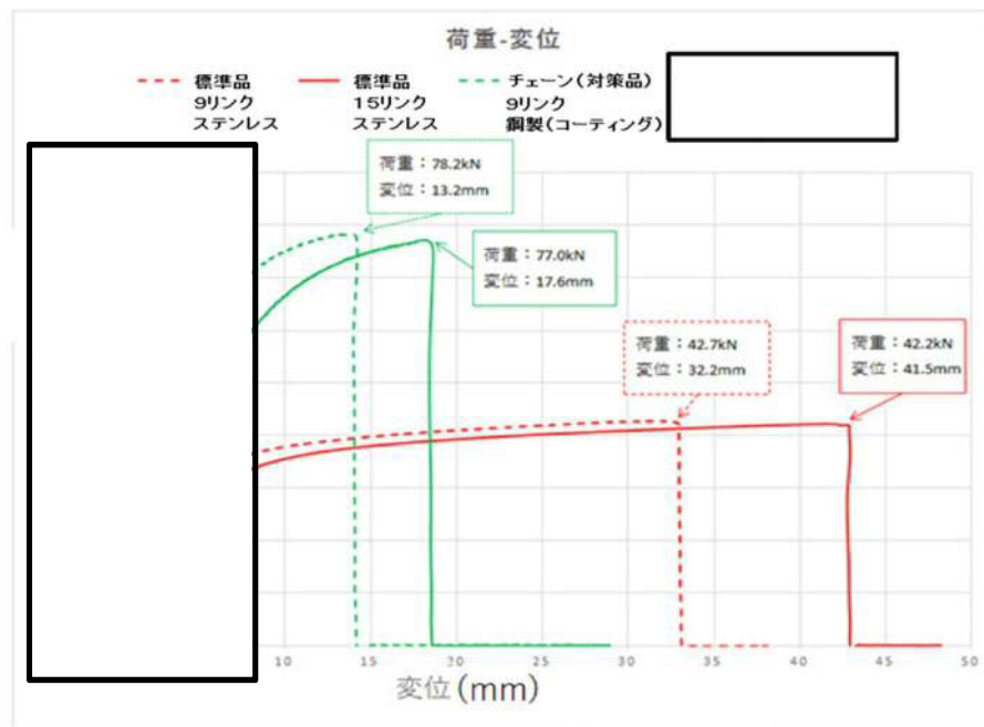
図 4-2 変位と荷重曲線
