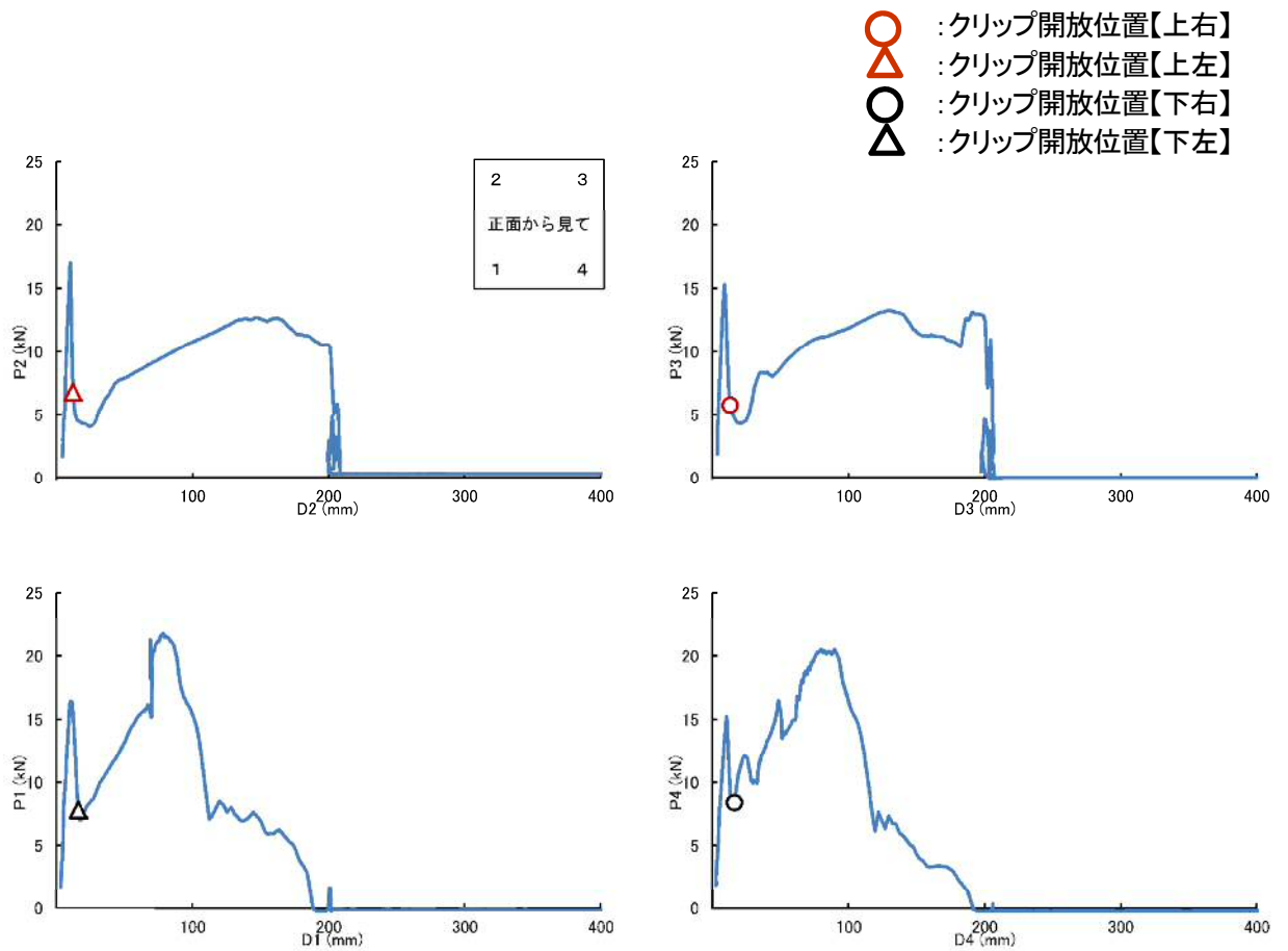
図 2-2(2) 各油圧ジャッキの荷重と変位測定結果 (2 回目)
