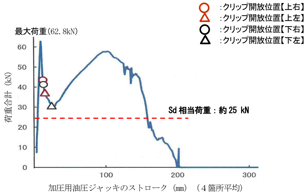
図 2-2(1) 油圧ジャッキの荷重合計と変位図
