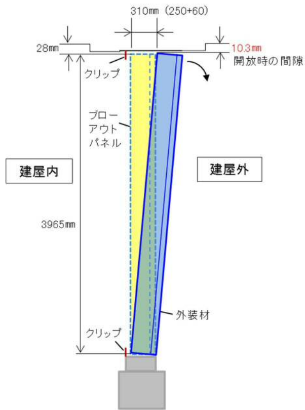
縦断面図
