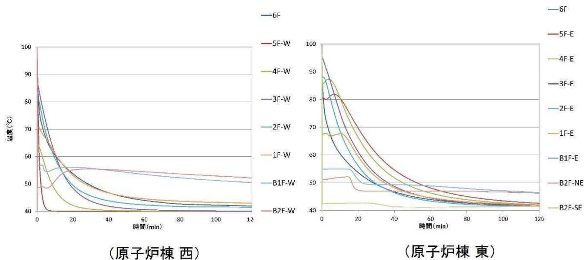
図 3-4 対策後の温度状況比較
