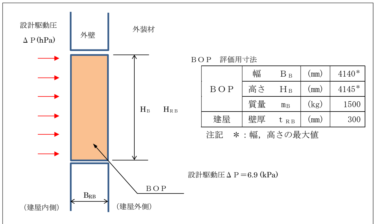
図 2-1 概略図及び寸法条件
