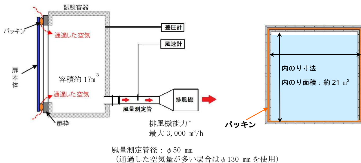
図 5-1 気密性能試験装置図
