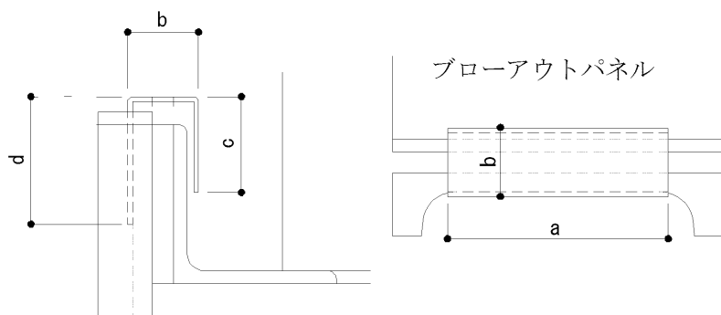
図 4-2 クリップの形状及び試験体寸法測定箇所
