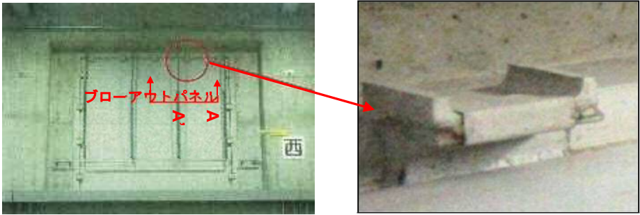
建屋内側よりの状況（6 階西側） クリップ部拡大（ A-A’ 矢視）
