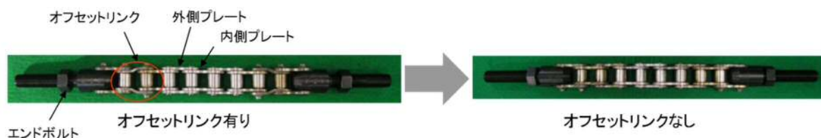
図 2-9 現設計チェーンと新設計のチェーンの比較
