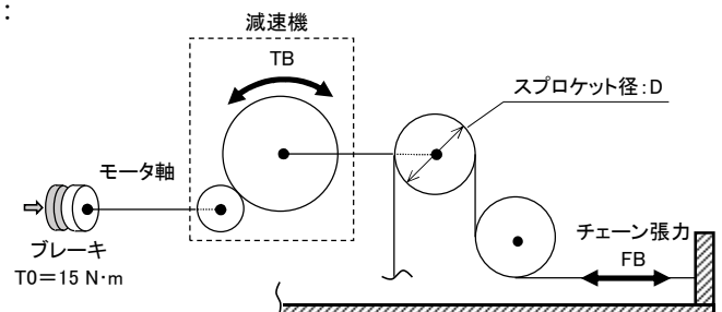
図 3-1 荷重伝達経路の模式図
