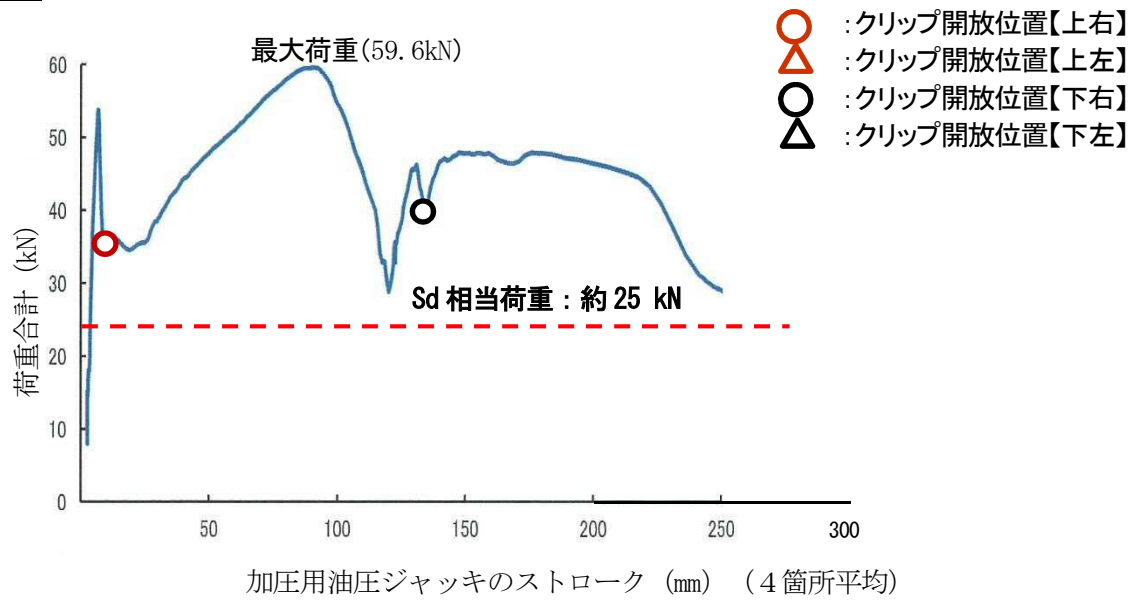
図 2-1(1) 油圧ジャッキの荷重合計と変位図
