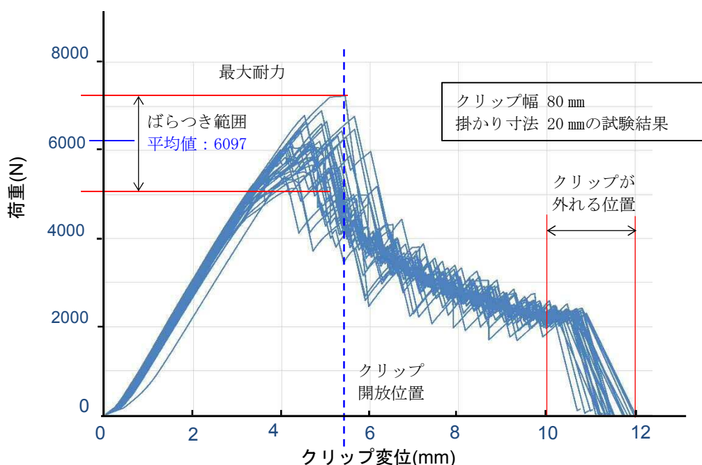
図 4-4 クリップの荷重・変位の関係
