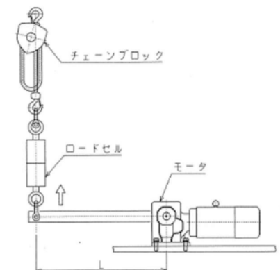
電動機ブレーキトルク試験概略図
