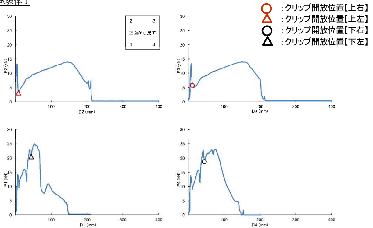
図 2-1(2) 各油圧ジャッキの荷重と変位測定結果 (1 回目)
