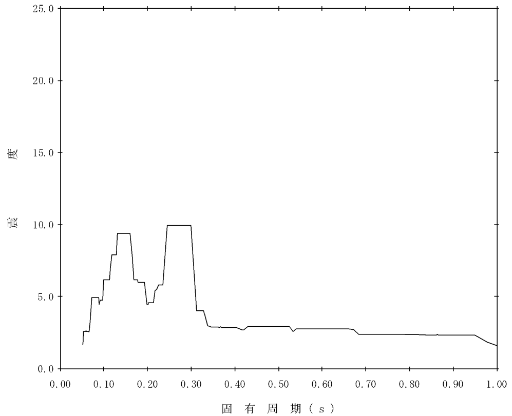
图4-14 床応答曲線(2/12) (減衰 1 % N-S方向(④-④断面) EL. 0.3 m : 鉛直)
