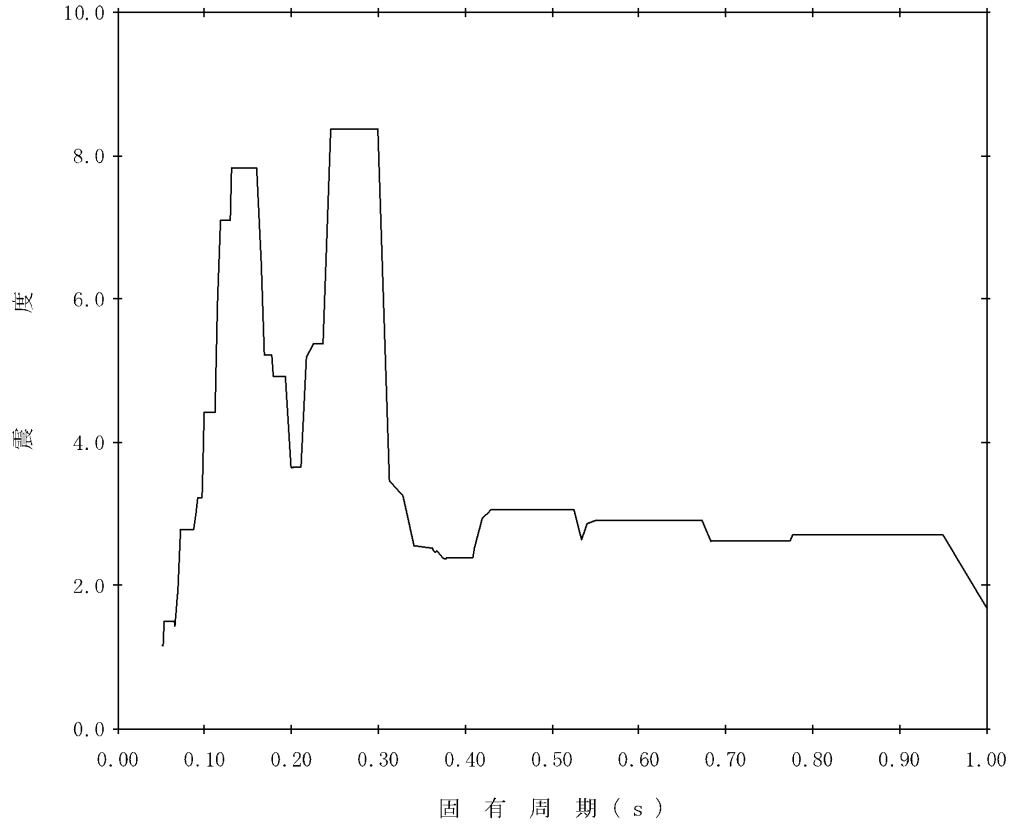
图4-14 床応答曲線(4/12) (減衰 1 % E-W方向(⑥-⑥断面) EL. 6.6 m : 鉛直)
