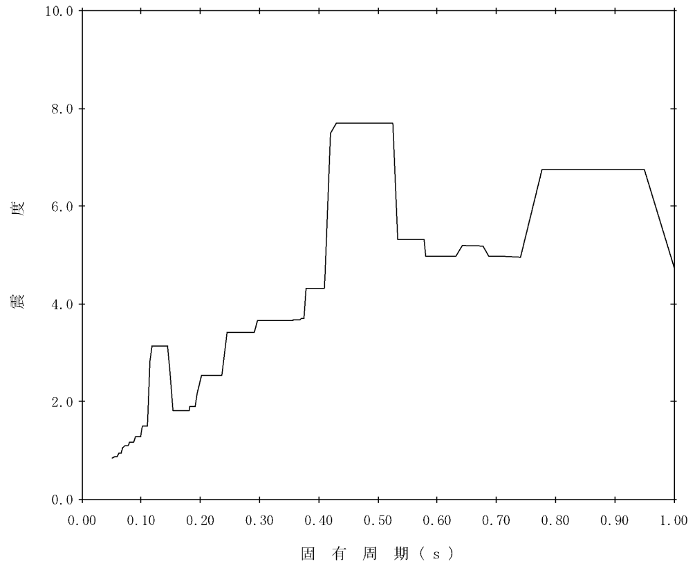
图4-14 床応答曲線(3/12) (減衰 1 % E-W方向(⑥-⑥断面) EL. 6.6 m : 水平)
