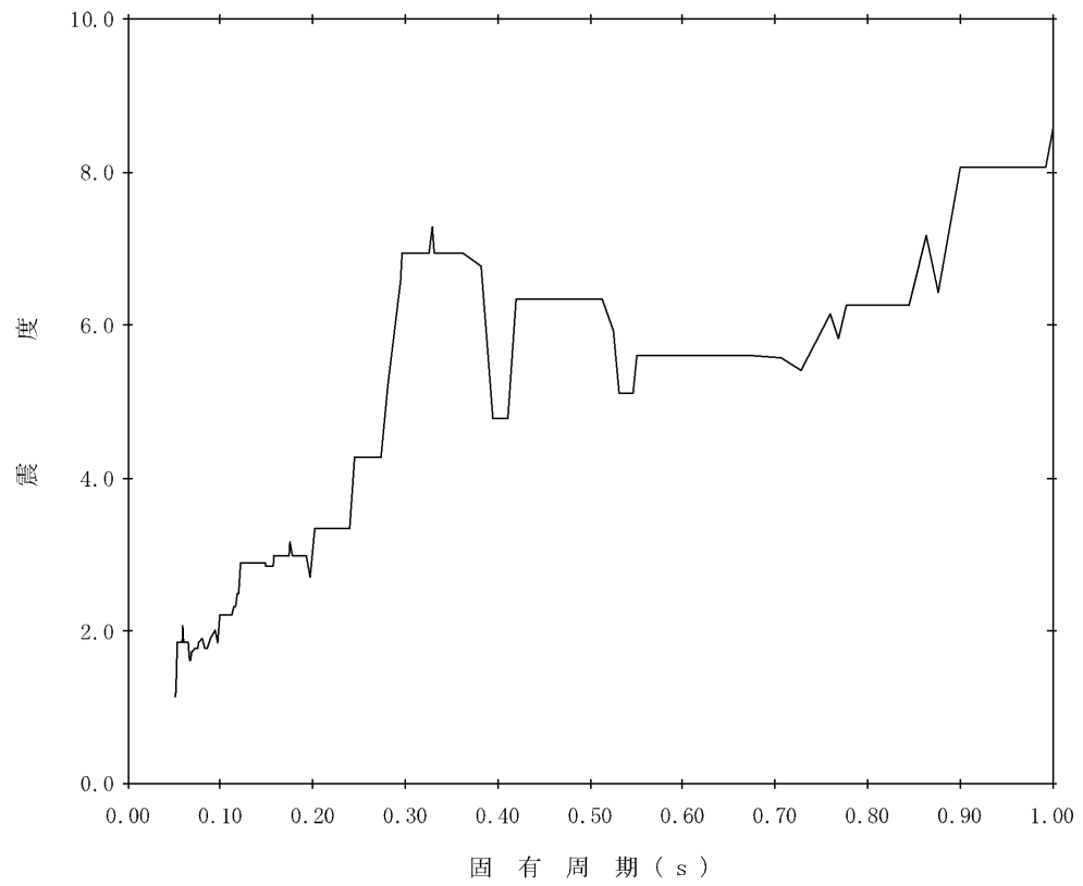
图4-14 床応答曲線(1/12) (減衰 1 % N-S方向(④-④断面) EL. 0.3 m : 水平)
