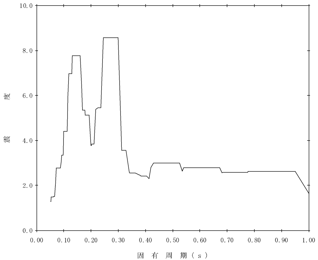
图4-14 床応答曲線(6/12) (減衰 1 % E-W方向(⑥-⑥断面) EL. 3.310 m : 鉛直)
