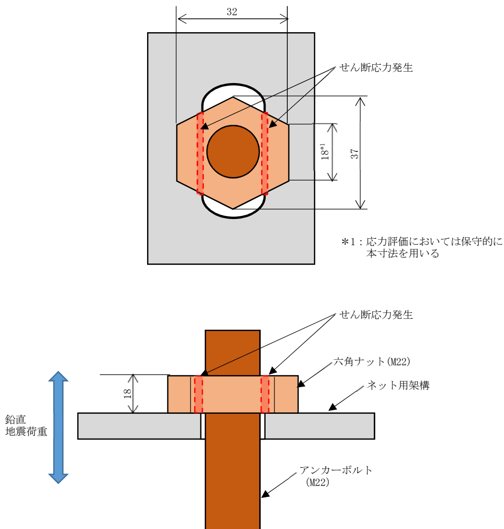
図 4-2 鉛直地震荷重により六角ナットに生じるせん断応力
