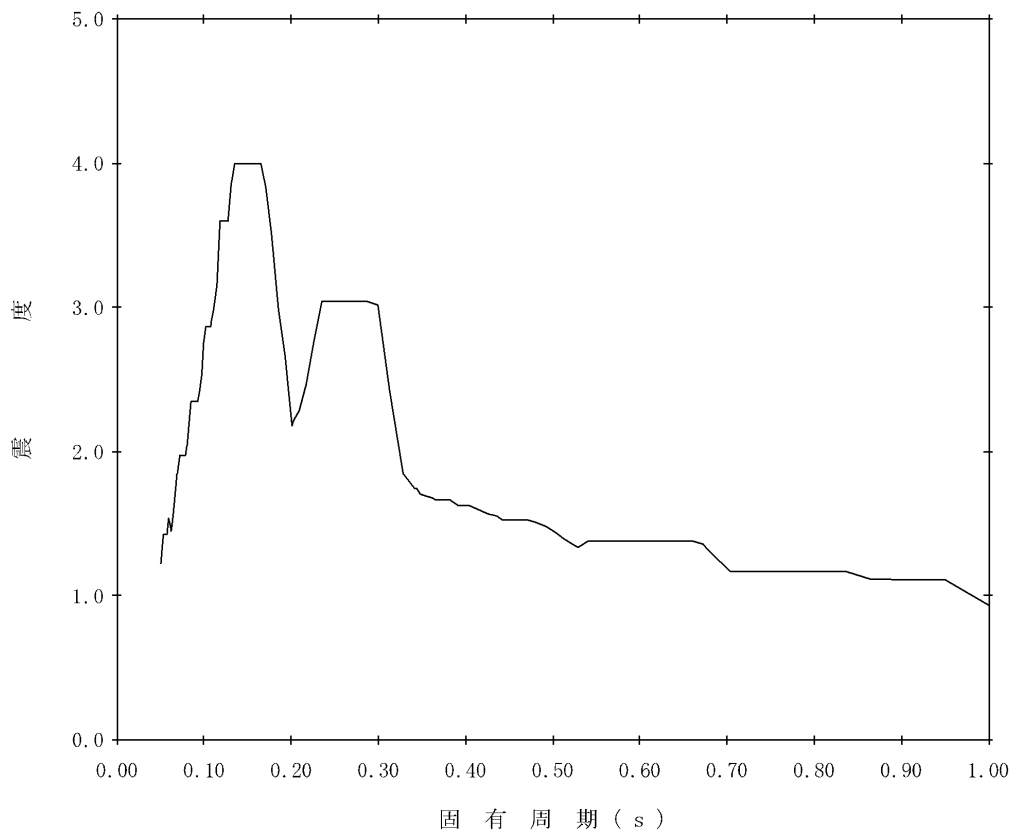
图4-14 床応答曲線(8/12) (減衰 5 % N-S方向(④-④断面) EL. 0.3 m : 鉛直)
