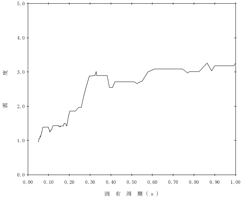
图4-14 床応答曲線(7/12) (減衰 5 % N-S方向(④-④断面) EL. 0.3 m : 水平)
