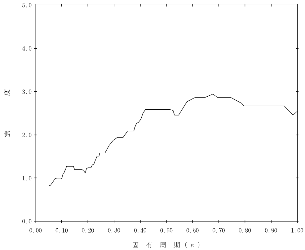
图4-14 床応答曲線(11/12) (減衰 5 % E-W方向(⑥-⑥断面) EL. 3.310 m : 水平)
