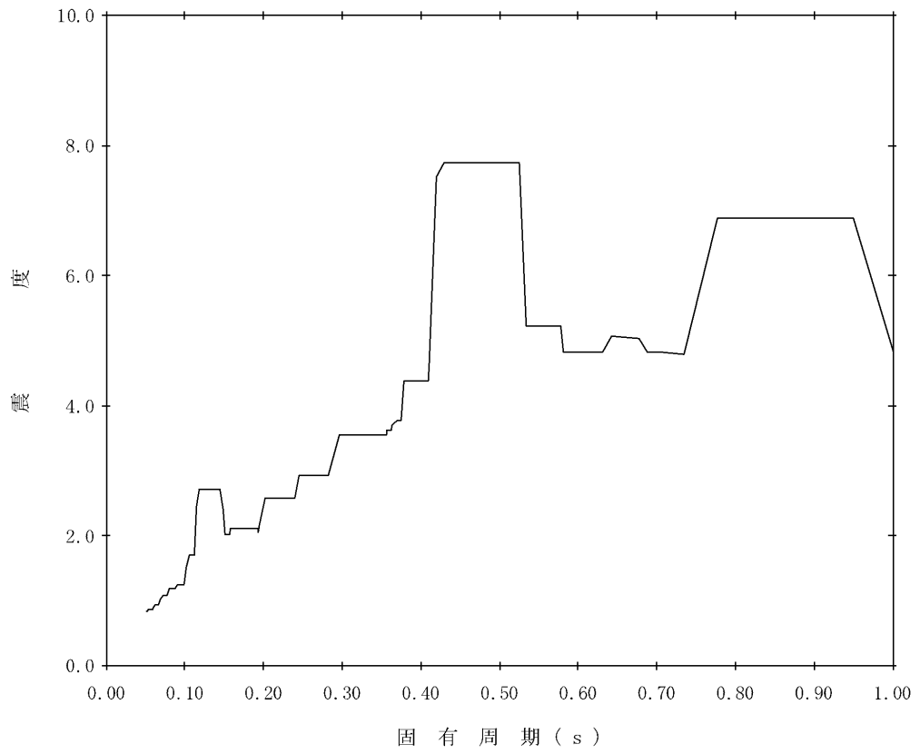
图4-14 床応答曲線(5/12) (減衰 1 % E-W方向(⑥-⑥断面) EL. 3.310 m : 水平)
