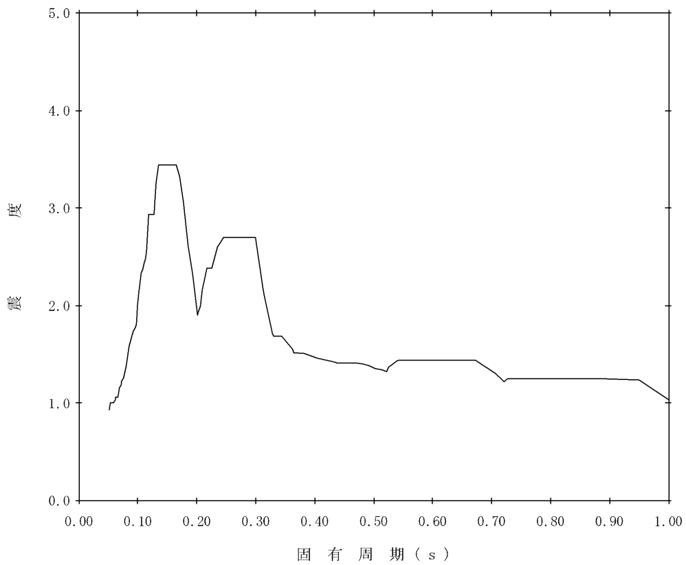
图4-14 床応答曲線(12/12) (減衰 5 % E-W方向(⑥-⑥断面) EL. 3.310 m : 鉛直)
