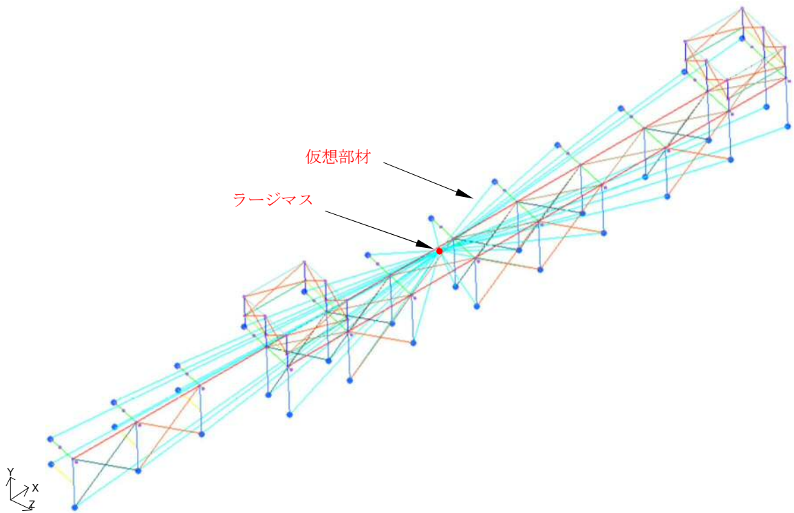
図 4-10 鉄骨架構の強度評価モデルへの入力荷重(地震荷重)
