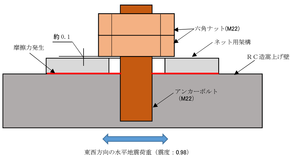
図 4-3 ネット用架構に生じる静摩擦力及び水平地震荷重
