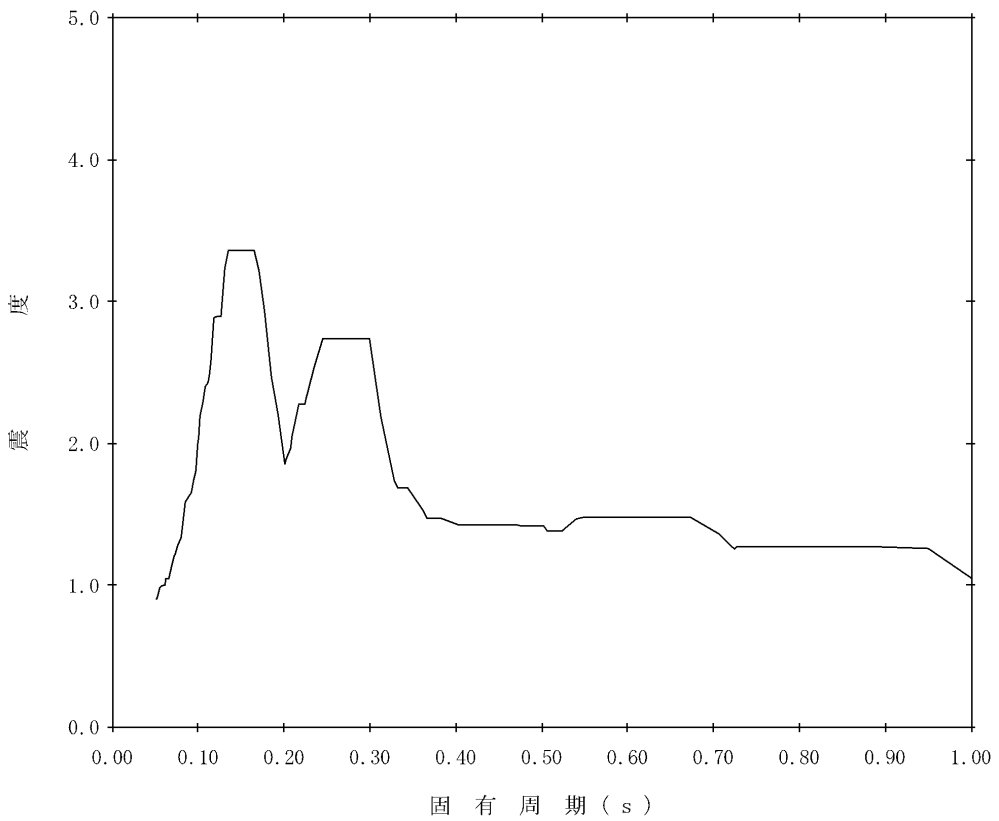
图4-14 床応答曲線(10/12) (減衰 5 % E-W方向(⑥-⑥断面) EL. 6.6 m : 鉛直)
