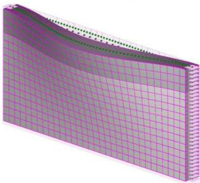
図4-12 振動モード図 (RC造躯体) (1/2)
