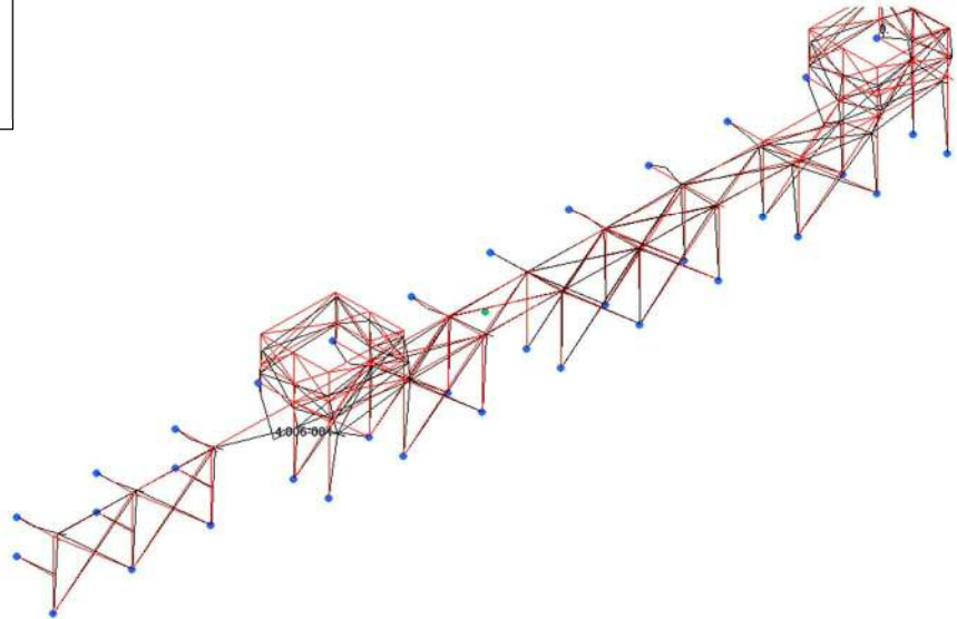
図4-11 振動モード図 (ネット架構及び鉄骨架構) (6/6) (◇-1)
