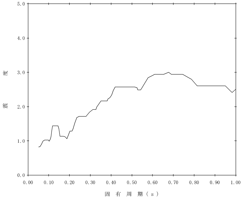
图4-14 床応答曲線(9/12) (減衰 5 % E-W方向(⑥-⑥断面) EL. 6.6 m : 水平)
