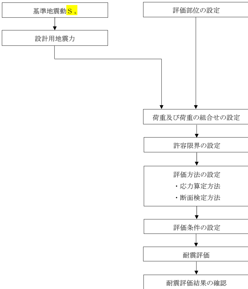
図2-6 水密扉の耐震評価の確認フロー
