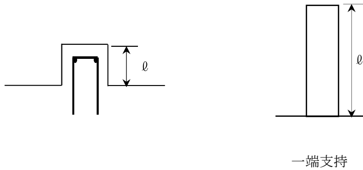
図3-1 堰の評価モデル図
