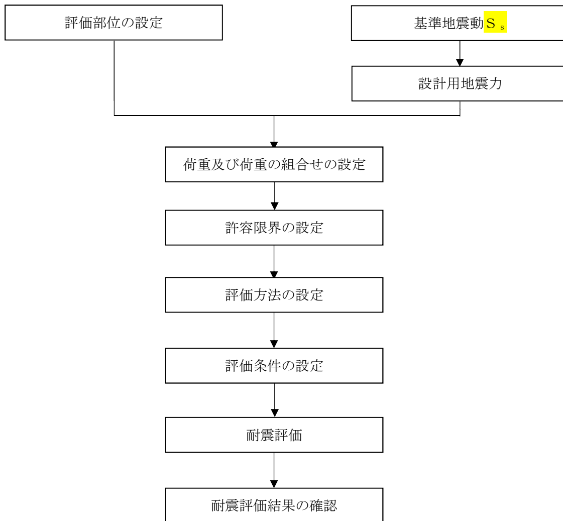
図 2-2 堰の耐震評価フロー
