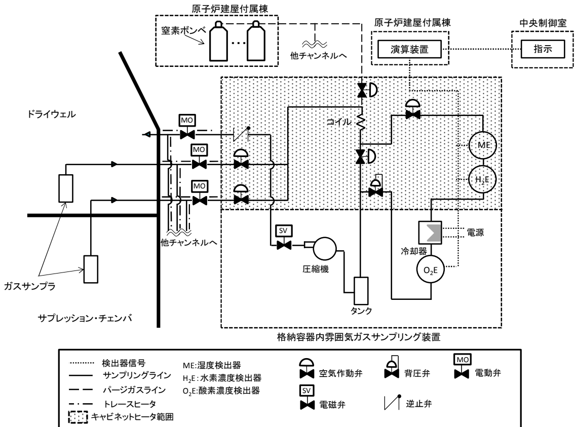
図 2.2.1-1 格納容器内雰囲気ガスサンプリング装置の概略構成図
