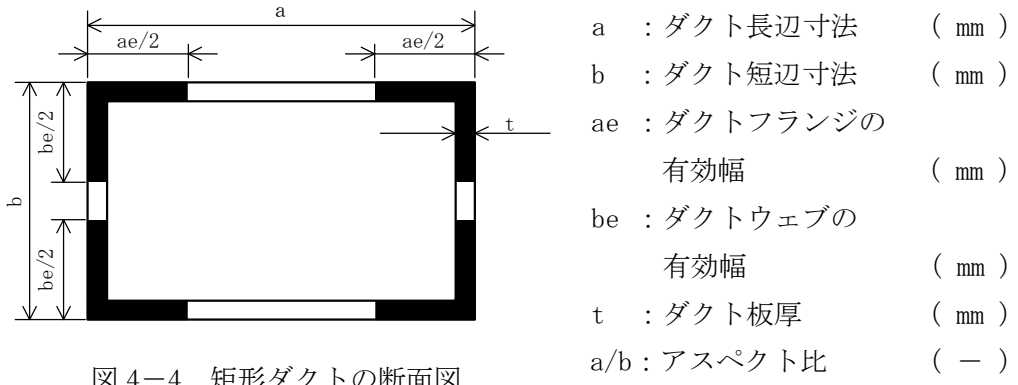
図 4-4 矩形ダクトの断面図
