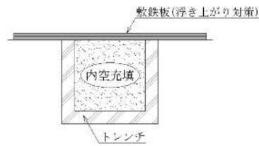
タイプC (内空充填)
