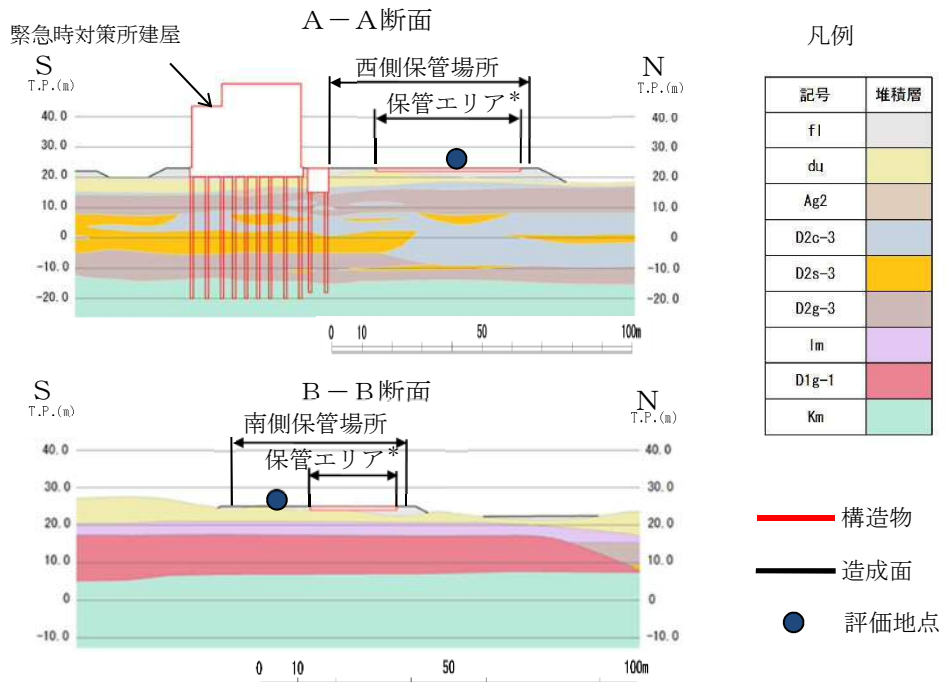
第 2-5 図 保管場所における液状化及び揺すり込み沈下による 不等沈下に対する影響評価断面の位置図及び断面図
