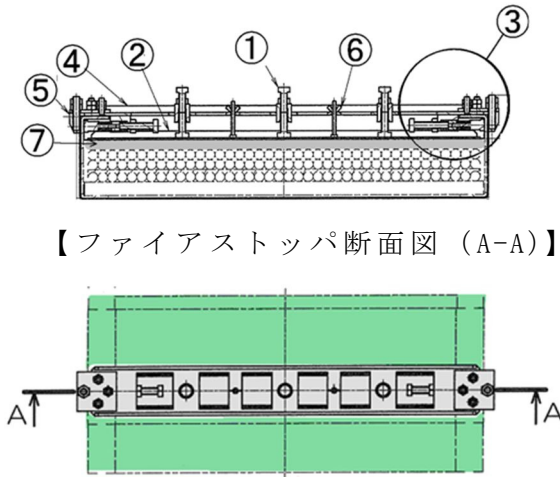
【ファイアストップ正面図】
