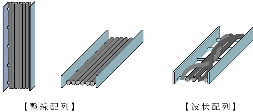
第 5 図 ケーブルの配列
