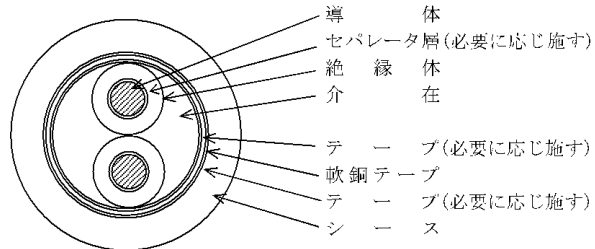
CCV-S 構造 (例)
