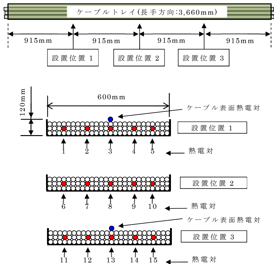
第 1 図 熱電対設置位置
