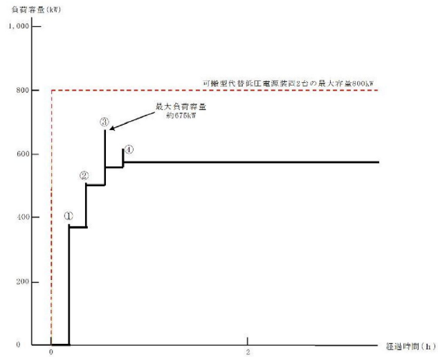
可能型代替低圧電源車の負荷積算イメージ
