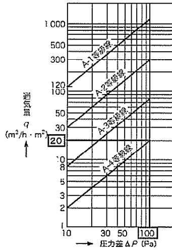
図1-気密等級線
