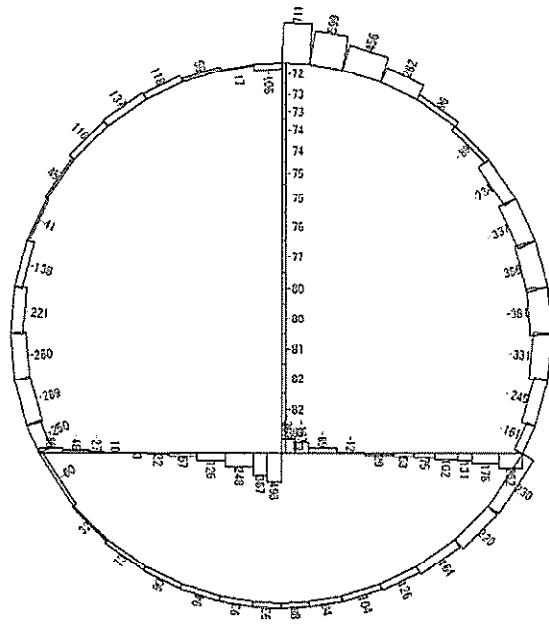
せん断力 (kN)
