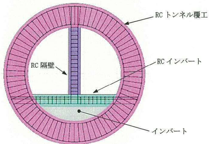
参考図 5-3 (2) トンネルの配筋イメージ
