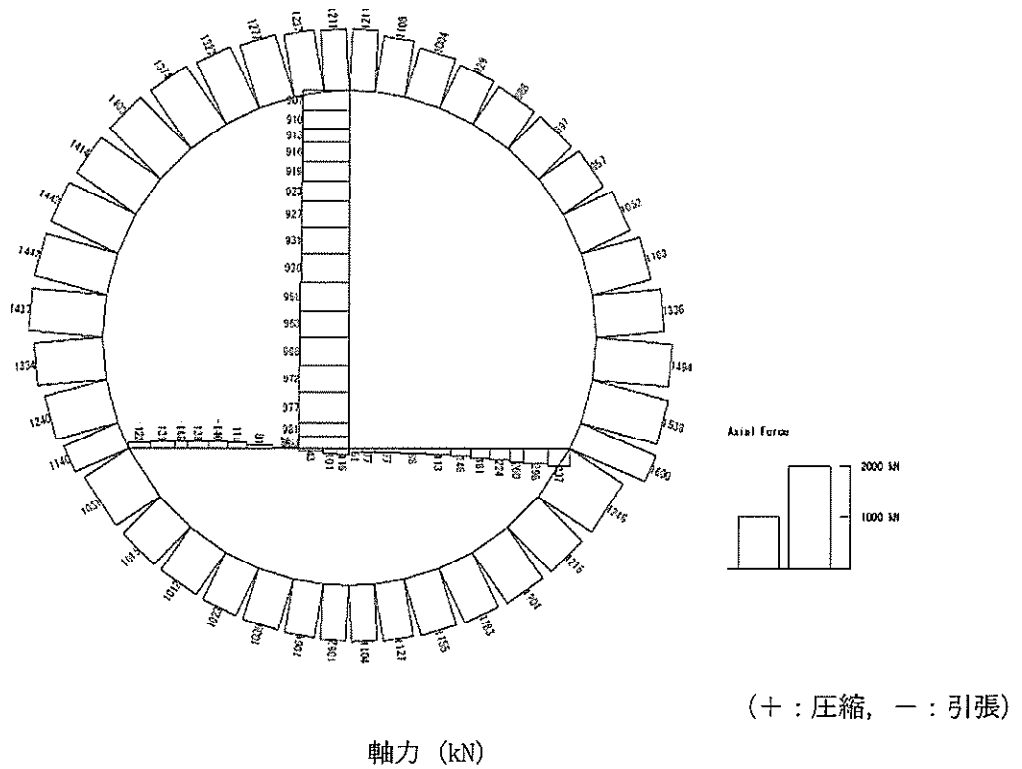
図 5.4-6 (15) S_s-14 (H+, V+) において最も厳しい照査値となる時刻の断面力 (t=28.96s)
