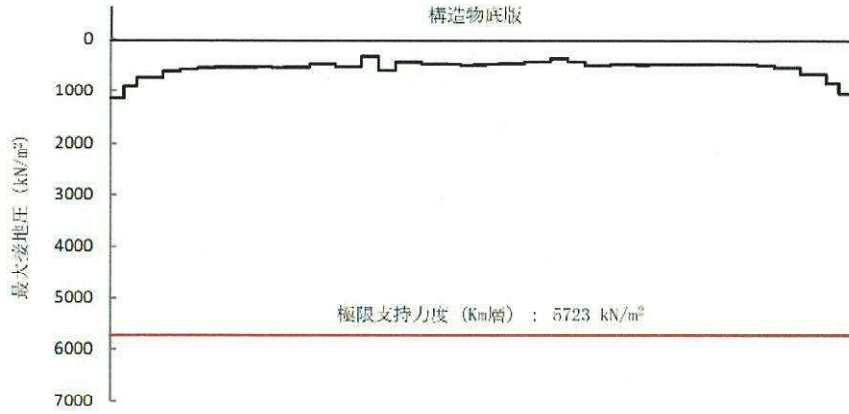
図 4.4-15 (7) 接地圧分布図 (S s -13)
