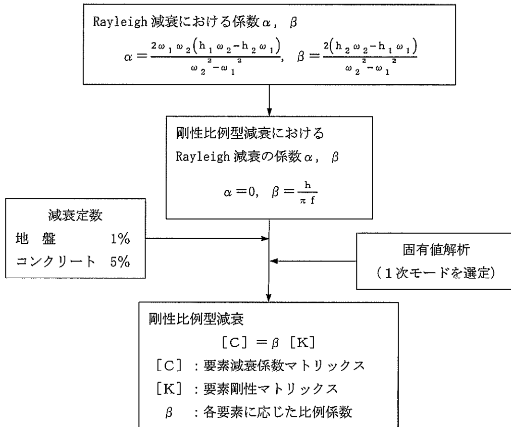
図 5.2-18 Rayleigh 減衰の設定フロー
