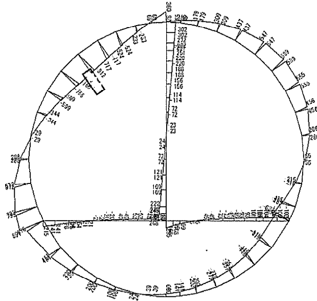
曲げモーメント (kN・m)
