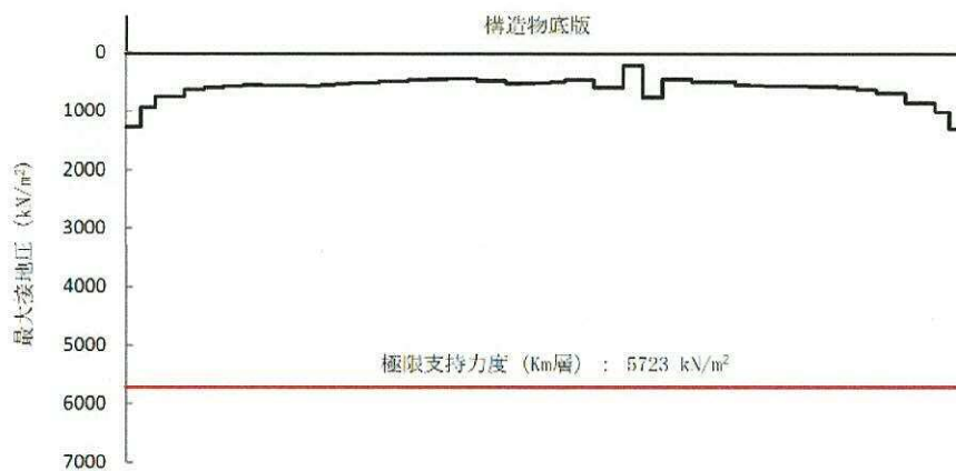
図 4.4-15 (18) 接地圧分布図 (S s -D 1 (H-, V-)) (検討ケース③: 地盤物性のばらつきを考慮 (-1σ) した解析ケース)
