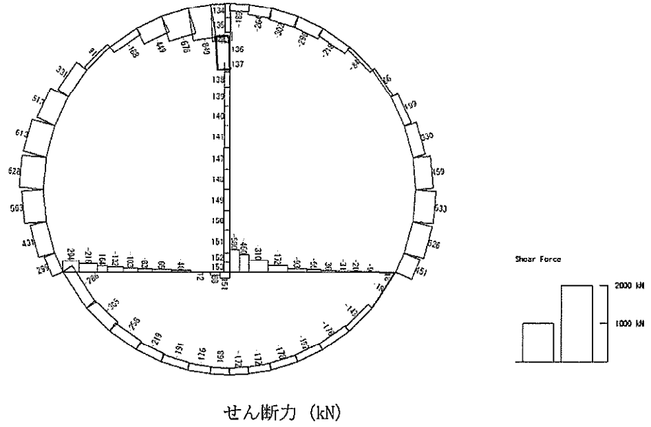
せん断力 (kN) 図 5.4-5 (2) RC トンネル覆工において最も厳しい照査値となる時刻の断面力 (S s -31 (H+, V+), t=8.74s) (検討ケース②: 地盤物性のばらつきを考慮 (+1σ) した解析ケース)
