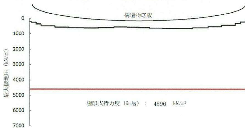
図 5.4-12 (12) 接地圧分布図 (S s -31 (H-, V+))
