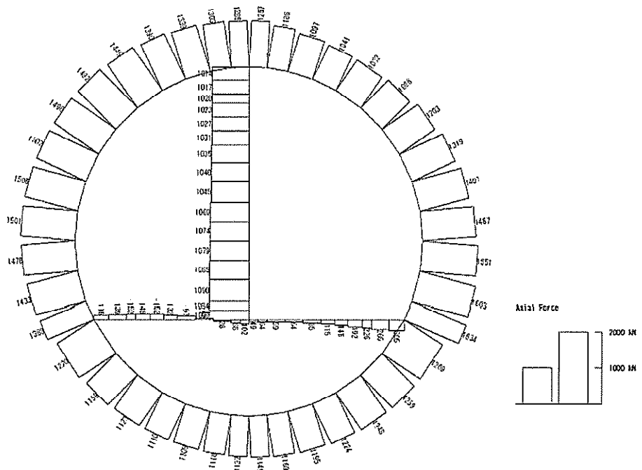
軸力 (kN)
