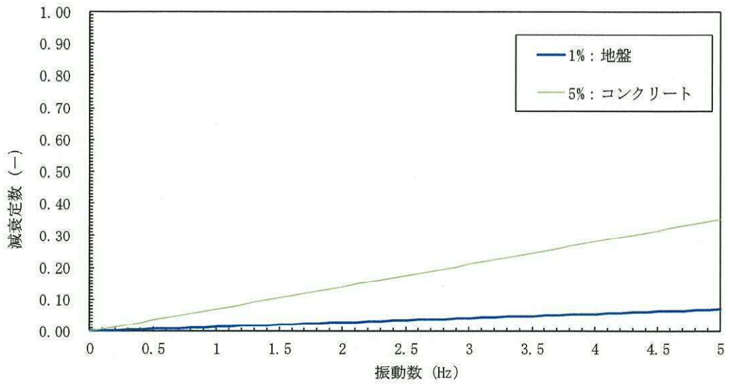
参考図 5-2 (3) 設定した Rayleigh 減衰
