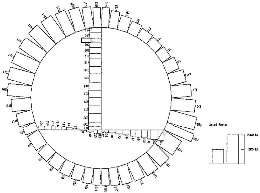
軸力 (kN)
