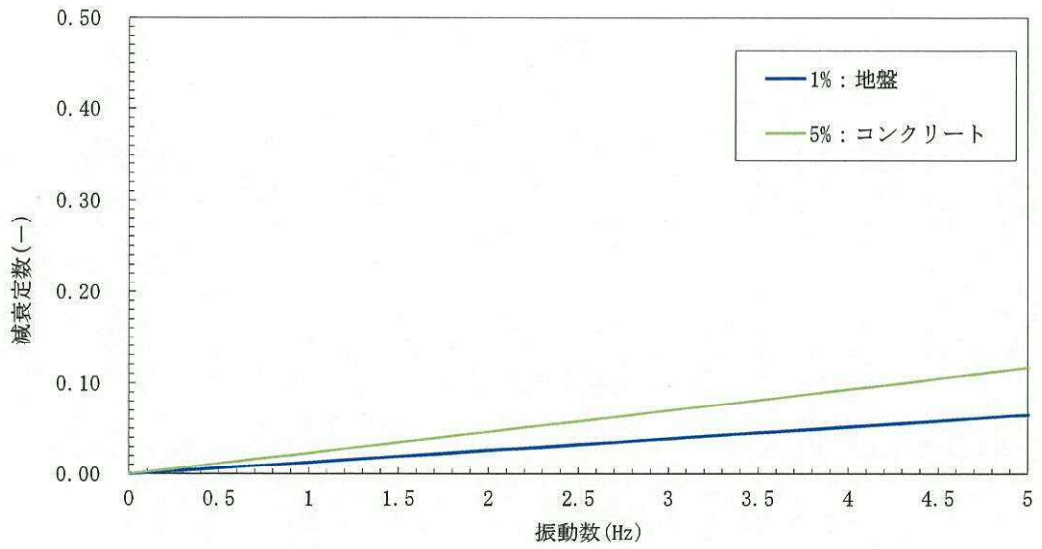
参考図 4-2 (3) 設定した Rayleigh 減衰
