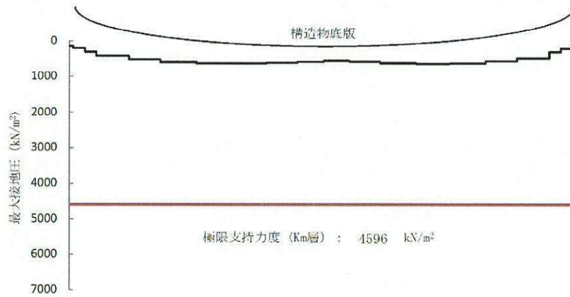
図 5.4-12 (14) 接地圧分布図 (S s -31 (H+, V+)) (検討ケース③: 地盤物性のばらつきを考慮 (-1σ) した解析ケース)
