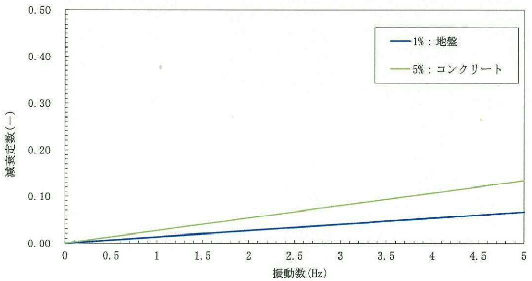
参考図 4-2 (4) 設定した Rayleigh 減衰
