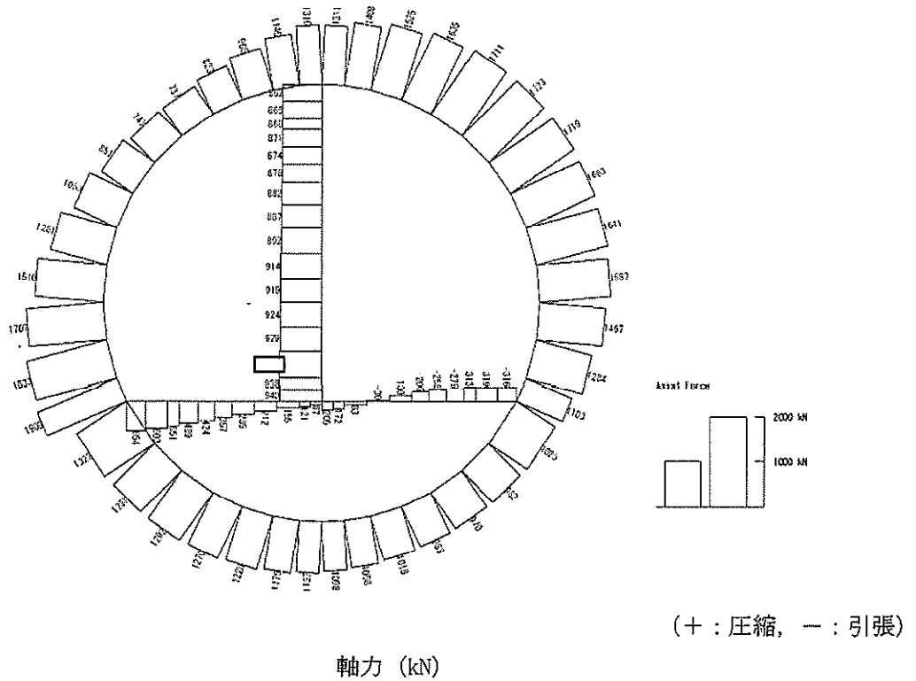
図 5.4-5 (3) RC 隔壁において最も厳しい照査値となる時刻の断面力 (S s -31 (H+, V+), t=8.73s) (検討ケース②: 地盤物性のばらつきを考慮 (+1σ) した解析ケース)
