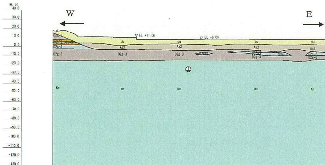
図 5.2-11 地質断面図
