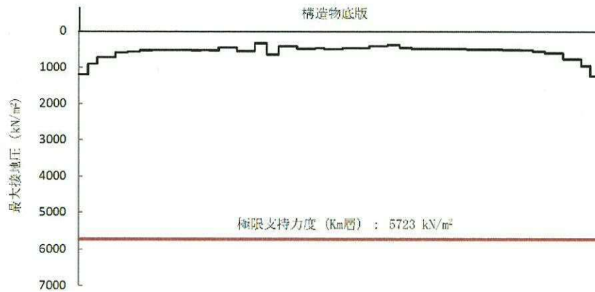
図 4.4-15 (9) 接地圧分布図 (S s -21)
