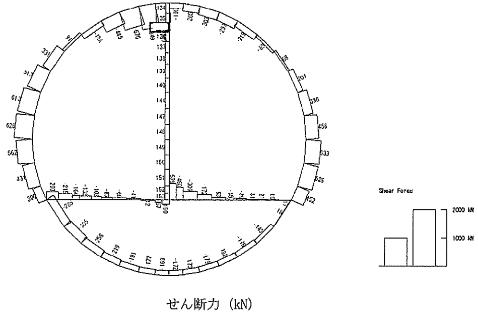
図 5.4-3 (4) RC 隔壁において最も厳しい照査値となる時刻の断面力 (S s -31 (H+, V+), t=8.73s) (検討ケース②: 地盤物性のばらつきを考慮 (+1σ) した解析ケース)
