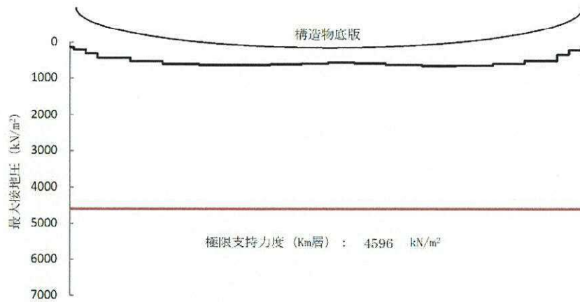
図 5.4-12 (13) 接地圧分布図 (S s -31 (H+, V+)) (検討ケース②: 地盤物性のばらつきを考慮 (+1σ) した解析ケース)
