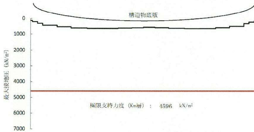
図 5.4-12 (11) 接地圧分布図 (S s -31 (H+, V+))
