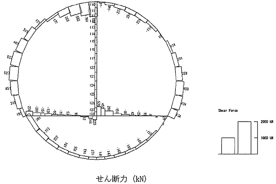
図 5.4-6 (6) S_s-D1 (H-, V+) において最も厳しい照査値となる時刻の断面力 ( t = 53.84s )
