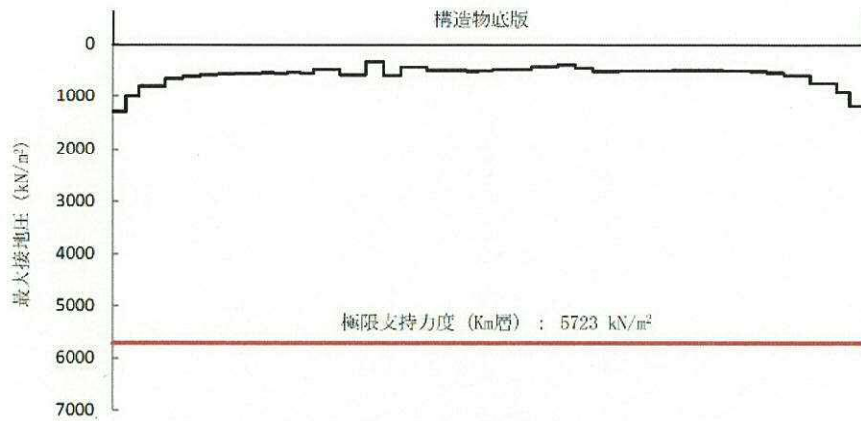
図 4.4-15 (10) 接地圧分布図 (S s -2 2)
