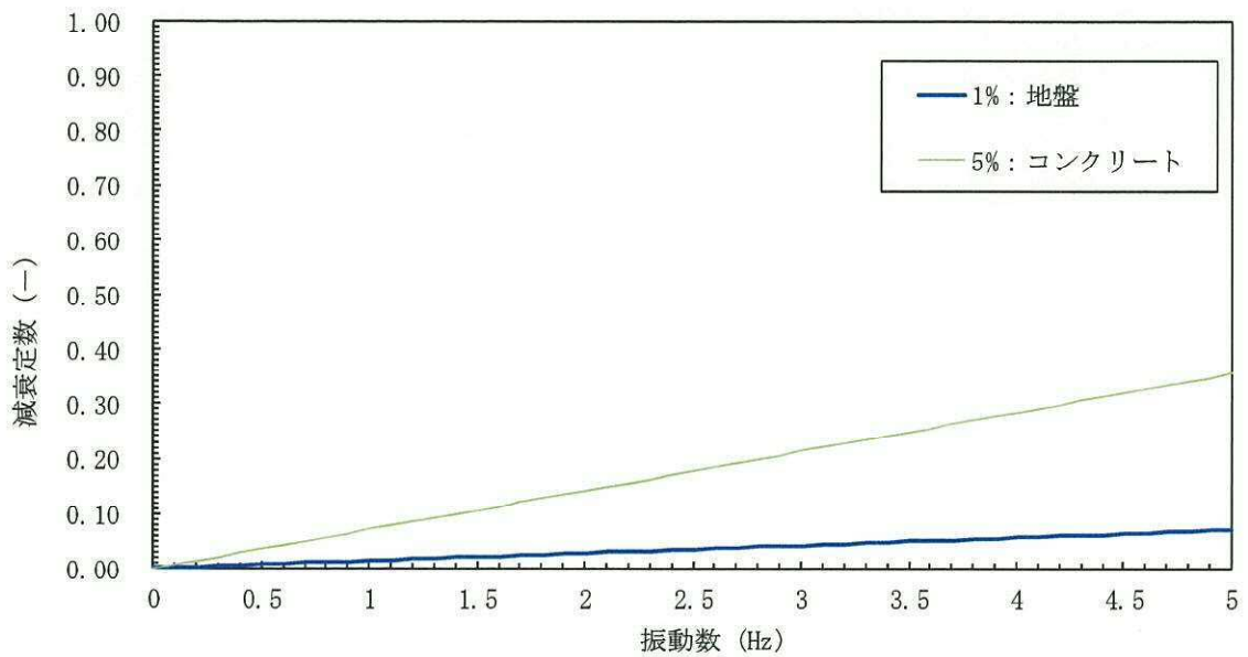
参考図 5-2 (4) 設定した Rayleigh 減衰
