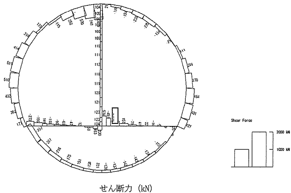
図 5.4-5 (6) RC インバートにおいて最も厳しい照査値となる時刻の断面力 ( S_s-D1 (H-, V+), t=53.81s ) (検討ケース①: 原地盤に基づく液状化強度特性を用いた解析ケース)
