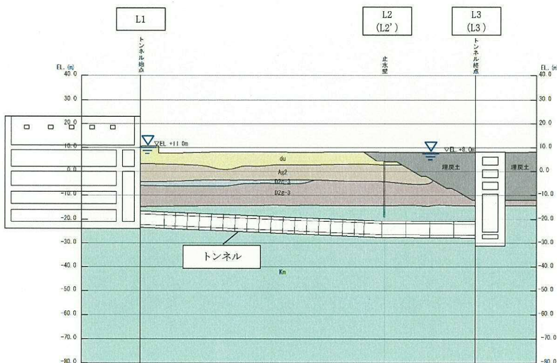
図 5.2-4 トンネルの縦断図
