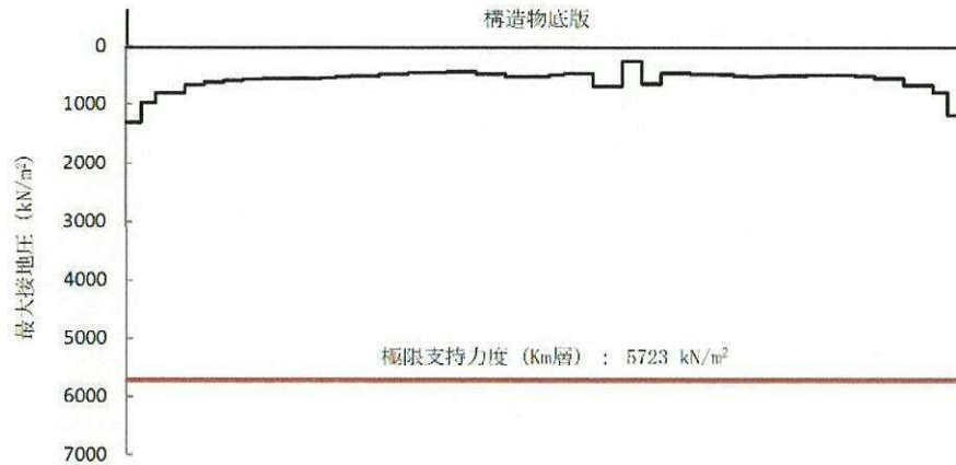
図 4.4-15 (16) 接地圧分布図 (S s -D 1 (H+, V+)) (検討ケース③: 地盤物性のばらつきを考慮 (-1σ) した解析ケース)
