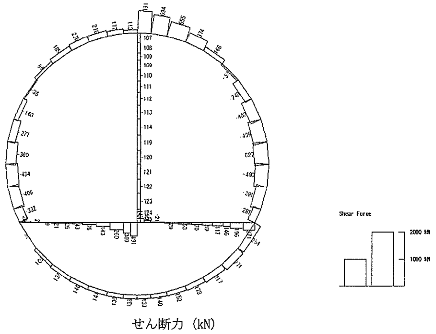
図 5.4-6 (4) S s -D 1 (H+, V-) において最も厳しい照査値となる時刻の断面力 ( t = 53.84s)
