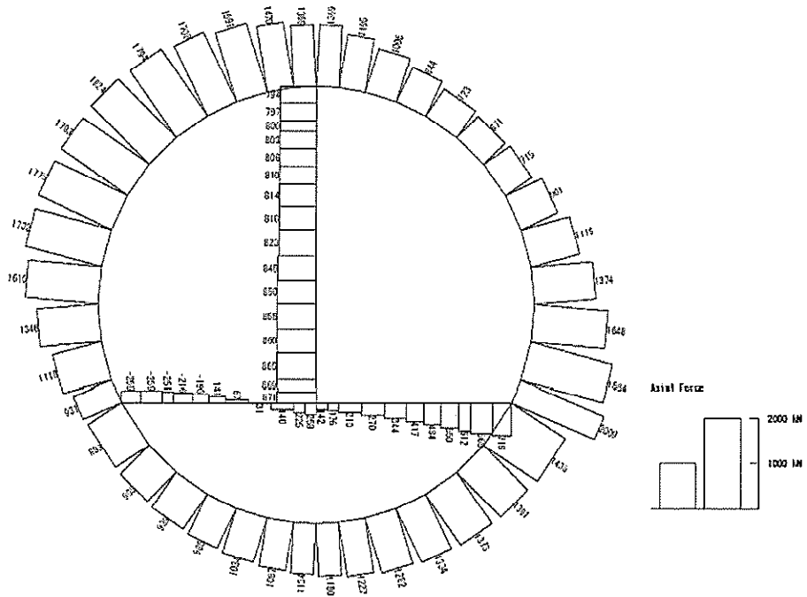
軸力 (kN)
