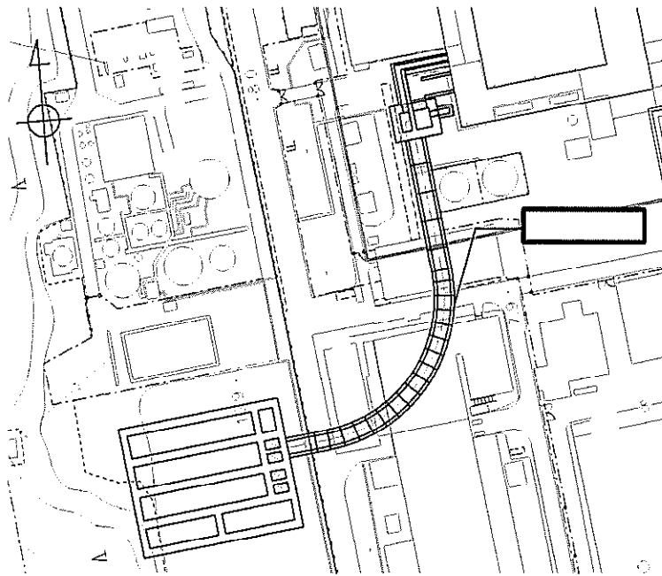
図 5.2-3 トンネルの位置図 (拡大図)
