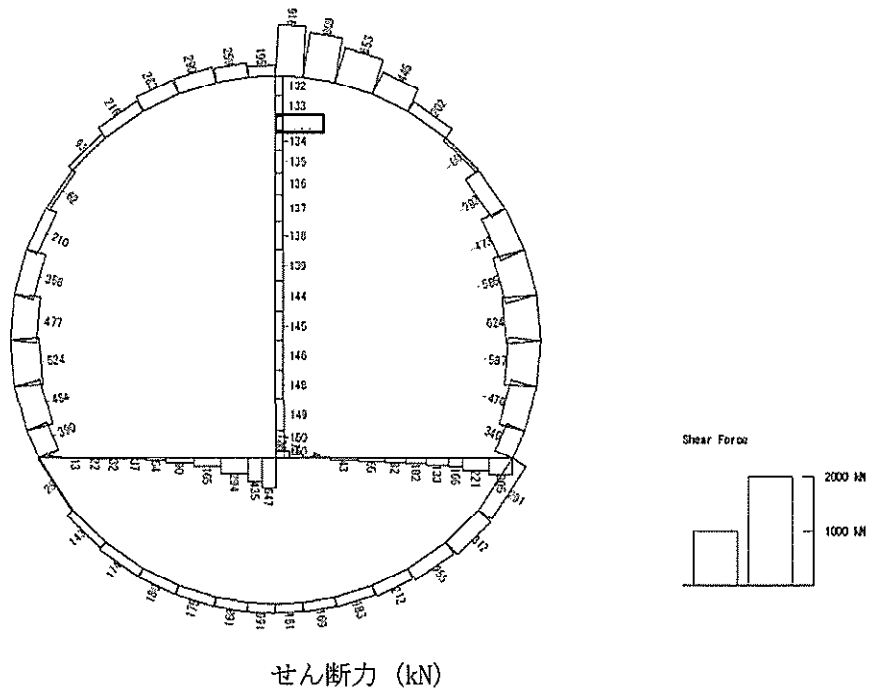
図 5.4-4 (4) RC 隔壁において最も厳しい照査値となる時刻の断面力 (S s -31 (H-, V+), t=8.73s) (検討ケース①: 原地盤に基づく液状化強度特性を用いた解析ケース)
