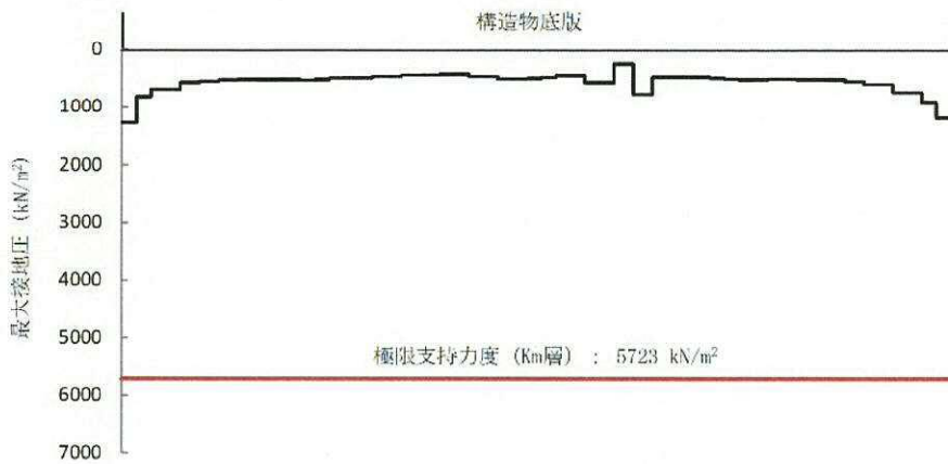
図 4.4-15 (17) 接地圧分布図 (S s -D 1 (H-, V+)) (検討ケース③: 地盤物性のばらつきを考慮 (-1σ) した解析ケース)
