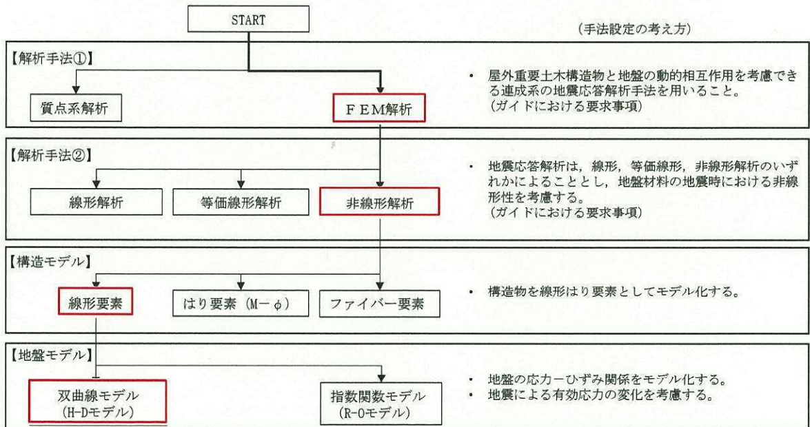
図 5.2-8 地震応答解析手法の選定フロー
