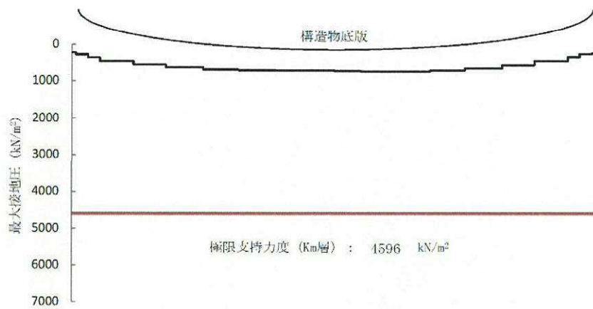
図 5.4-12 (10) 接地圧分布図 (S s -22)
