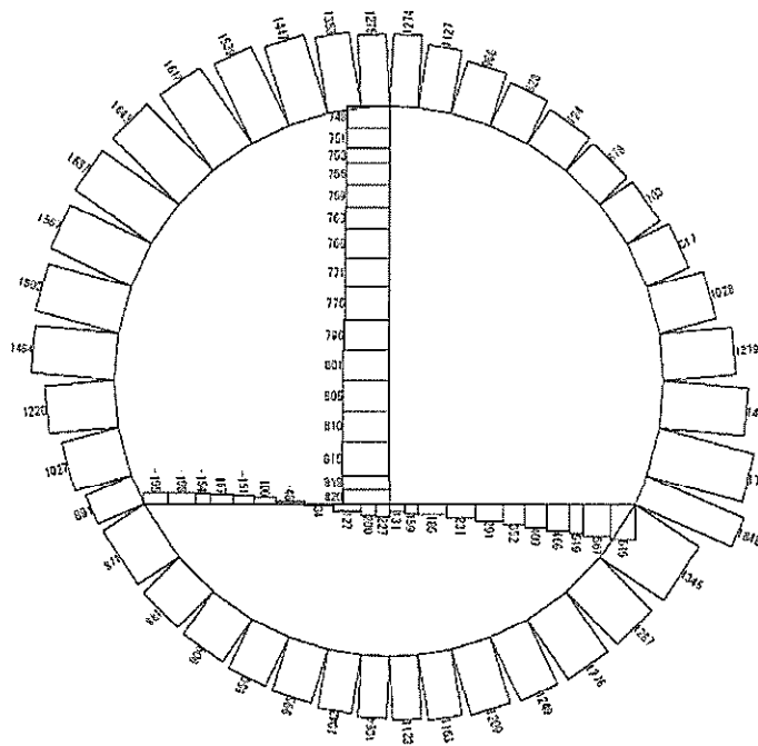
軸力 (kN)
