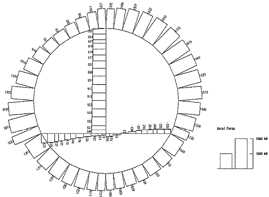
軸力 (kN)
