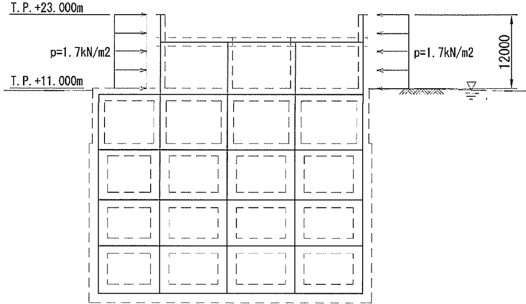
参考図 4-3 風荷重の作用方法
