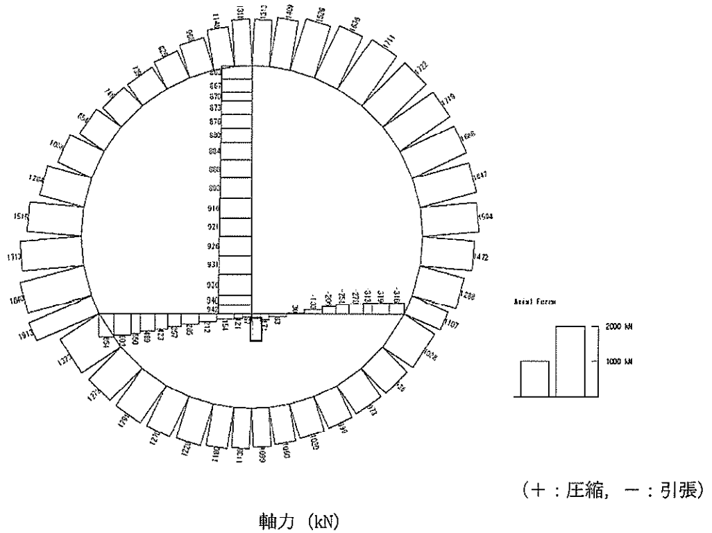
図 5.4-3 (5) RC インバートにおいて最も厳しい照査値となる時刻の断面力 (S s -31 (H+, V+), t=8.74s) (検討ケース②: 地盤物性のばらつきを考慮 (+1σ) した解析ケース)
