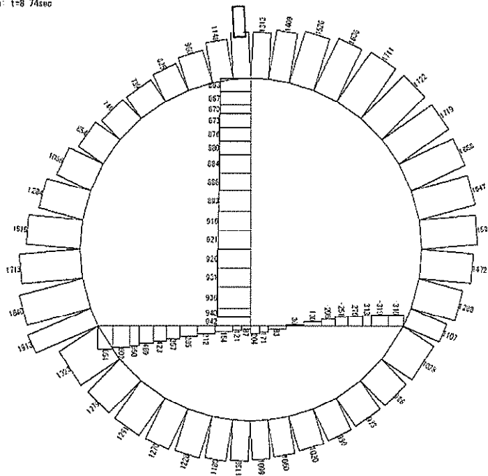
軸力 (kN)
