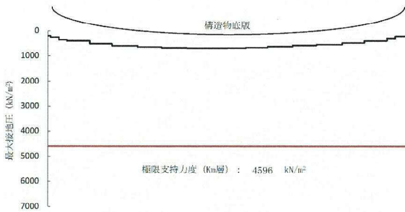
図 5.4-12 (7) 接地圧分布図 (S s -13)
