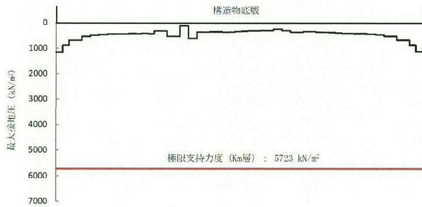
図 4.4-15 (11) 接地圧分布図 (S s -3 1 (H+, V+))
