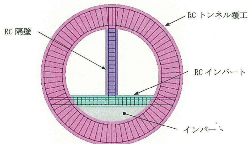
図 5.2-7 評価部位と配筋イメージ
