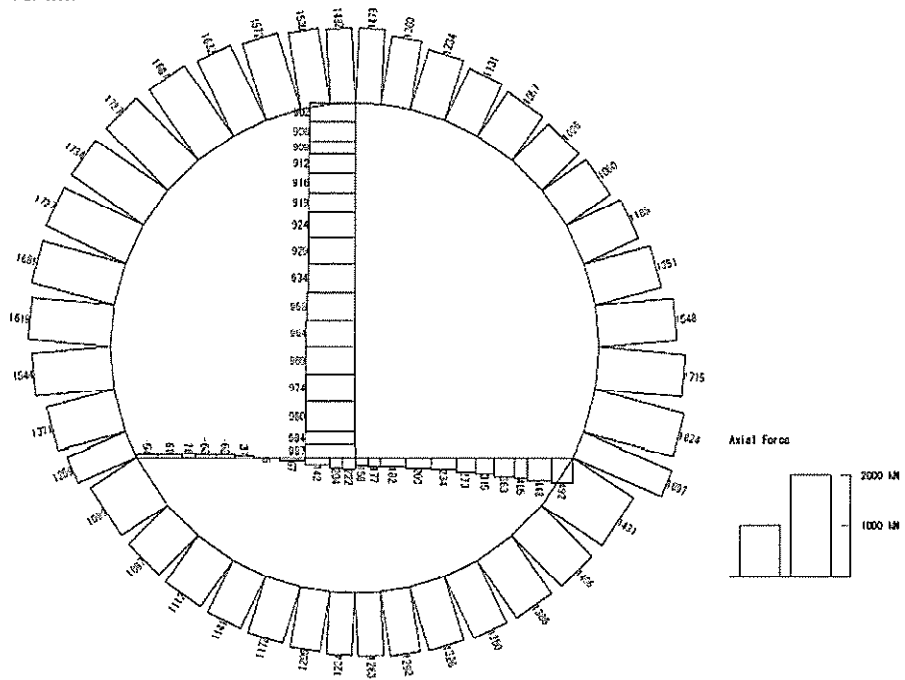
軸力 (kN)
