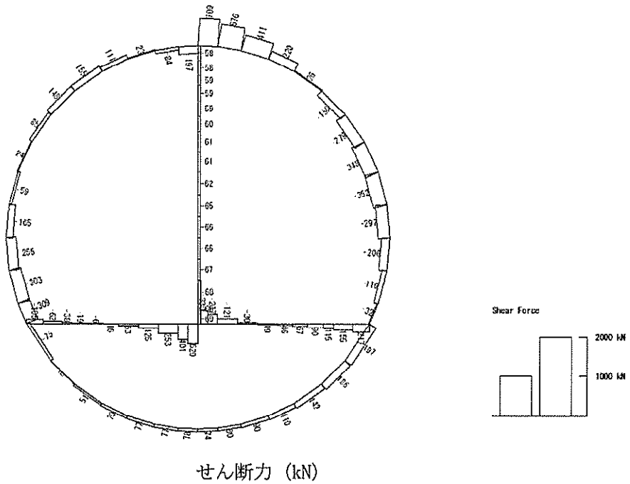
図 5.4-6 (14) S_s-13 (H+, V+) において最も厳しい照査値となる時刻の断面力 ( t = 26.64s )
