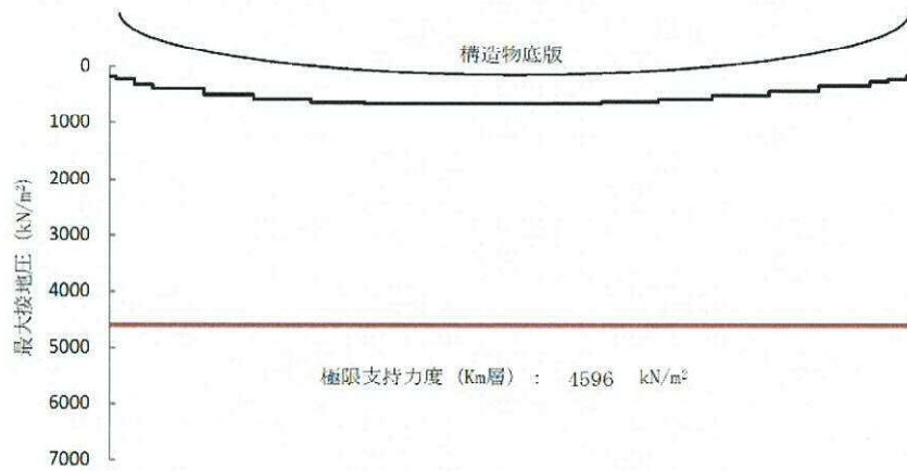
図 5.4-12 (8) 接地圧分布図 (S s -14)
