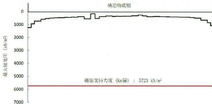
図 4.4-15 (12) 接地圧分布図 (S s -3 1 (H-, V+))
