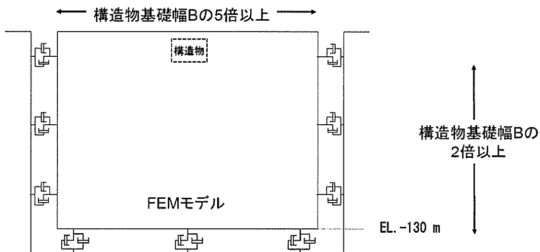
図 5.2-9 モデル範囲の考え方
