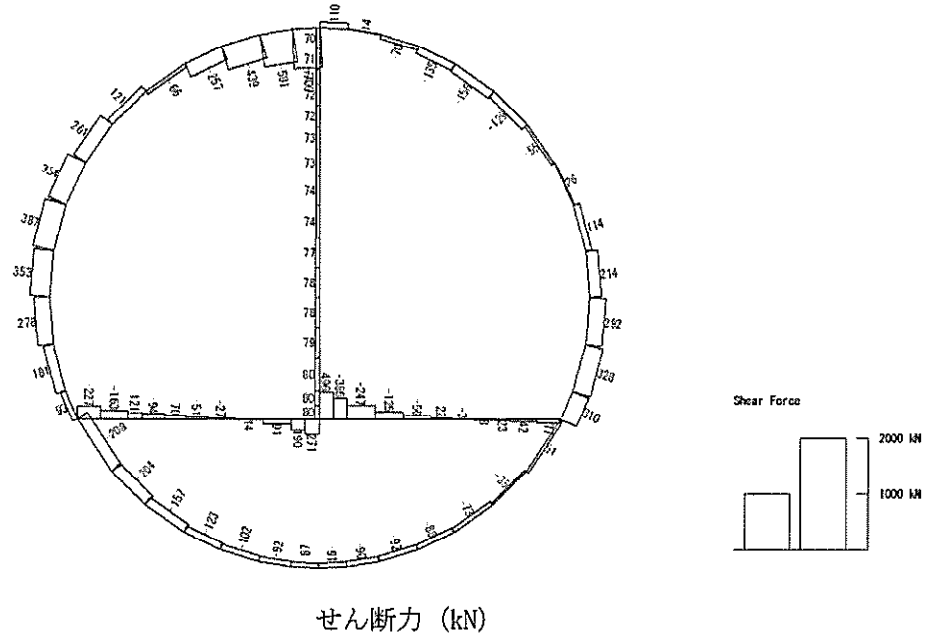
図 5.4-6 (18) S_s-21 (H+, V+) において最も厳しい照査値となる時刻の断面力 ( t=65.94s )
