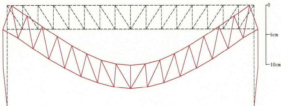
(a) 屋根スラブ剛性無視
