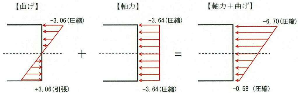
図 2-2 軸力を考慮した場合の応力度
