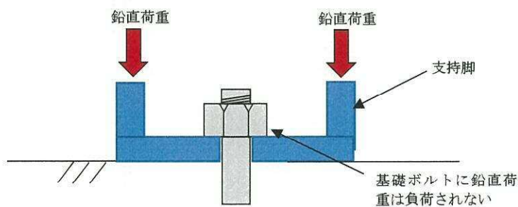
図 1 基礎ボルト部拡大図
