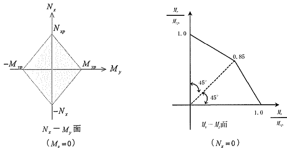
図 4-2 降伏曲面
