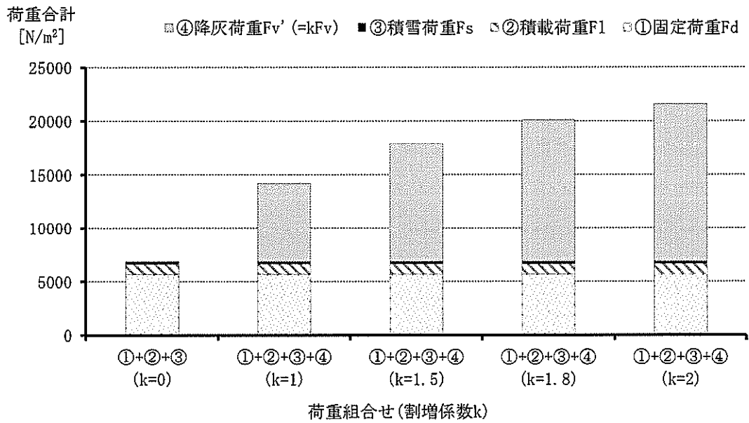
図 2-4 荷重組合せと荷重合計
