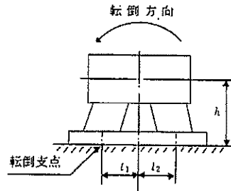
図 3 横形ポンプモデル図 (JEAG)
