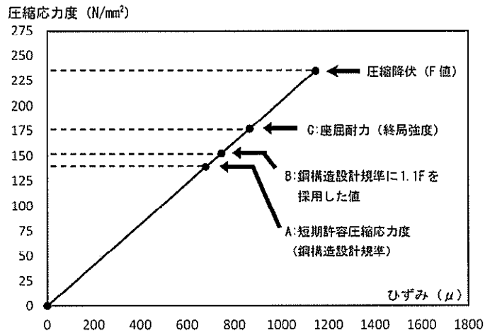
図 2 F 値×1.1 を適用し算定した強度と座屈耐力の比較例
