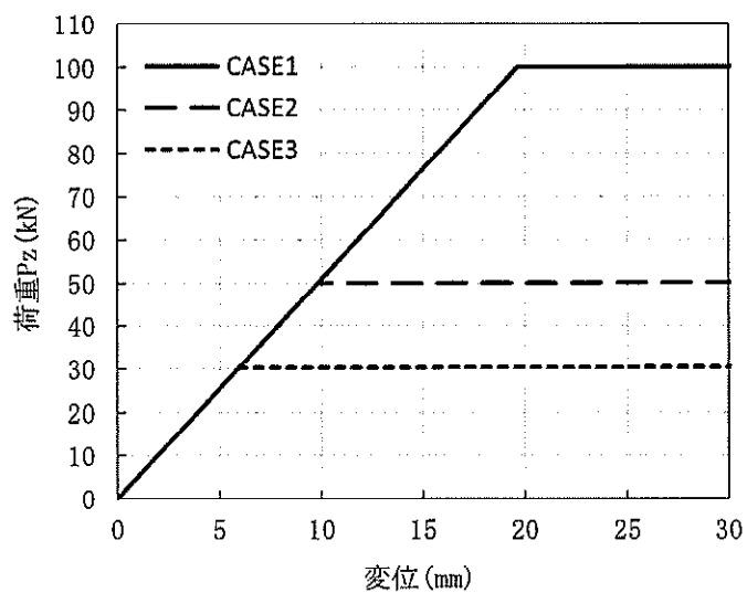
図4-3 荷重変位関係 (荷重ステップ2, A端)
