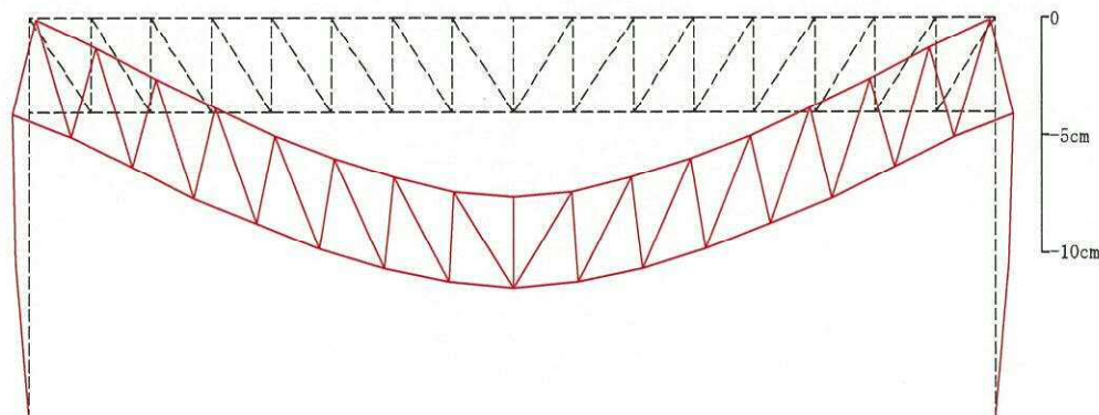
(b) 屋根スラブ剛性考慮
