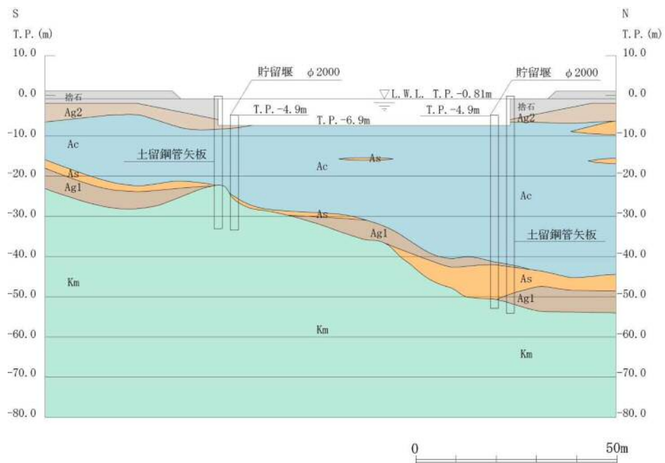
(断面図)
