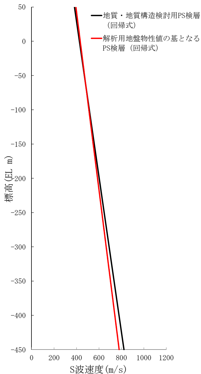
図 6.3-6 各 PS 検層の比較
