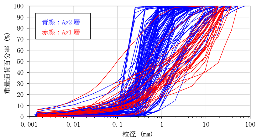
図5 Ag1層とAg2層の粒度分布の比較
