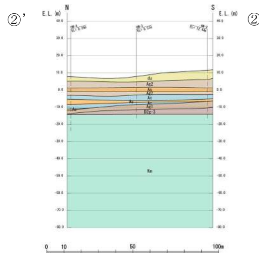
②—②' 断面
