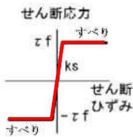
図8 杭軸方向ばねの力学特性
