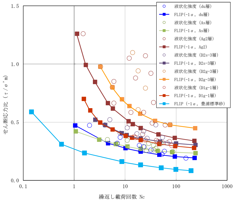
図 4.2-2 原地盤に基づく液化化強度特性と豊浦標準砂を仮定した液化化強度特性の比較
