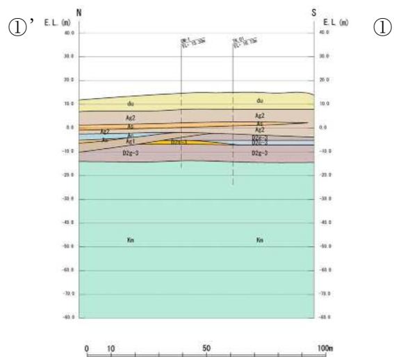
①—①' 断面
