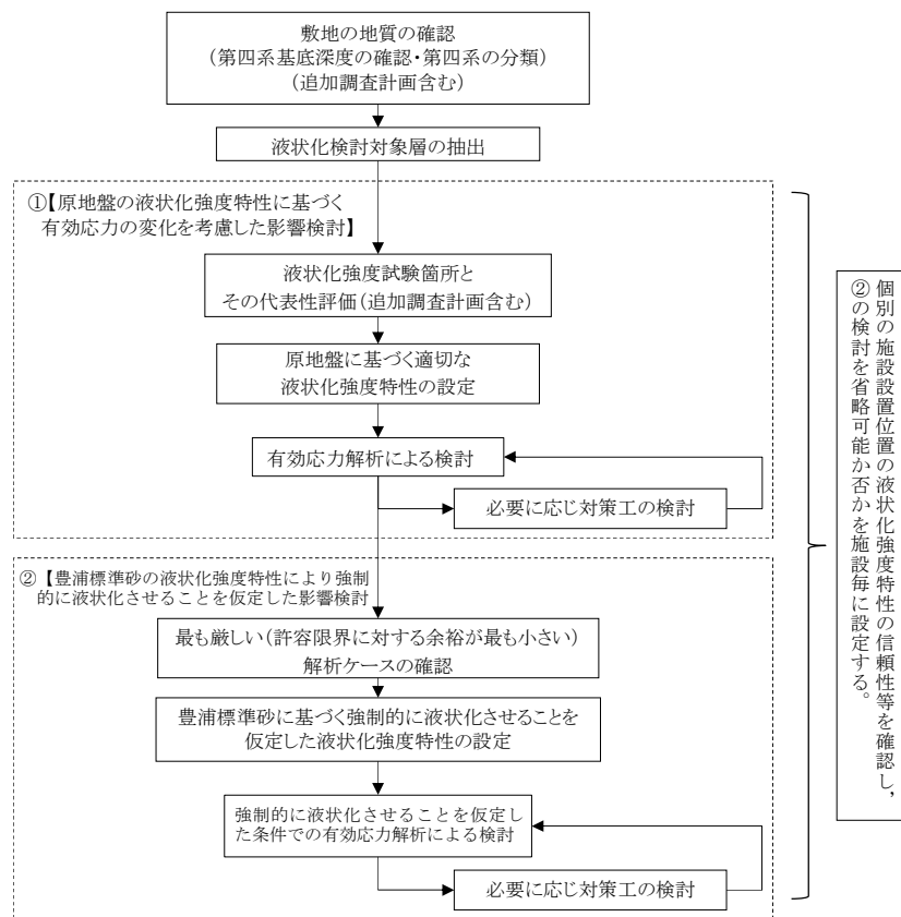
図 4.2-1 液化化影響評価のフロー
