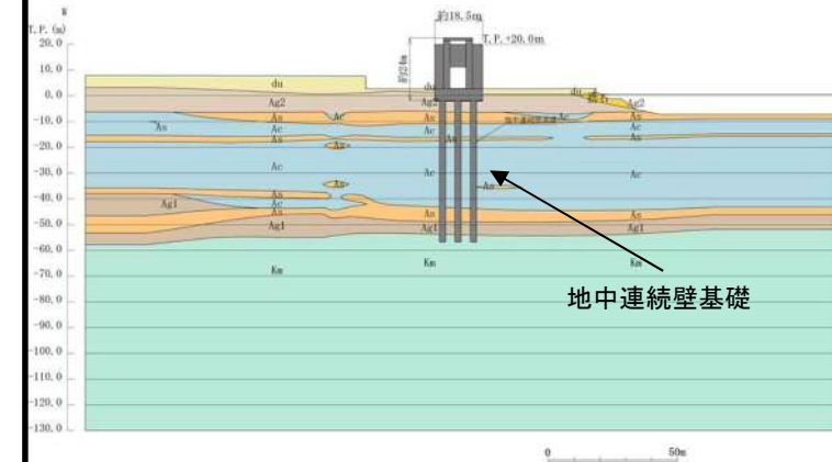
①-①断面
