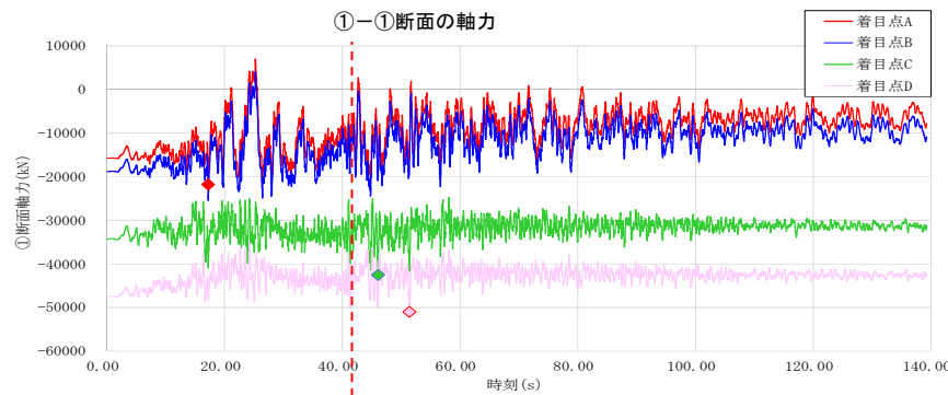
断面力時刻歴
