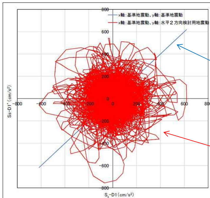
水平2方向検討用地震動の水平加速度振幅の軌跡図 (S s -D1)
