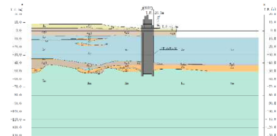
②-②断面
