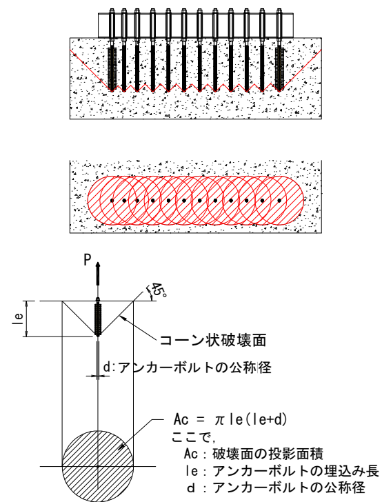
定着部コーン破壊照査における 有効水平投影面積
