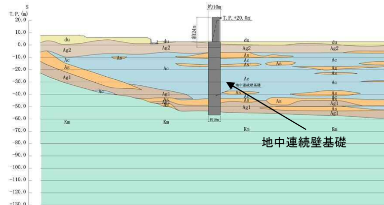
①-①断面
