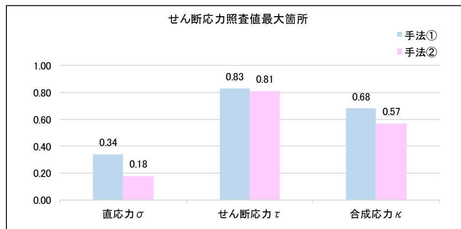
最大照査値比較
