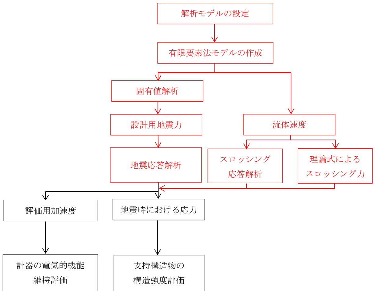
図 2-1 使用済燃料プール温度（S A）の耐震評価フロー
