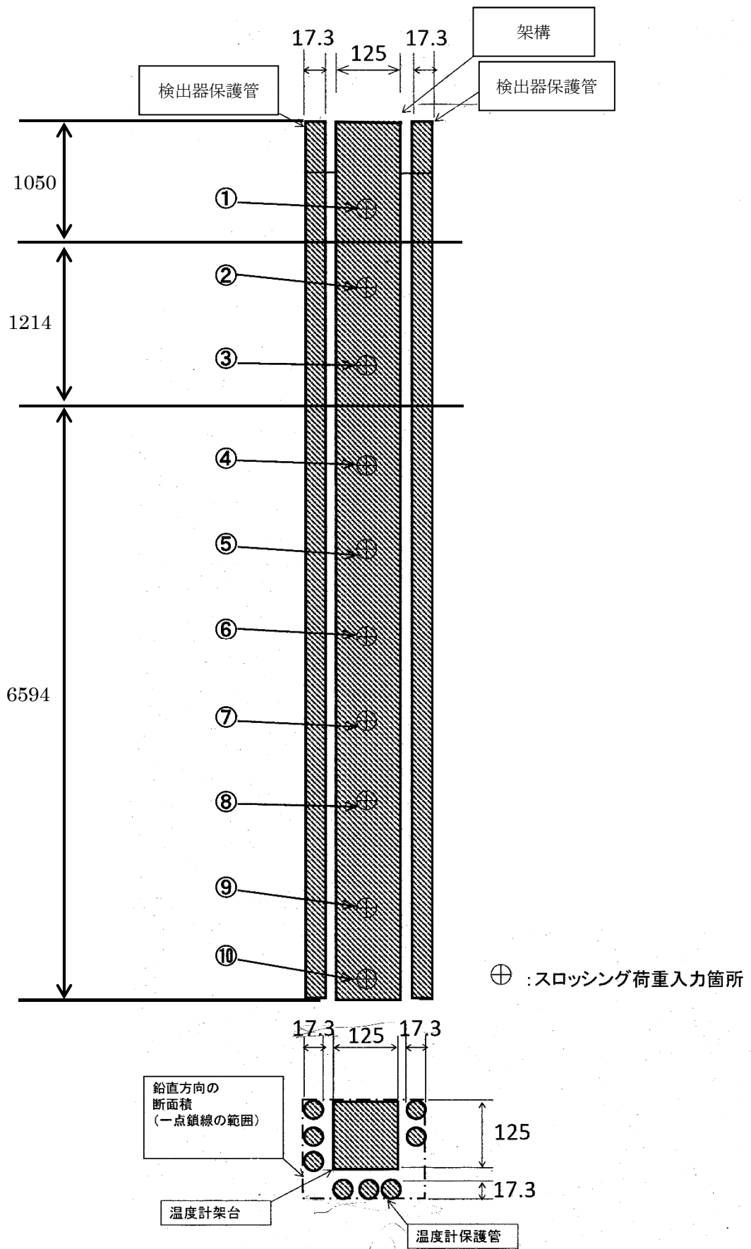
図 4-3 スロッシング評価モデル図
