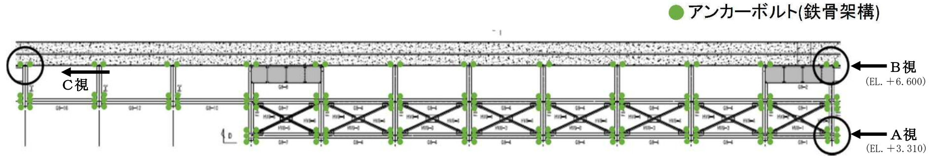
平面図
