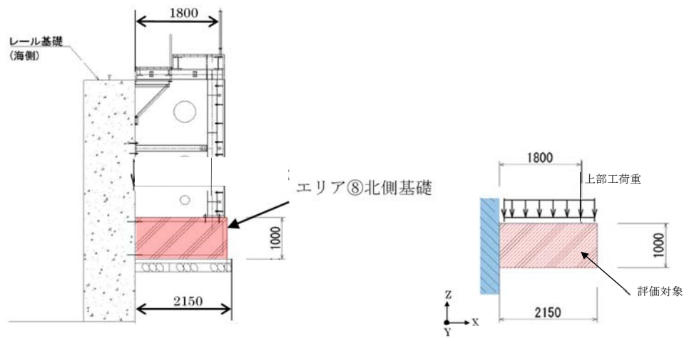
図 3-5 海水ポンプエリア防護壁の解析モデル図 (4/6)
