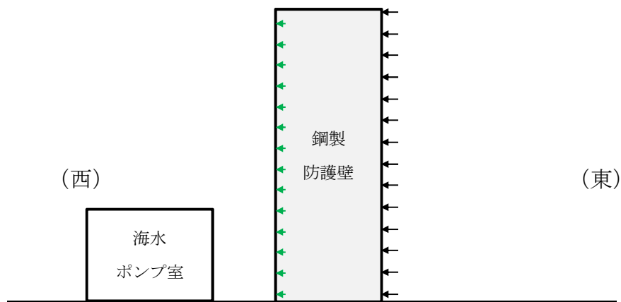
図4-3 風圧力による荷重 W_w の作用方法（鋼製防護壁）
