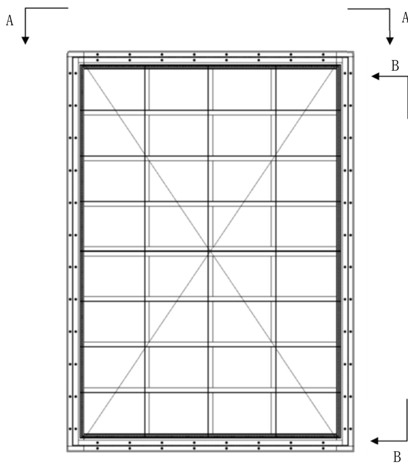
<扉立面図>
