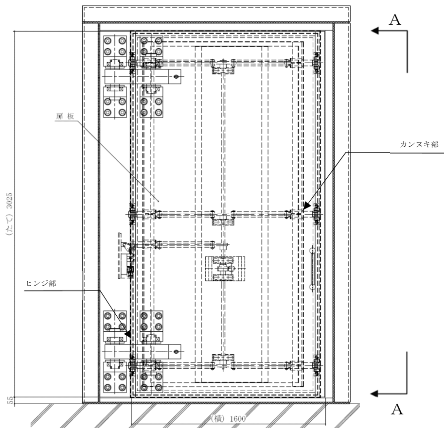
<扉立面図>
