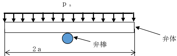
図 3-13 弁棒モデル図
