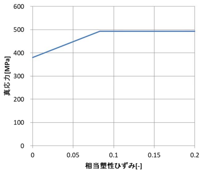
図3-5 真応力ー相当塑性ひずみ関係（鉄筋）
