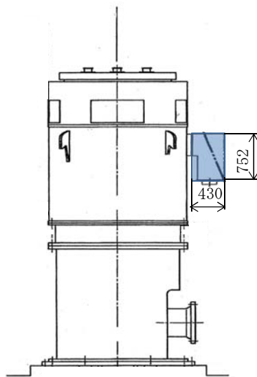
図3-17 一次側端子箱の受圧部図
