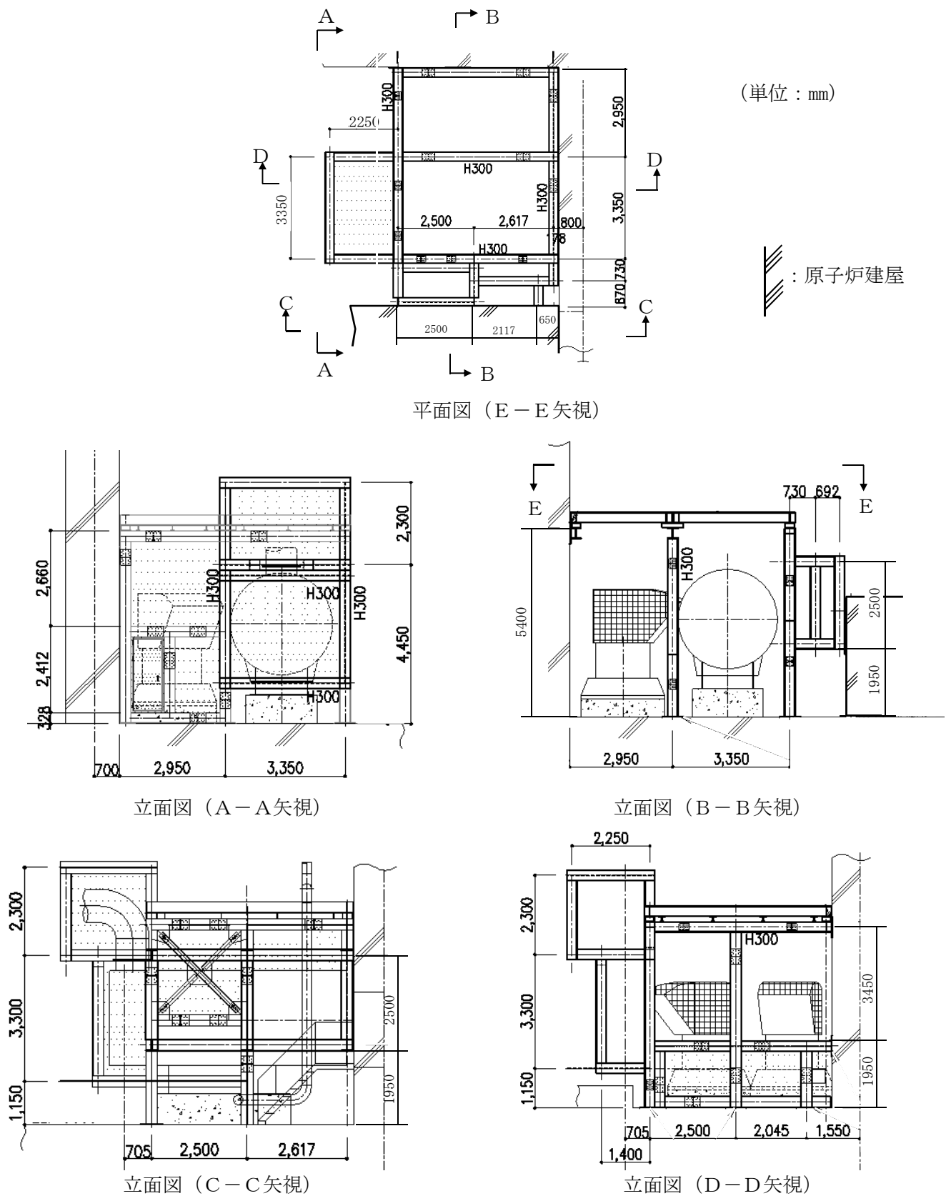
図 2-2 非常用ディーゼル発電機（高圧炉心スプレイ系ディーゼル発電機を含む。）室 ルーフベントファン防護対策施設架構の構造図(1/4) （2 C 非常用ディーゼル発電機室ルーフベントファン防護対策施設）
