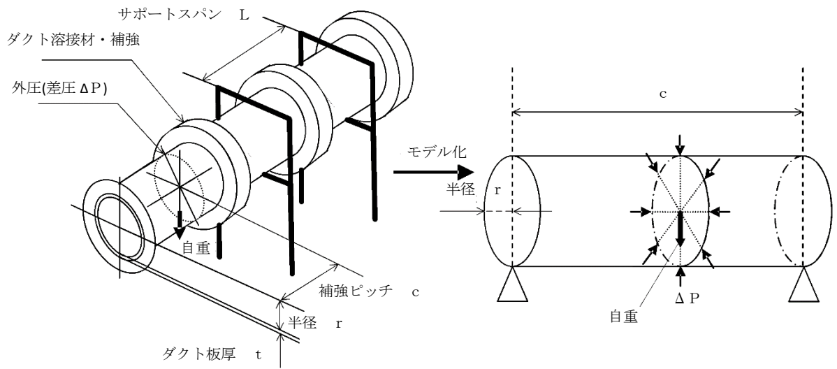
図5-20 丸ダクトモデル図
