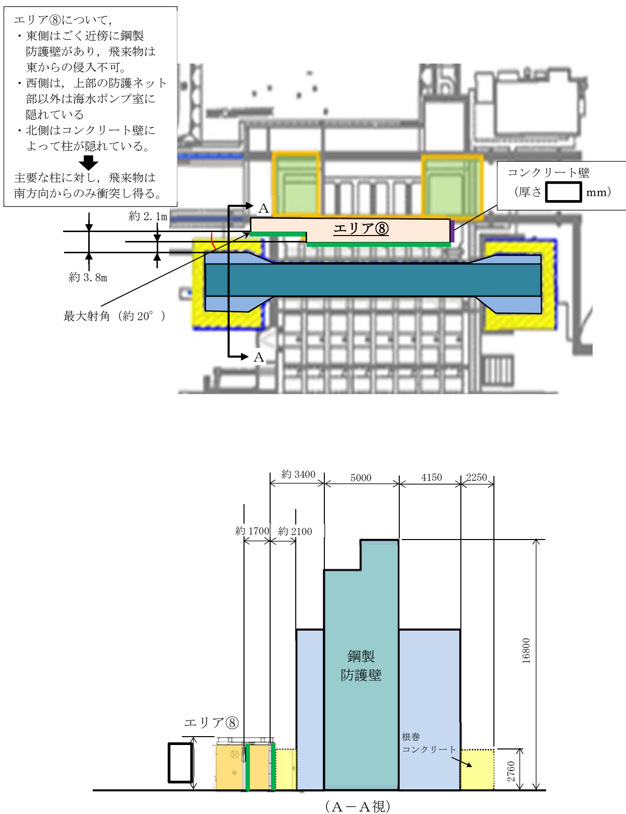
図 2-6 海水ポンプエリア防護対策施設防護鋼板の構造図 (3/3)
