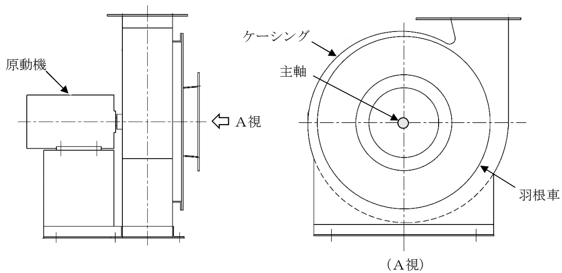
図 2-5 ファンの概要図（中央制御室換気系フィルタ系ファン）
