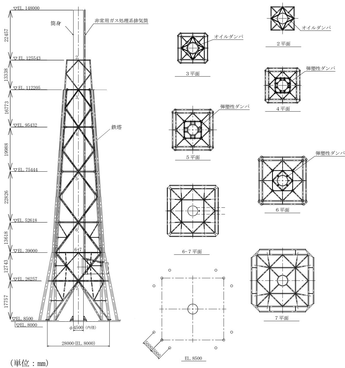
図 2-2 主排気筒概要図
