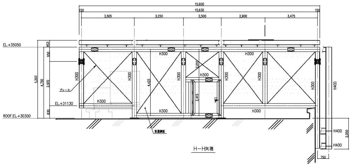
図 2-3 中央制御室換気系冷凍機防護対策施設架構の構造図(6/6)
