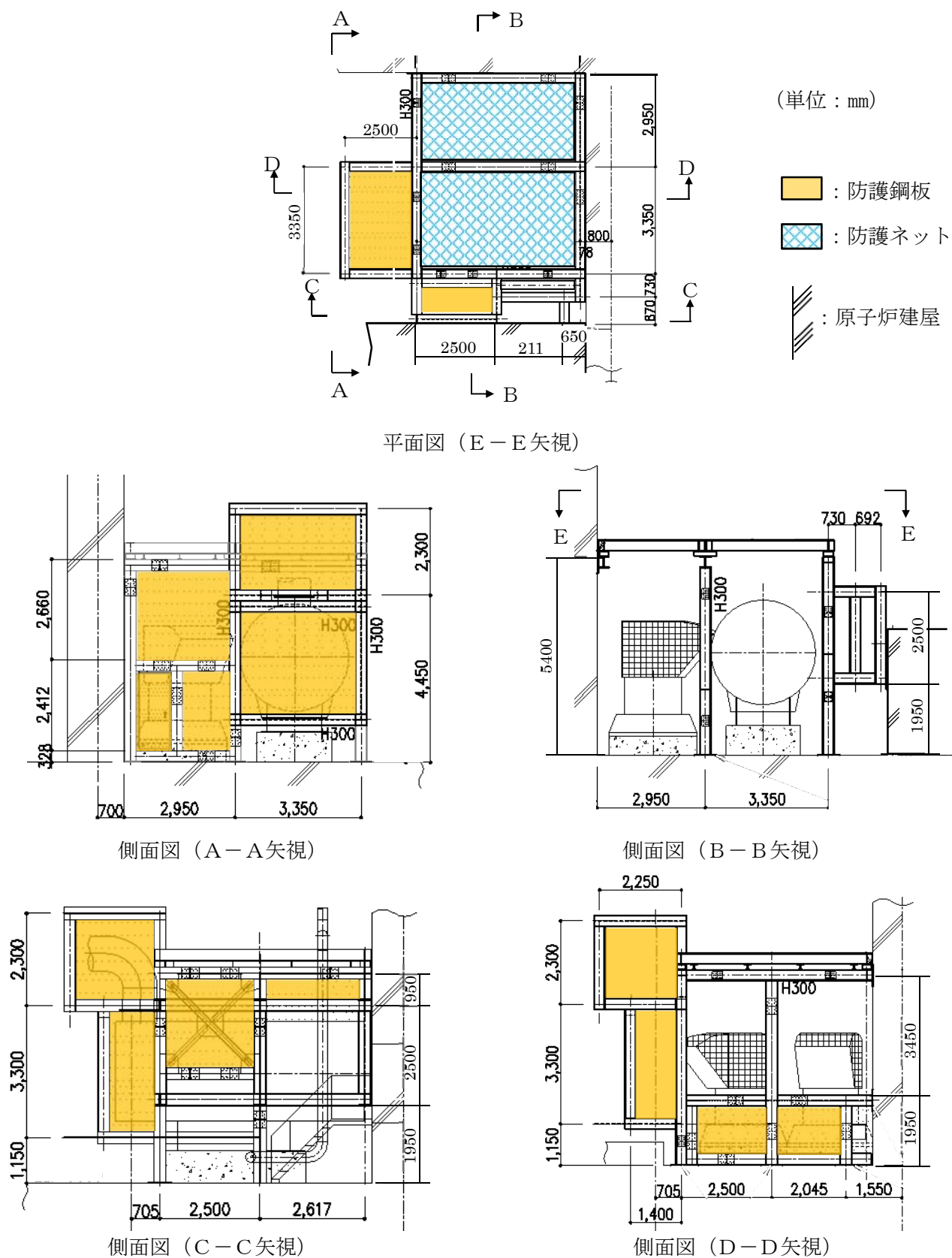
図 2-2 2 C 非常用ディーゼル発電機室ルーフベントファン防護対策施設防護鋼板の構造図 (1/2)
