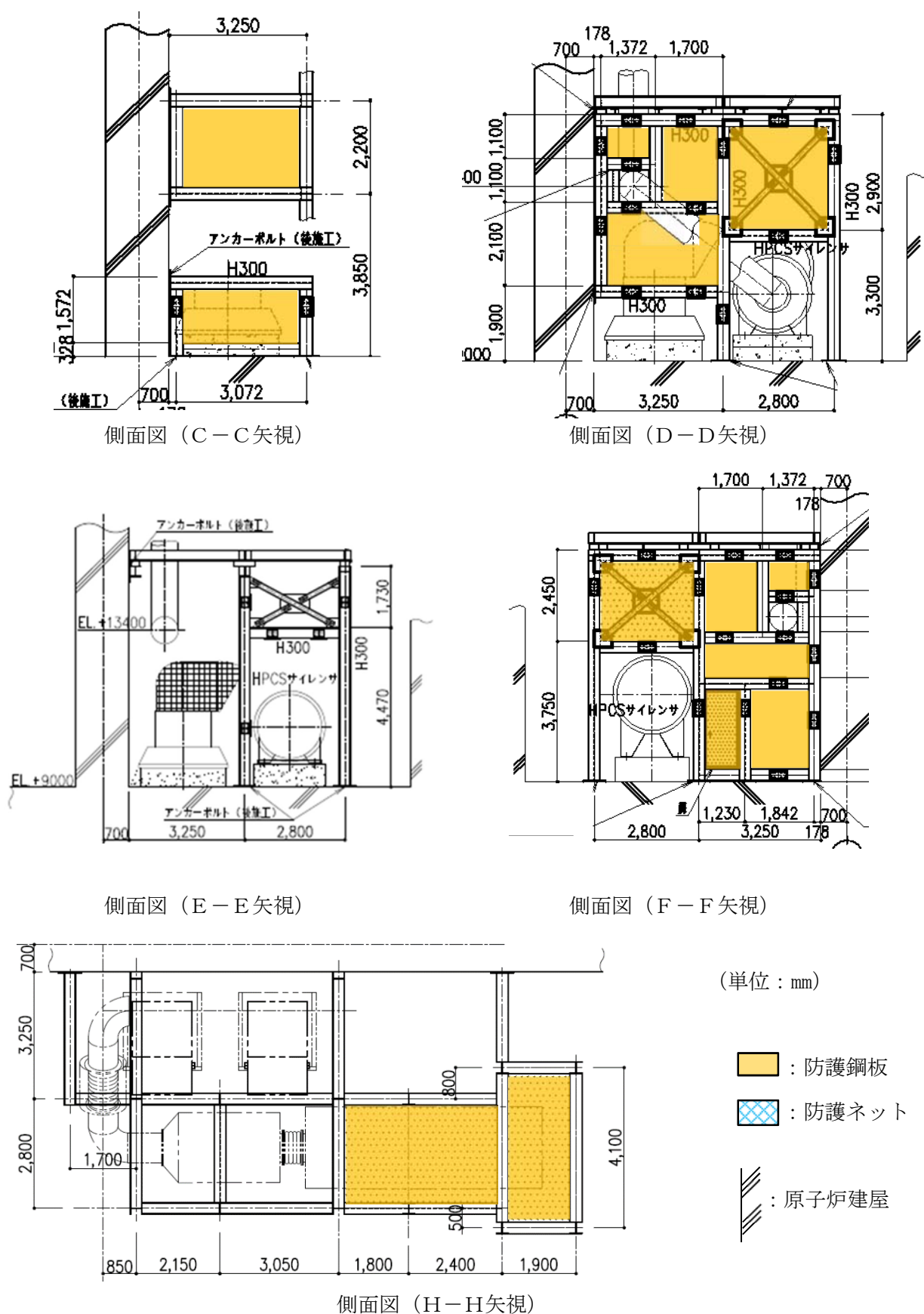
図 2-4 高圧炉心スプレイ系ディーゼル発電機室ルーフベントファン防護対策施設防護鋼板の構造図 (2/3)
