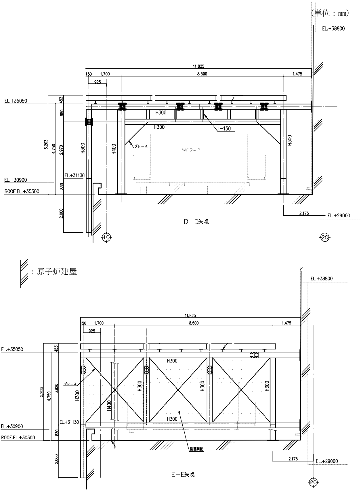
図 2-3 中央制御室換気系冷凍機防護対策施設架構の構造図(4/6)
