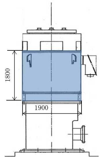
図3-16 原動機フレームの受圧部図
