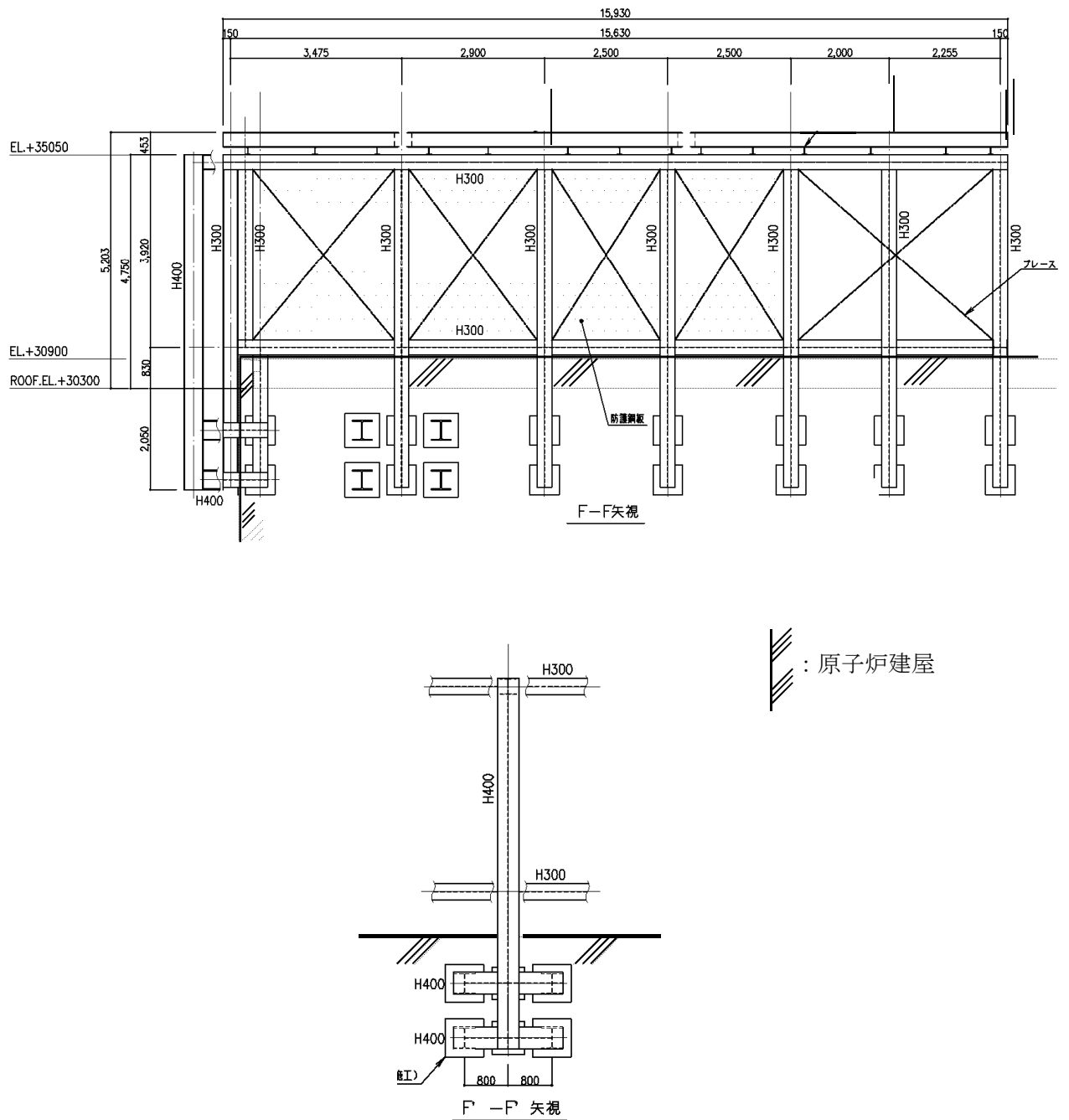
図 2-3 中央制御室換気系冷凍機防護対策施設架構の構造図 (5/6)
