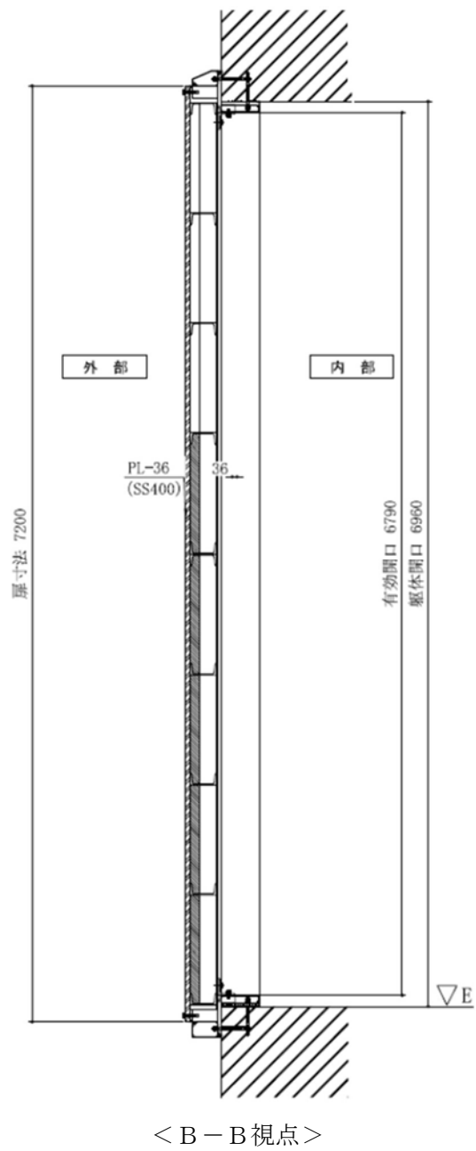
図2-17 原子炉建屋付属棟2階東側機器搬入口扉の構造図 (2/2)
