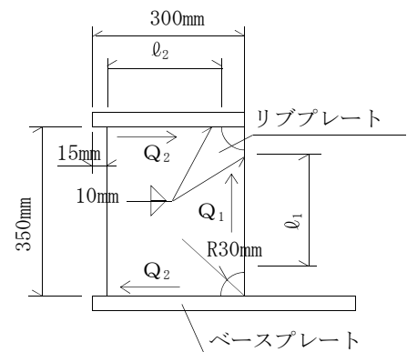
図 5-9 溶接位置図
