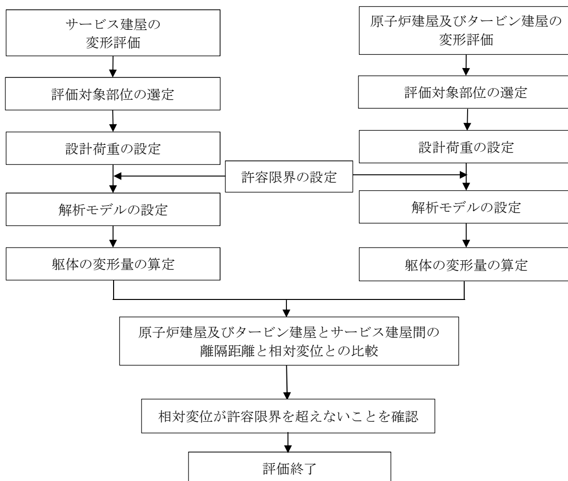
図2-7 サービス建屋の波及的影響評価フロー
