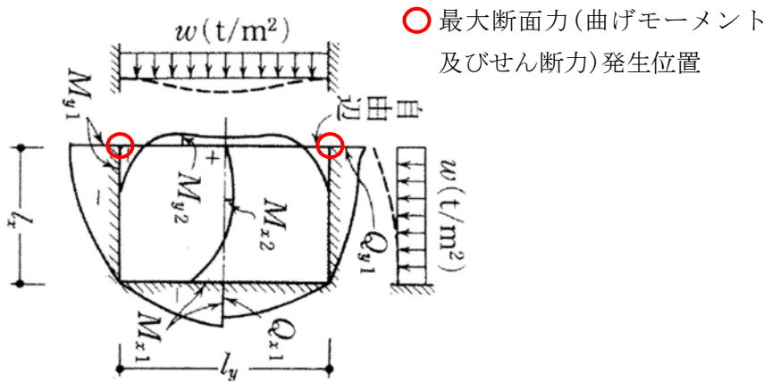
図3-6 3辺固定スラブモデルに発生する断面力の理論モデル及び算出式
