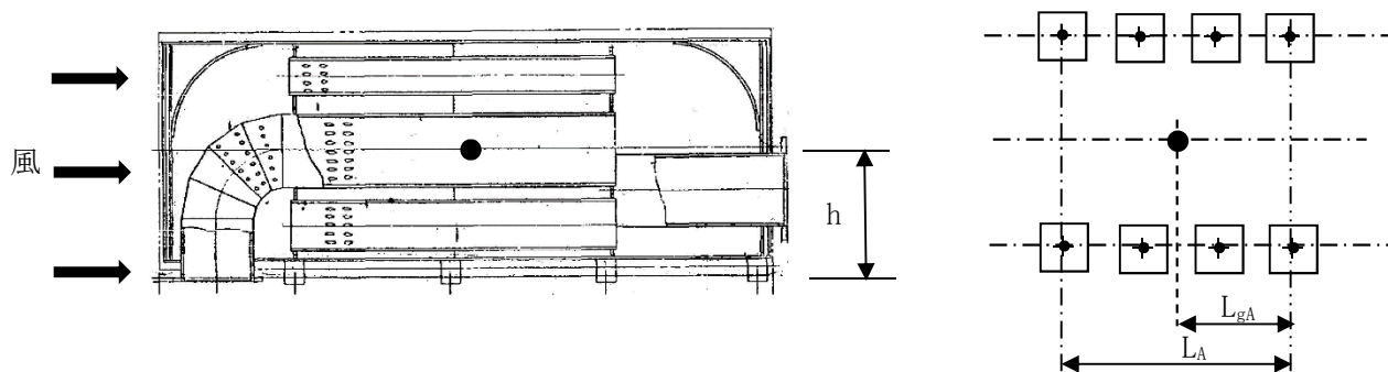
図 5-13(2/2) 非常用ディーゼル発電機 2D 排気消音器，高圧炉心スプレイ系ディーゼル 発電機排気消音器の評価モデル図（フィルタ部軸方向）
