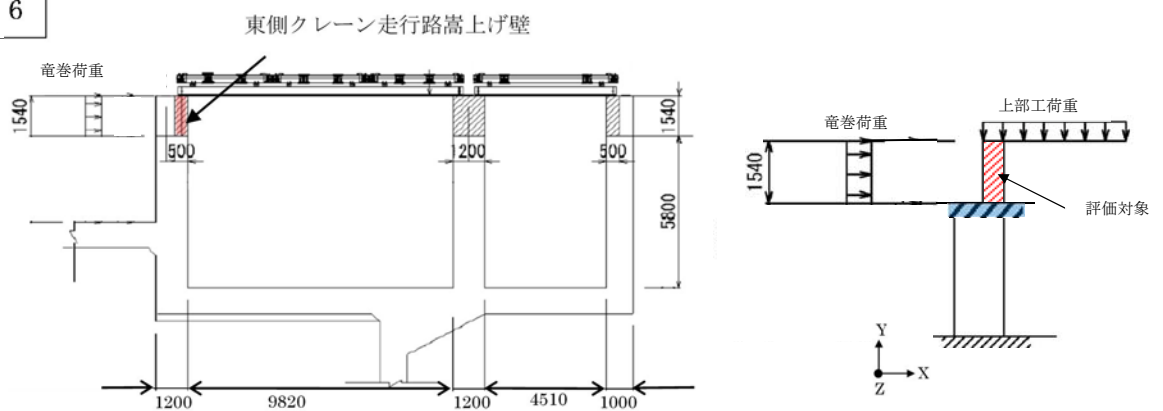
図3-5 海水ポンプエリア防護壁の解析モデル図 (2/6)
