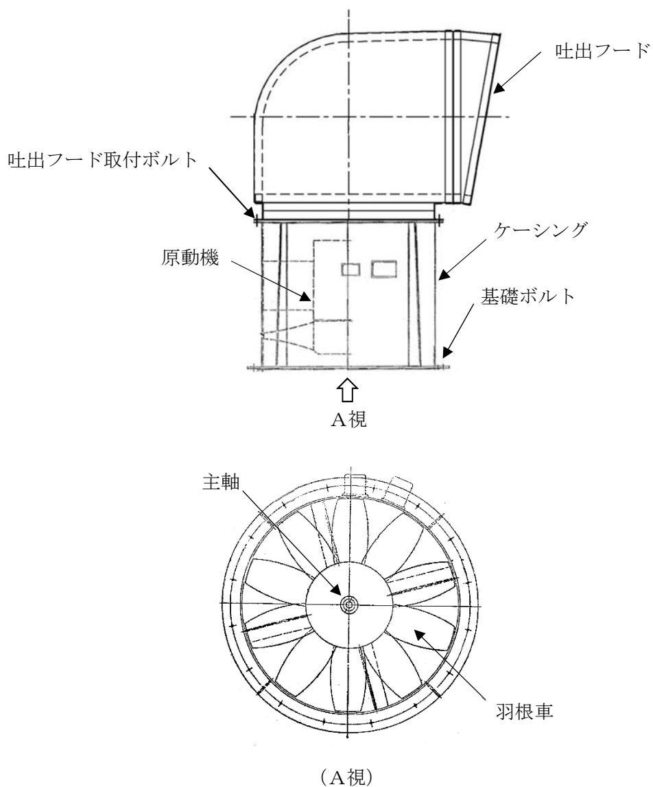
図 2-6 ファンの概要図（ディーゼル発電機室ルーフベントファン）
