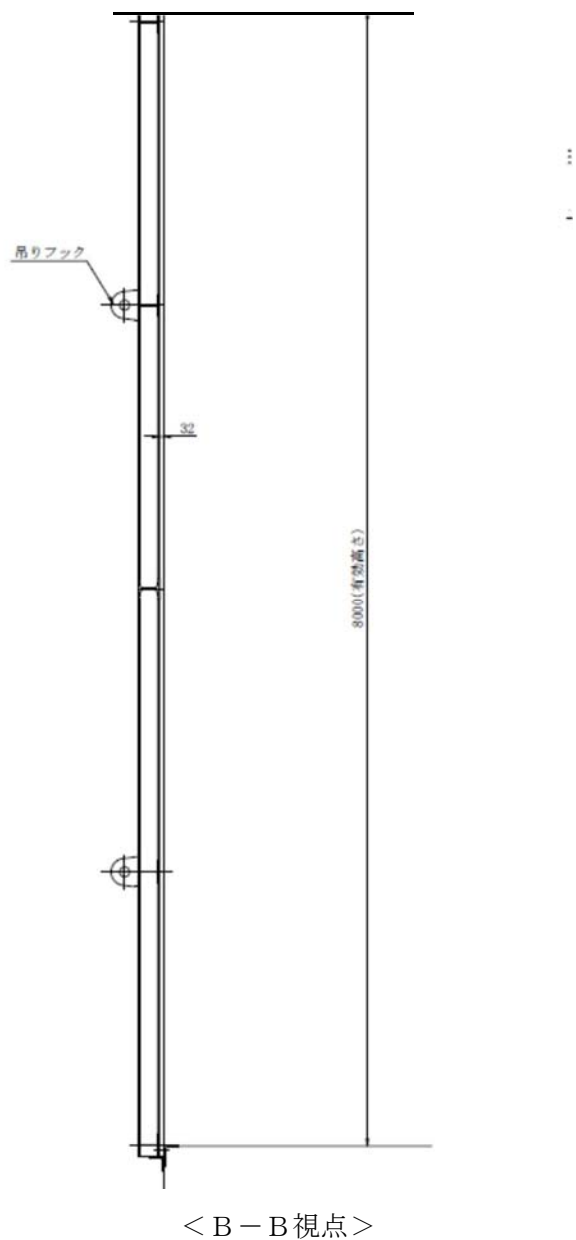
図2-22 原子炉付属棟4階南東側機器搬入口扉の構造図 (2/2)
