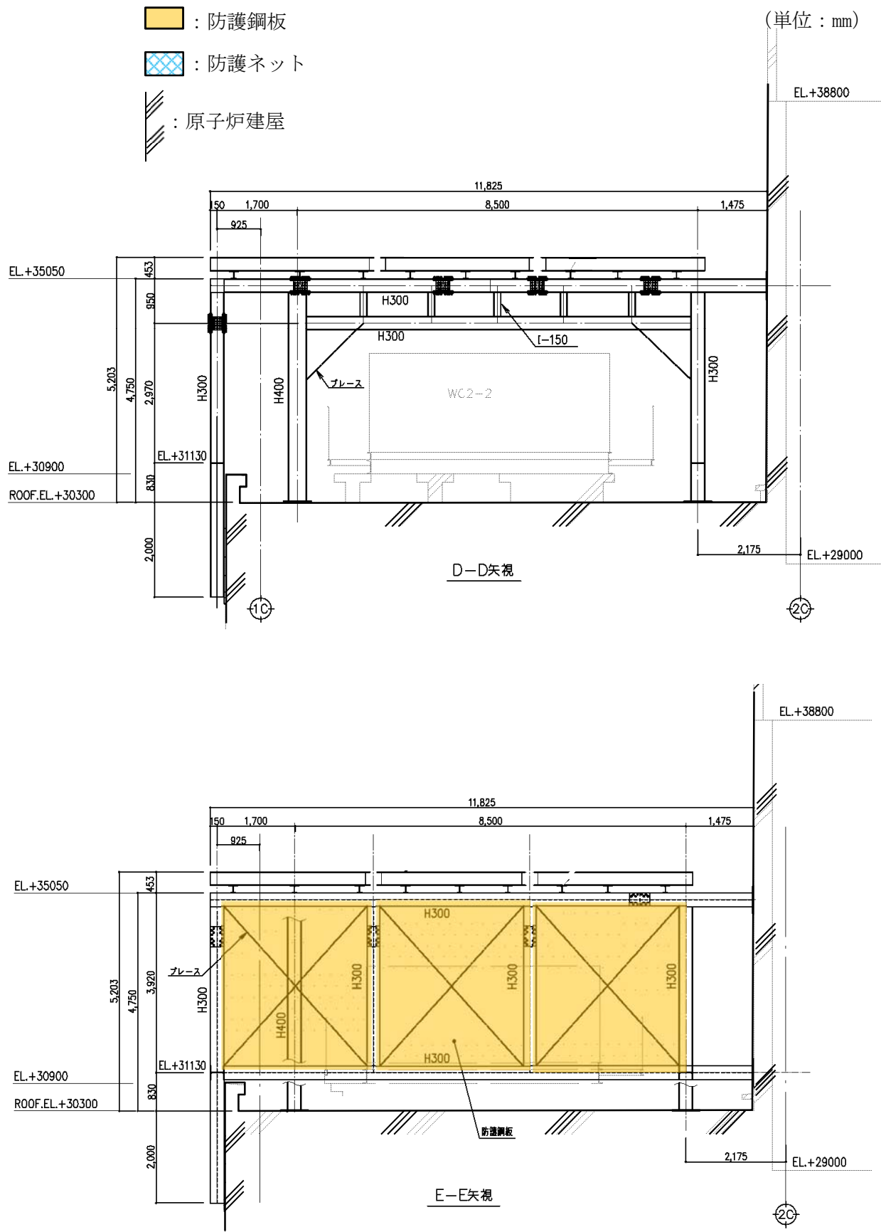
図 2-5 中央制御室換気系冷凍機防護対策施設防護鋼板の構造図(4/6)
