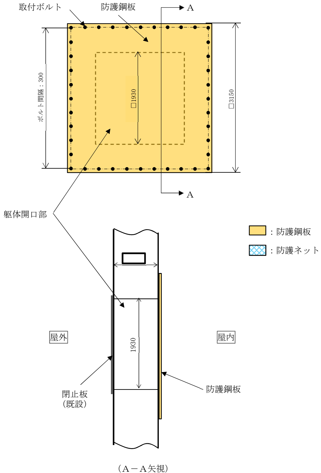
図 2-8 原子炉建屋付属棟開口閉鎖部防護対策施設防護鋼板の構造図
