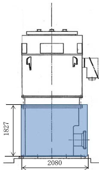
図3-15 原動機台の受圧部図
