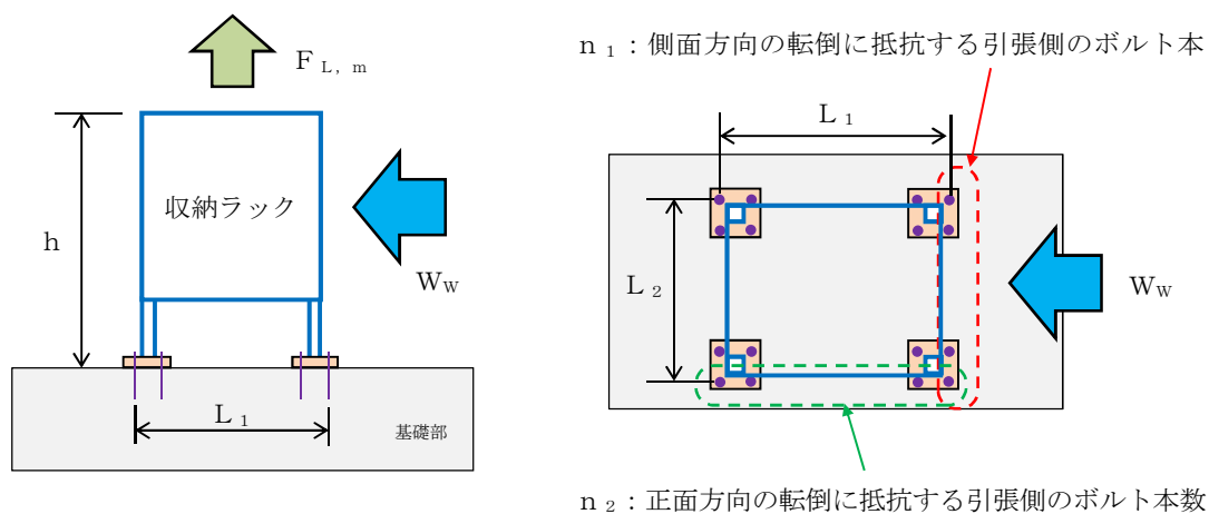
図 6-10 収納ラックの計算モデル図
