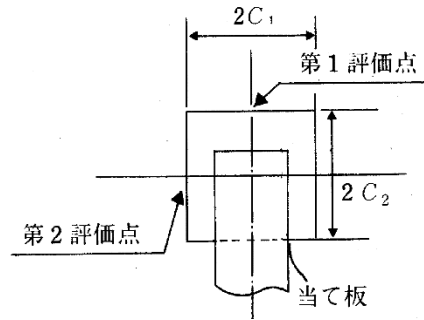
図 3-5 胴の評価点
