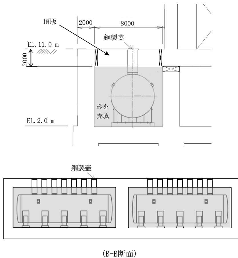
図2-28 軽油貯蔵タンクタンク室の概略断面図
