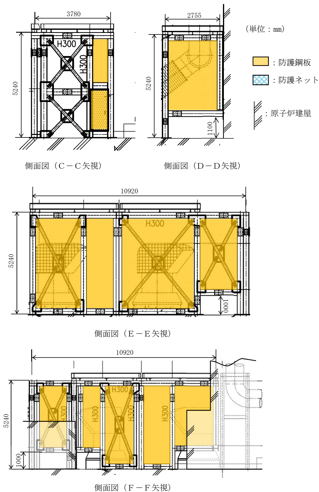
図 2-3 2D 非常用ディーゼル発電機室ルーフベントファン防護対策施設防護鋼板の構造図 (2/2)
