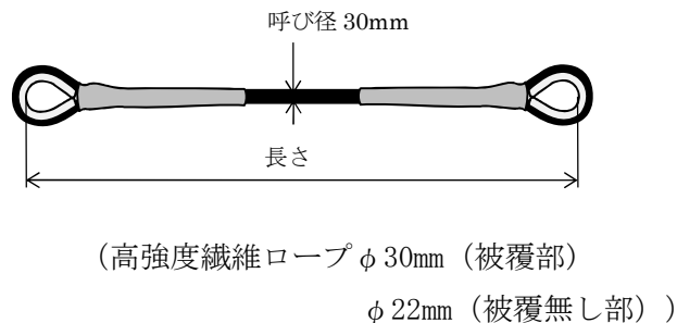
図 3-1 連結材の評価対象部位
