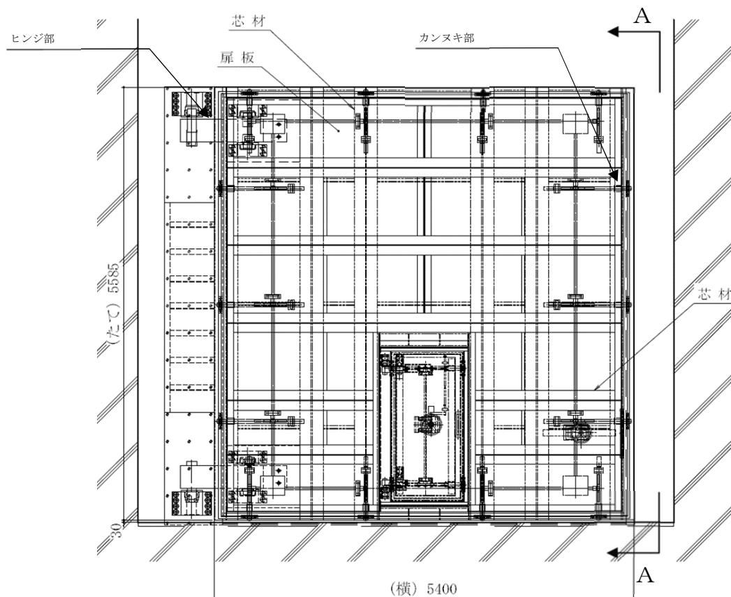
<扉立面図>
