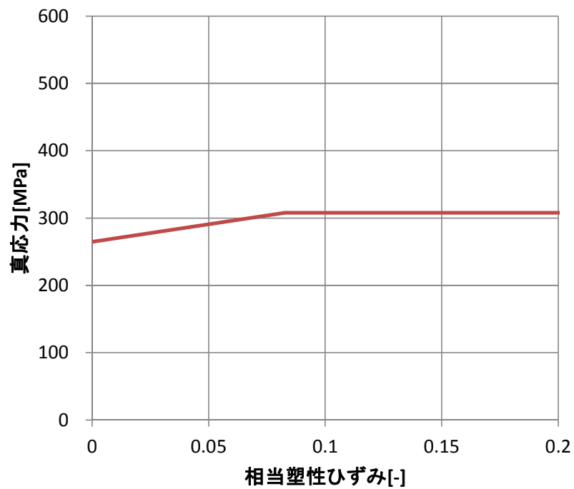
図3-6 真応力ー相当塑性ひずみ関係（デッキプレート）
