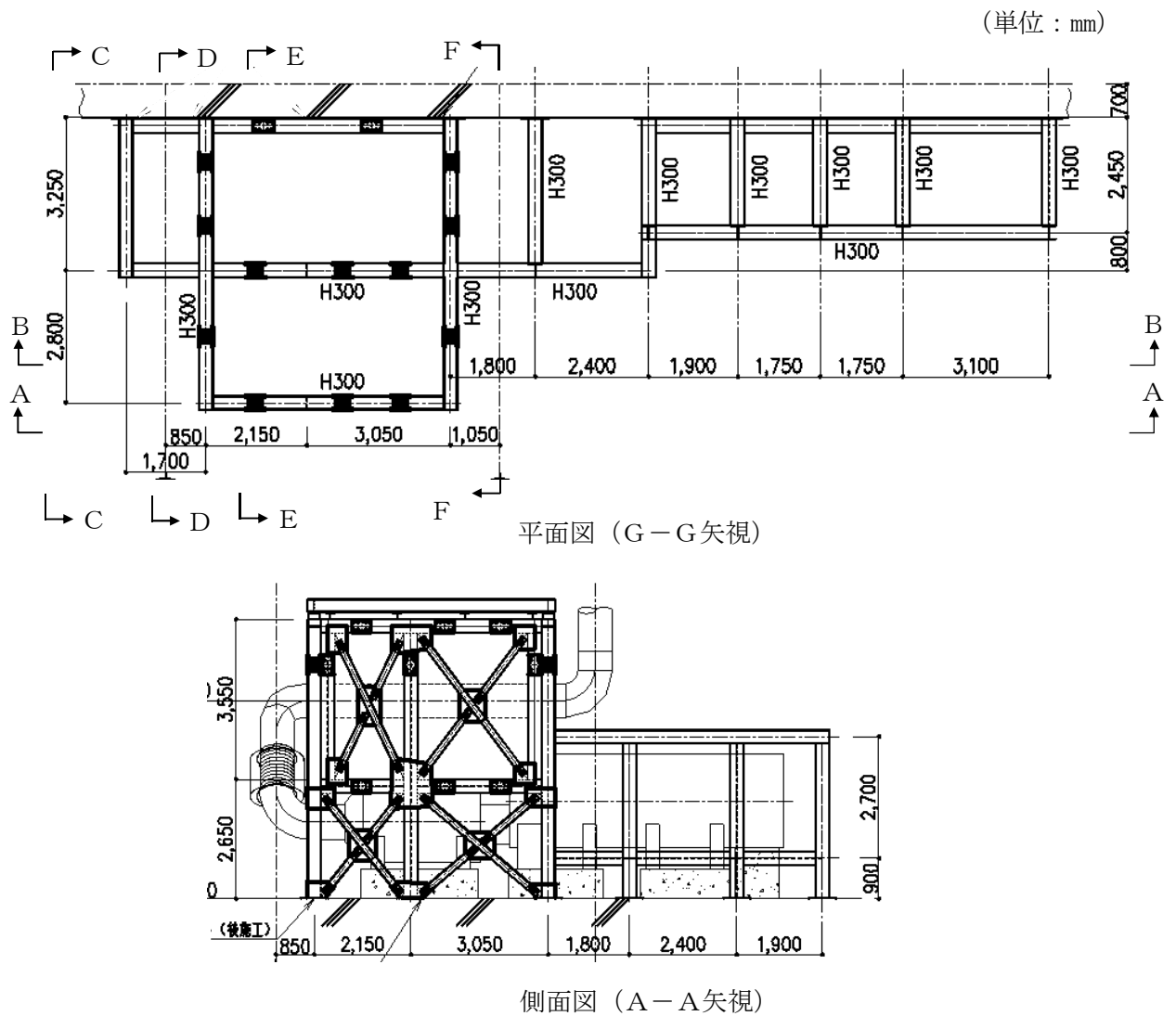
図 2-2 非常用ディーゼル発電機（高圧炉心スプレイ系ディーゼル発電機を含む。）室 ルーフベントファン防護対策施設架構の構造図(4/7) （高圧炉心スプレイ系ディーゼル発電機室ルーフベントファン防護対策施設(1/4)）
