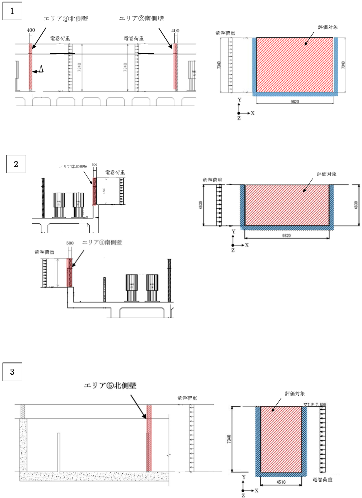
図3-5 海水ポンプエリア防護壁の解析モデル図 (1/6)
