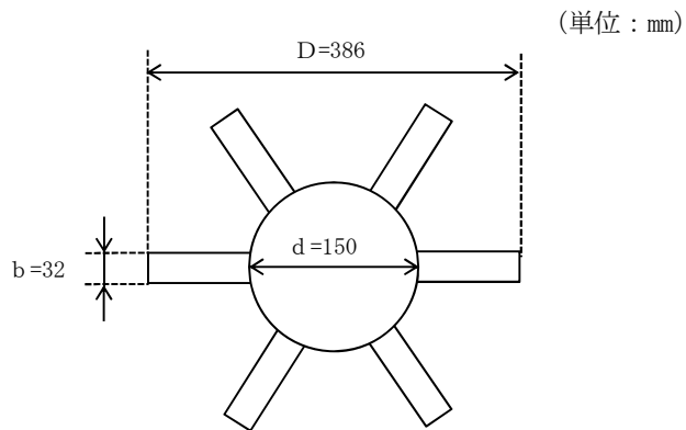
図3-22 回転子（原動機部）の断面図
