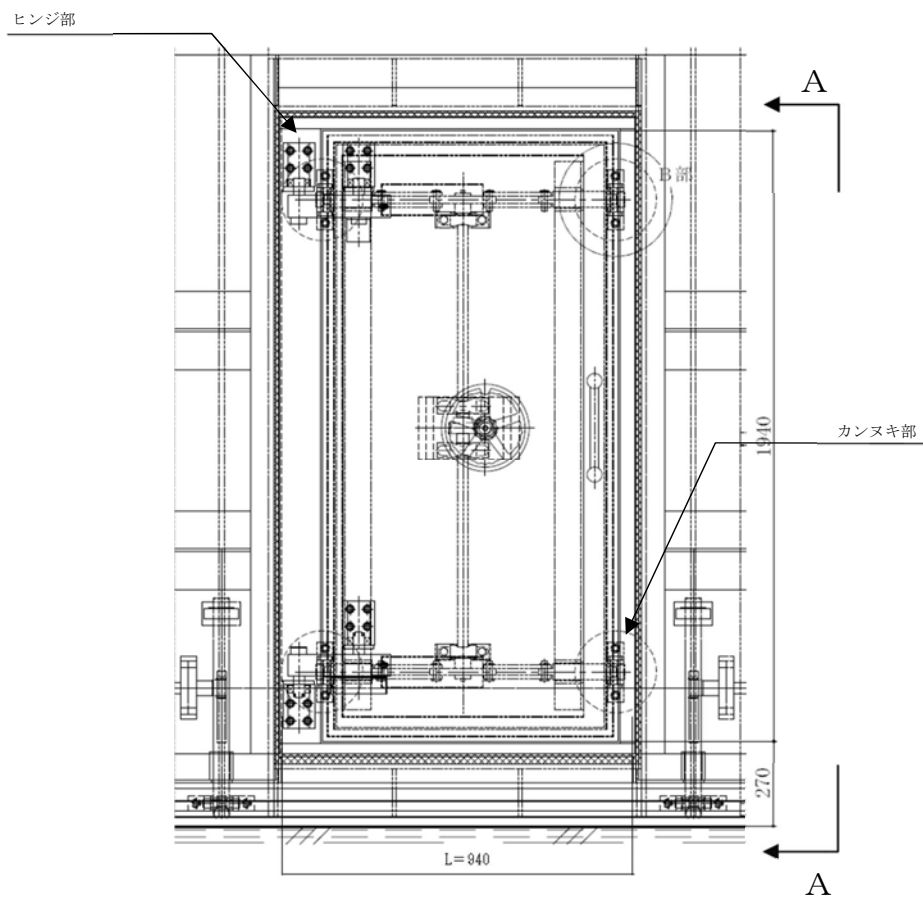
<扉立面図>
