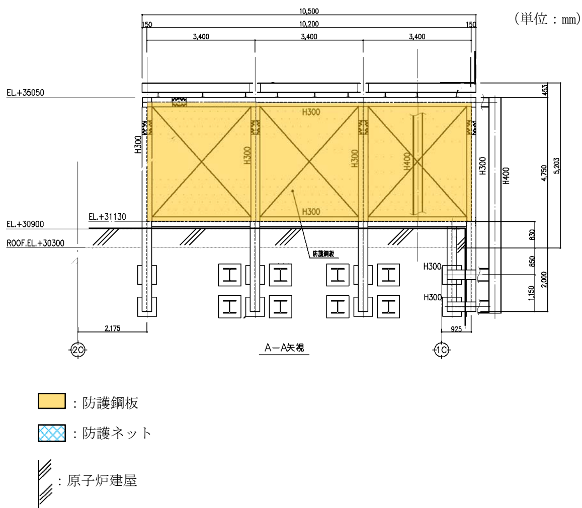
図 2-5 中央制御室換気系冷凍機防護対策施設防護鋼板の構造図(2/6)
