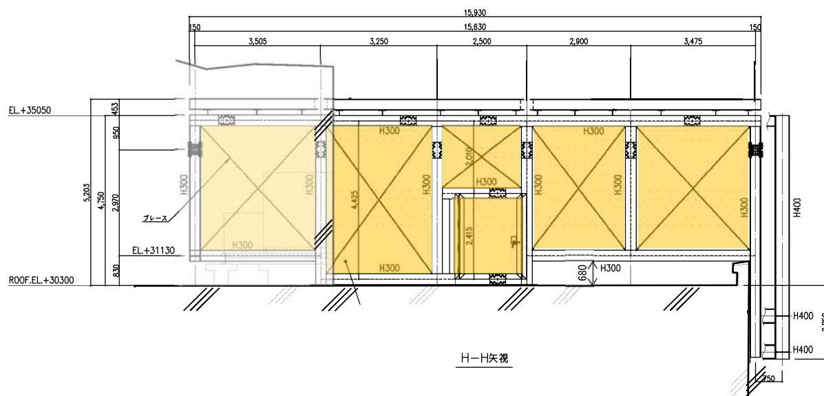
図 2-5 防護ネットの割付展開図(3/3)
