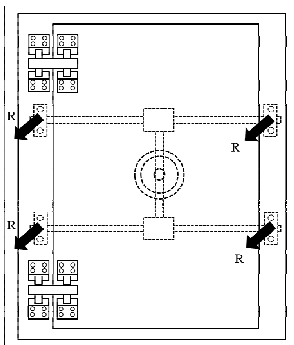
<扉立面図>
