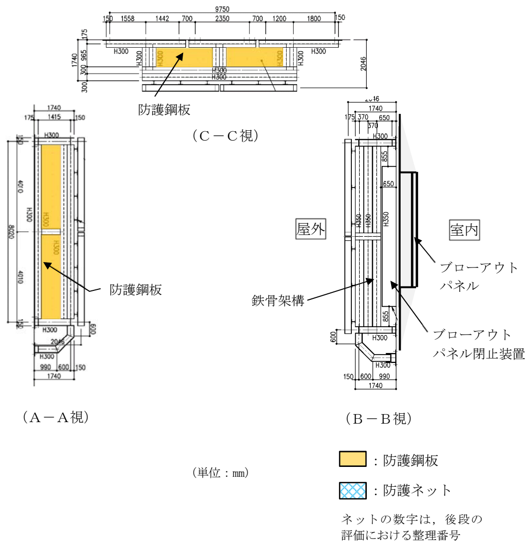
図 2-7 防護ネットの割付展開図 (原子炉建屋外側ブローアウトパネル防護対策施設) (2/2)
