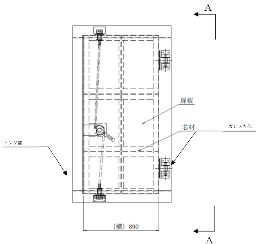
<扉立面図>
