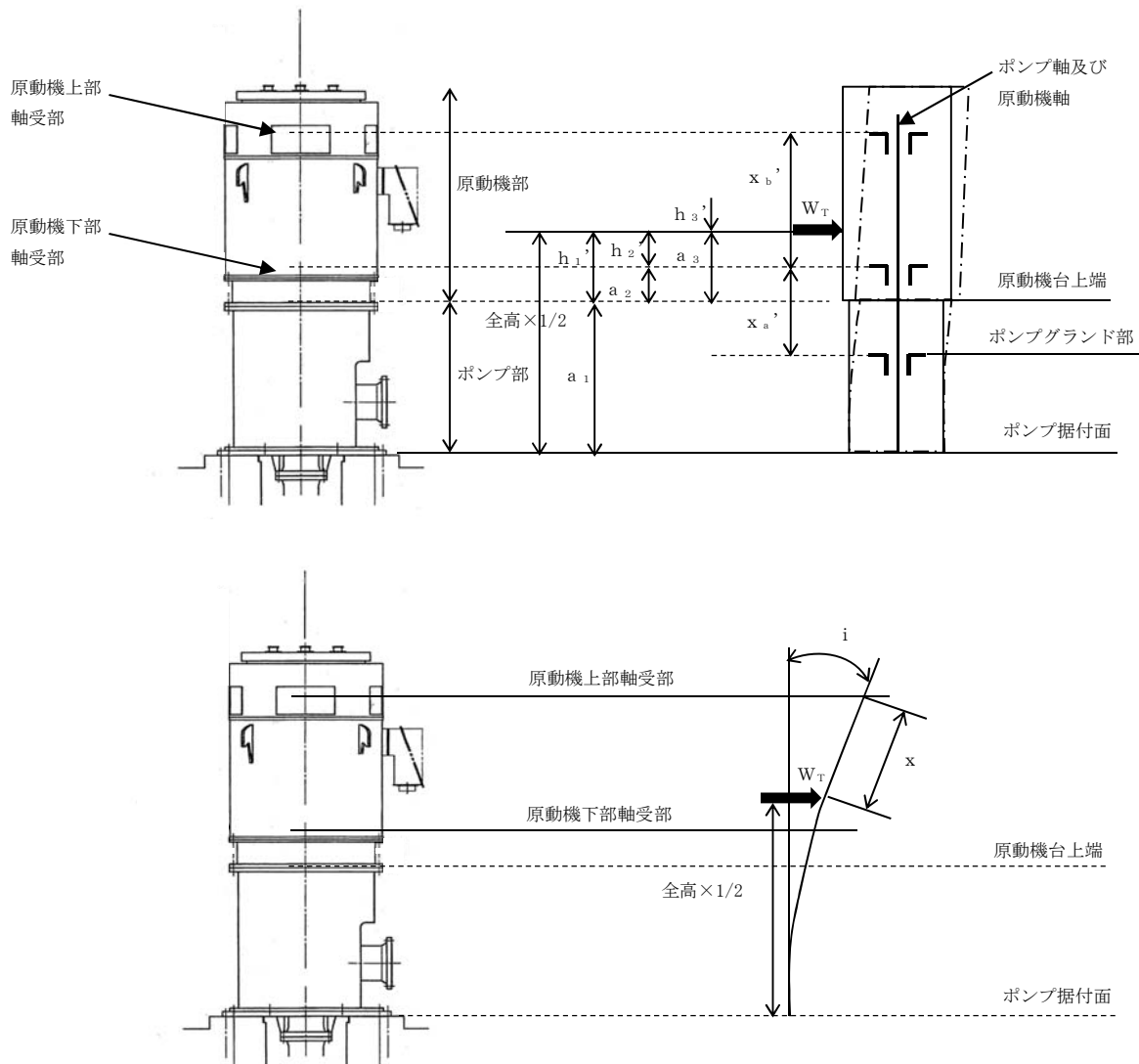
図 3-7 残留熱除去系海水系ポンプのたわみ量計算モデル図
