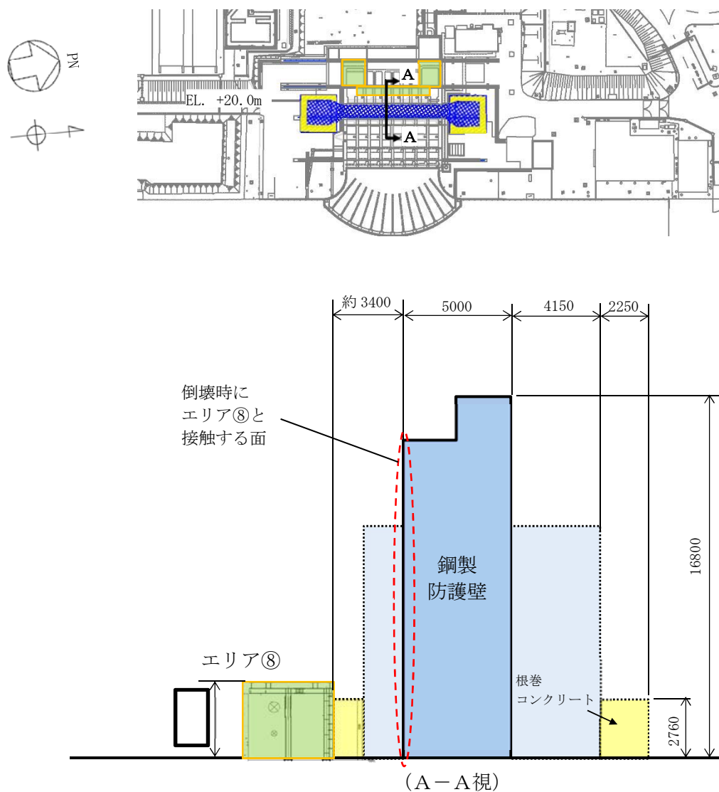
図 3-3 鋼製防護壁と防護対象の位置関係
