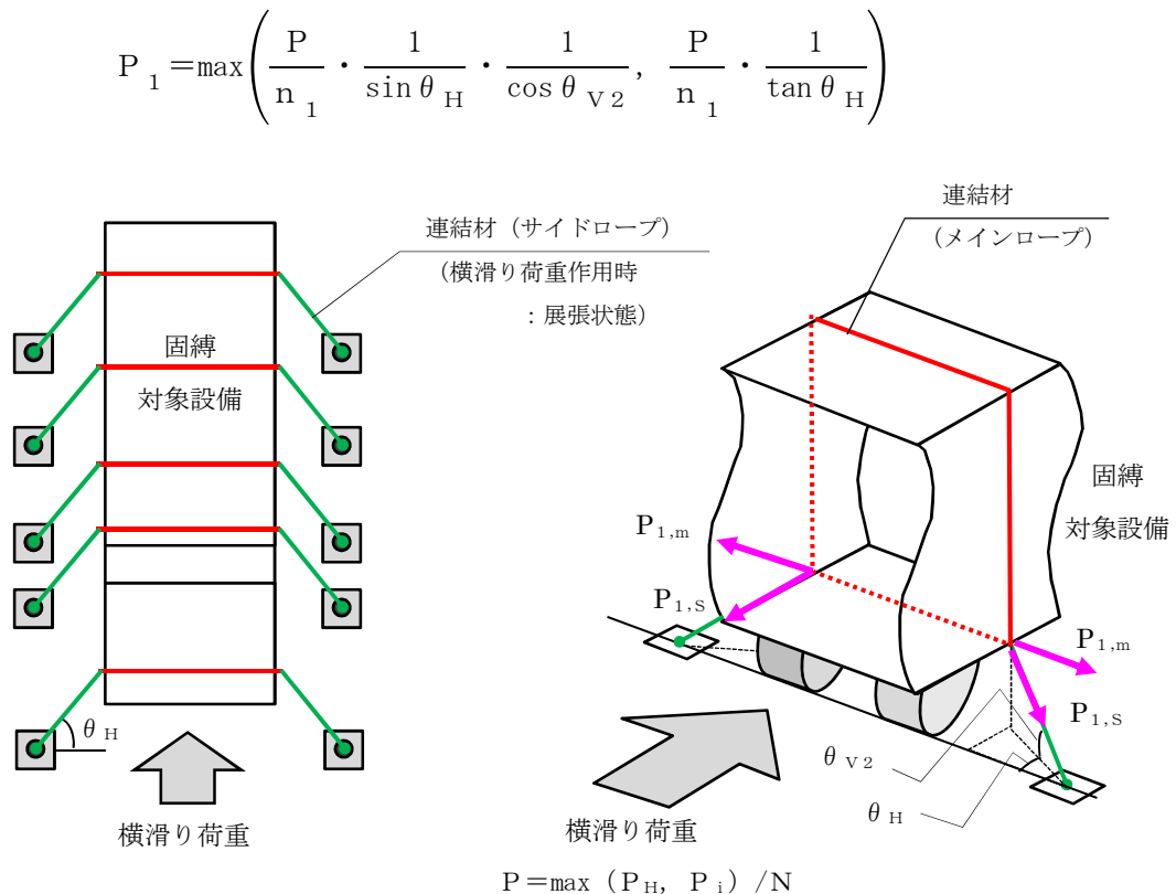
図 6-5 横滑り時（正面方向）の連結材の評価モデルの概要図
