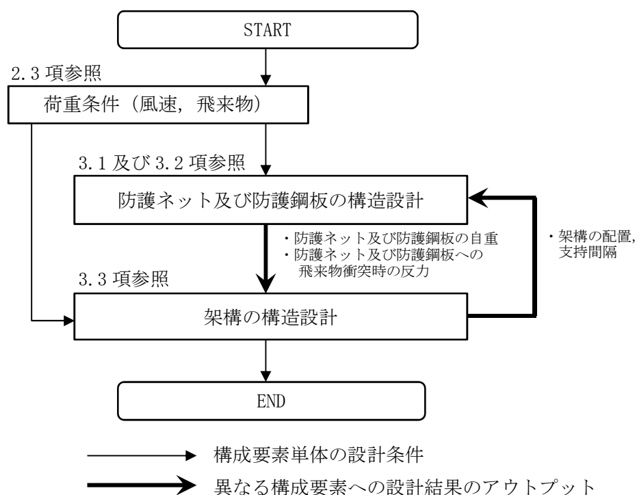
図 3-1 防護対策施設の設計フロー
