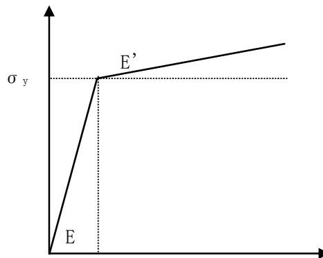
図 3-2 バイリニア型応力-ひずみ関係の概念図
