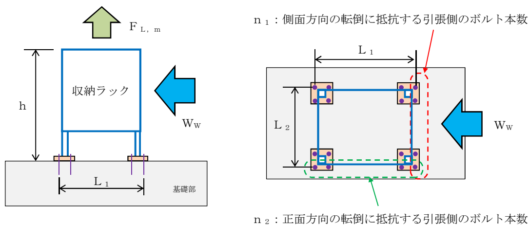
図 3-11 収納ラックの計算モデル図
