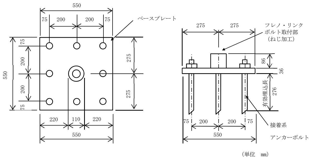
図 3-3 固定材（アンカープレート）及び基礎部（アンカーボルト）の評価対象部位
