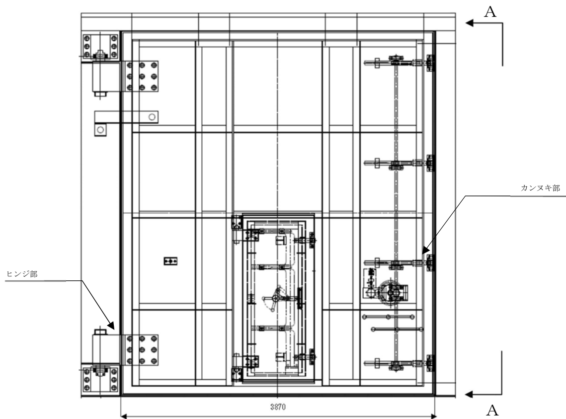
<扉立面図>
