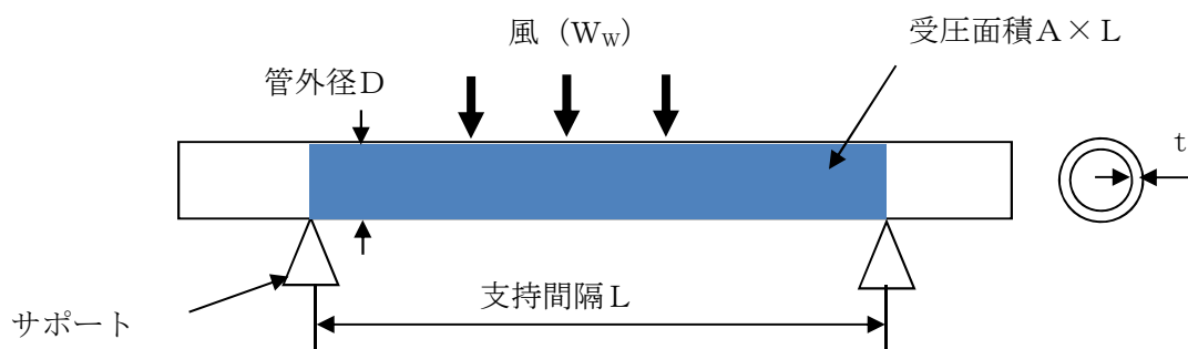
図 5-17 配管モデル図（両端支持形状）
