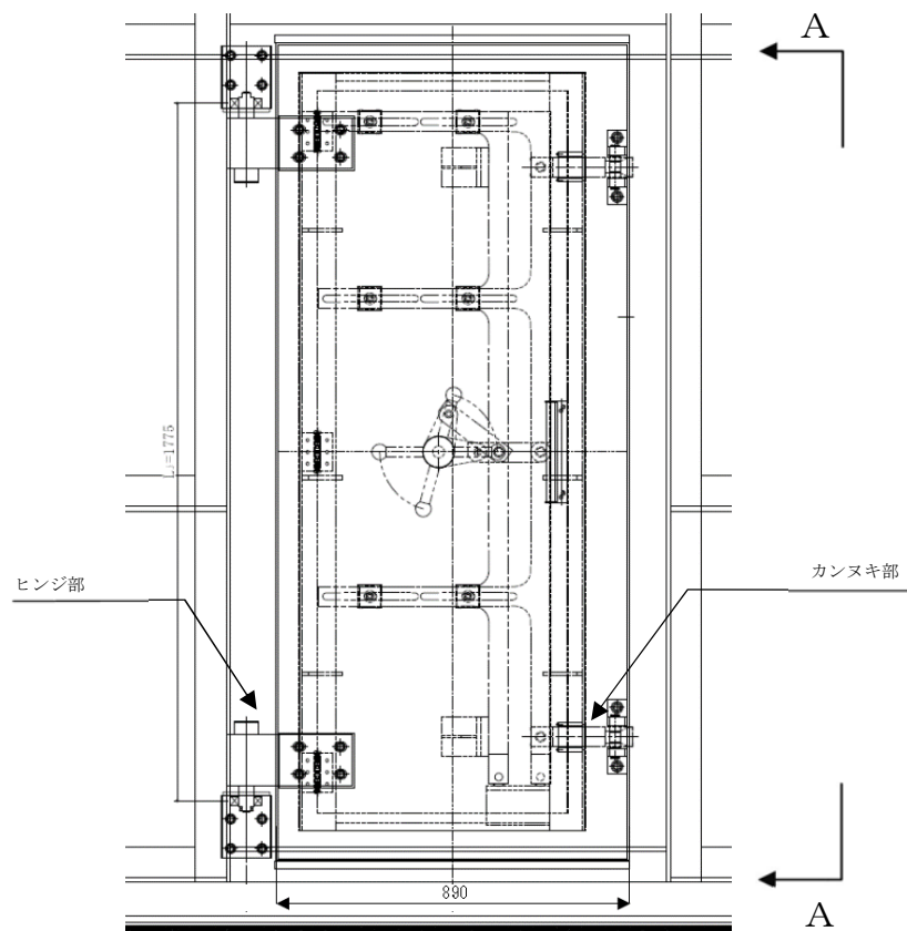
<扉立面図>
