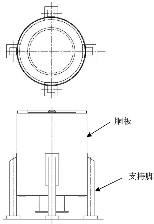
図2-2 ディーゼル発電機吸気口の概要図
