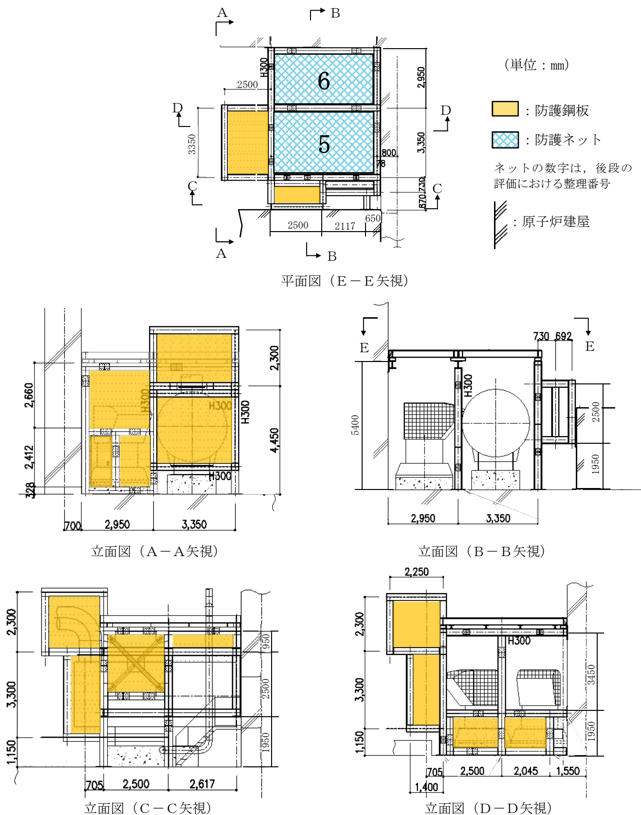
図 2-2 防護ネットの割付展開図 (2 C 非常用ディーゼル発電機室ルーフベントファン防護対策施設)
