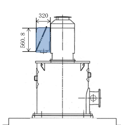
図3-17 主回路用端子箱の受圧部図
