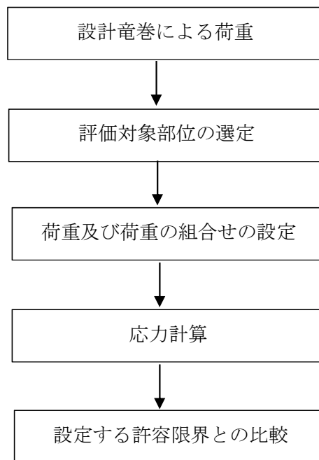
図2-5 ディーゼル発電機付属排気配管及びベント配管，残留熱除去系海水配管（放出側）並びにディーゼル発電機海水配管（放出側）の構造強度評価フロー
