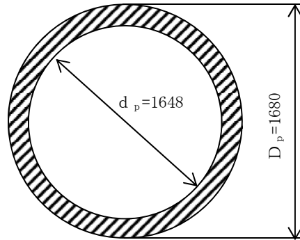
図3-20 原動機台の断面図
