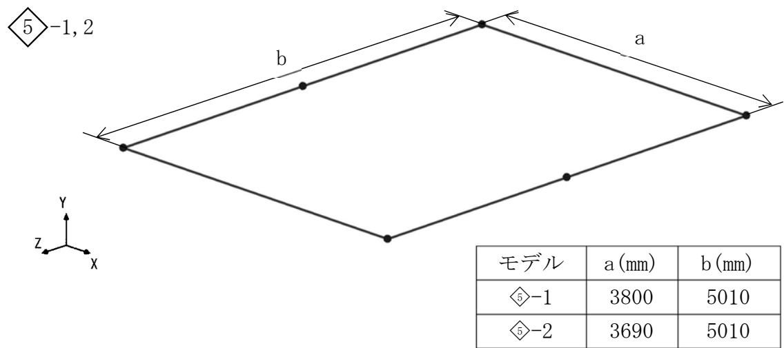
図3-5 海水ポンプエリア防護壁の解析モデル図 (5/6)
