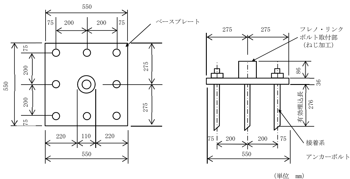
図 2-6 固定材（アンカープレート）及び基礎部（アンカーボルト）の概要図
