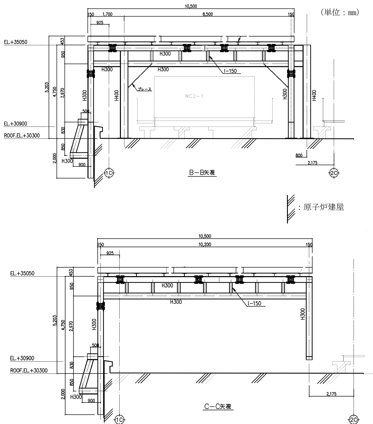
図 2-3 中央制御室換気系冷凍機防護対策施設架構の構造図(3/6)
