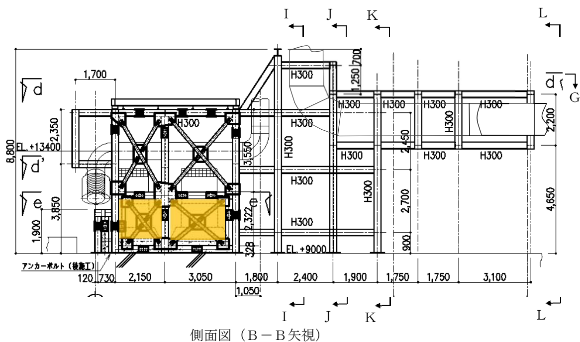
図 2-4 高圧炉心スプレイ系ディーゼル発電機室ルーフバントファン防護対策施設防護鋼板の構造図 (1/3)
