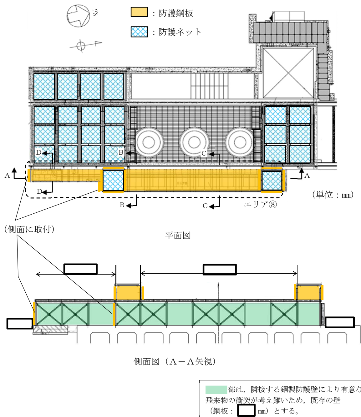
図 2-6 海水ポンプエリア防護対策施設防護鋼板の構造図(1/3)
