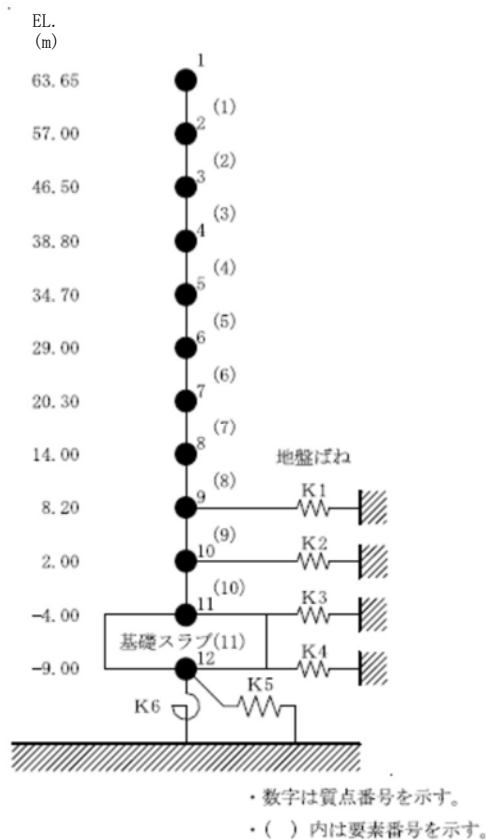
図3-15 原子炉建屋の地震応答解析モデル図
