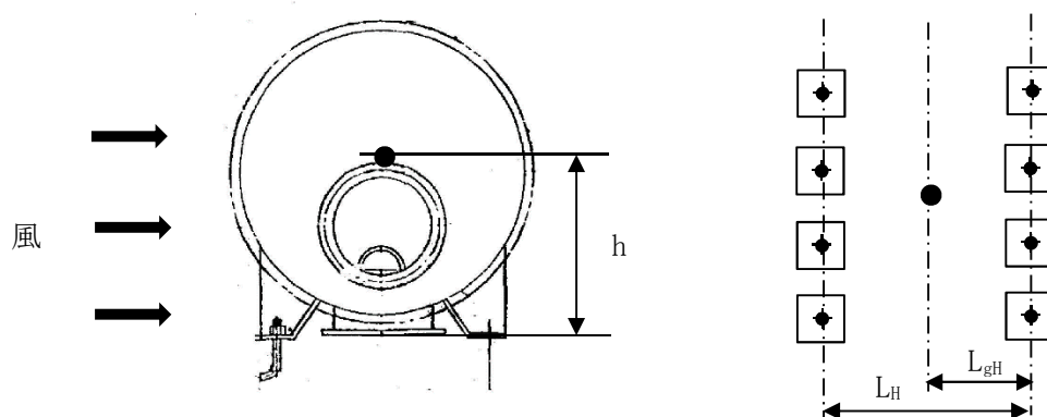
図 5-13(1/2) 非常用ディーゼル発電機 2 D 排気消音器，高圧炉心スプレイ系ディーゼル発電機排気消音器の評価モデル図 (フィルタ部軸直角方向)
