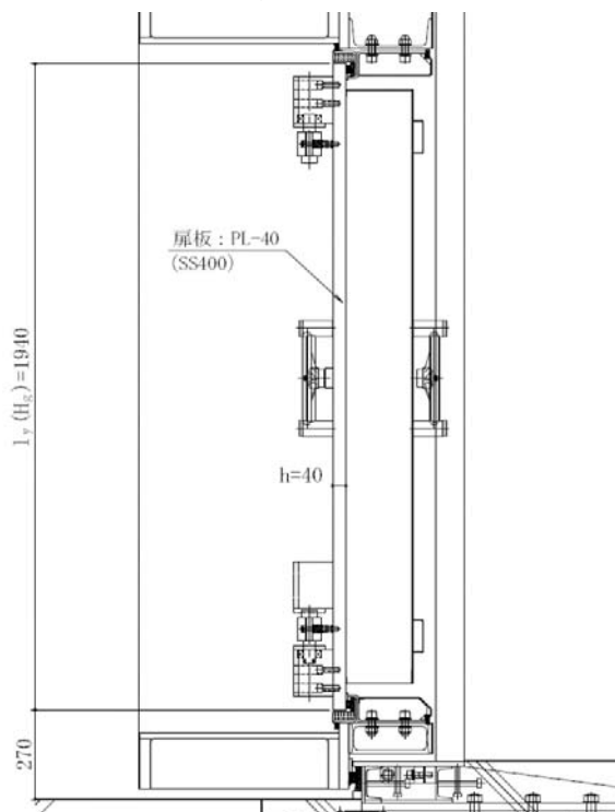
<扉立面図>
