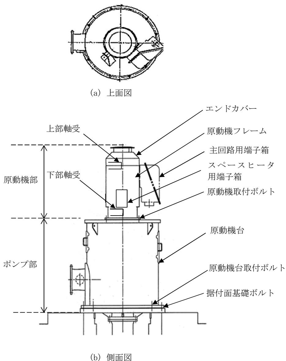
図2-2 ディーゼル発電機用海水ポンプの概要図
