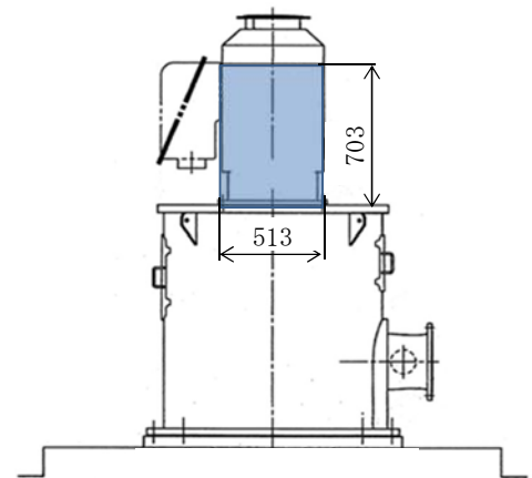
図3-16 原動機フレームの受圧部図
