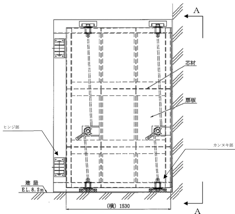
< 扉立面図 >
