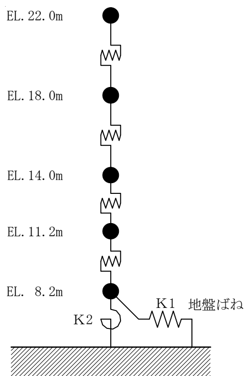
図3-4 サービス建屋の解析モデル図
