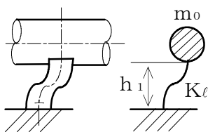
図 4-1 長手方向の固有周期 計算モデル
