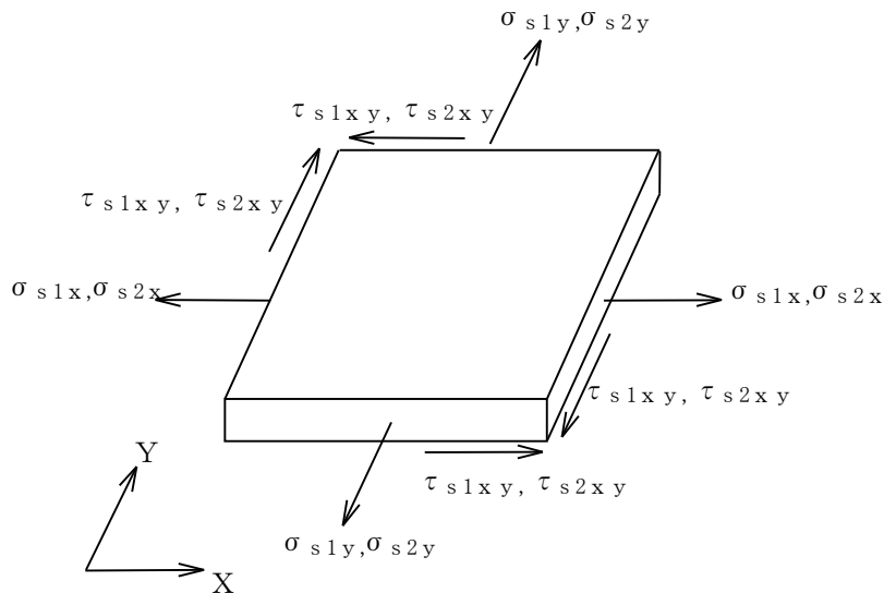
図 5-2 脚の応力計算モデル
