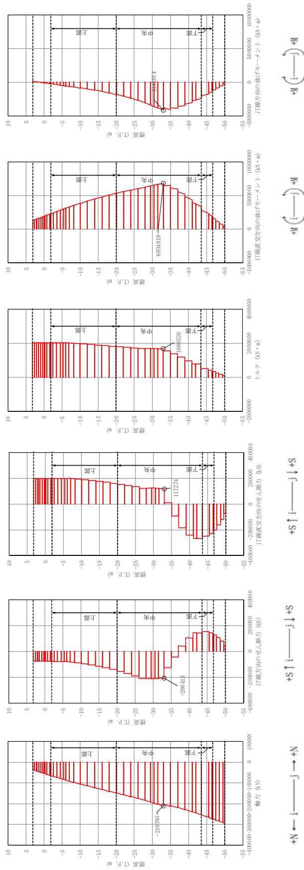
図 5.2-9 (7) 地中連続壁基礎において鉄筋の曲げ軸力照査結果が最も厳しい断面力 ①-①断面, ③-③断面 (重畳時: 敷地に遡上する津波, 南-中央, 地盤バネ 5)
