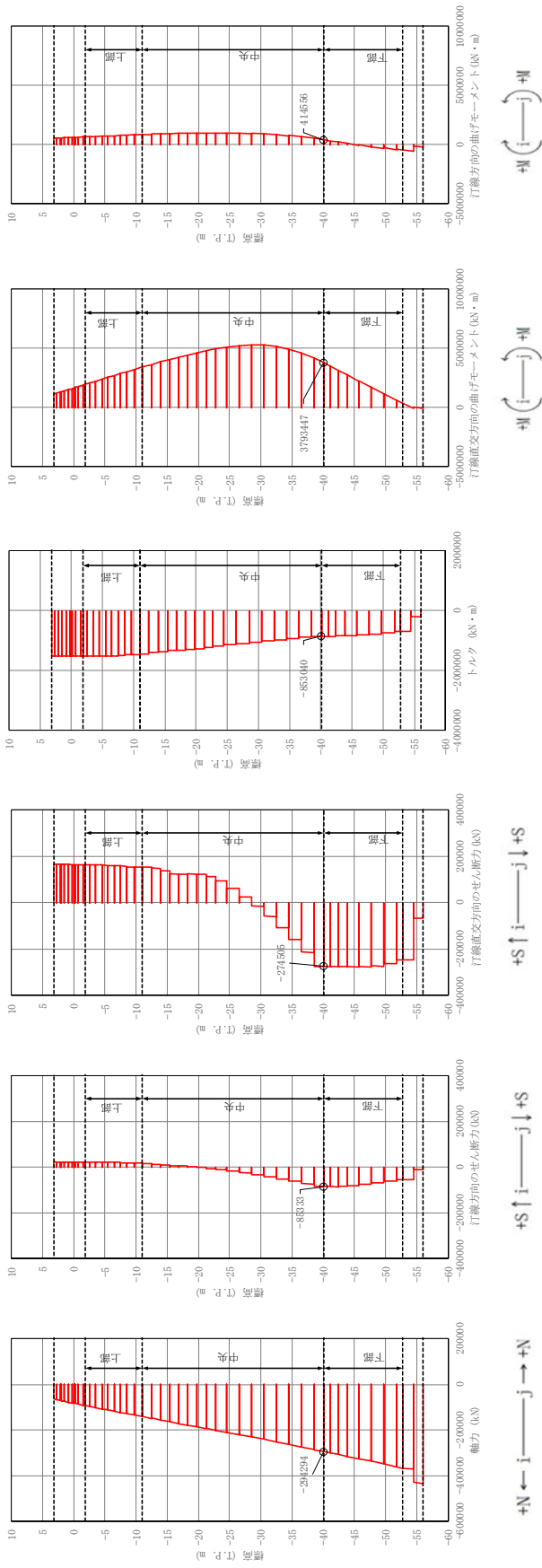
図 5.2-10 (12) 地中連続壁基礎においてせん断力照査結果が最も厳しい断面力
