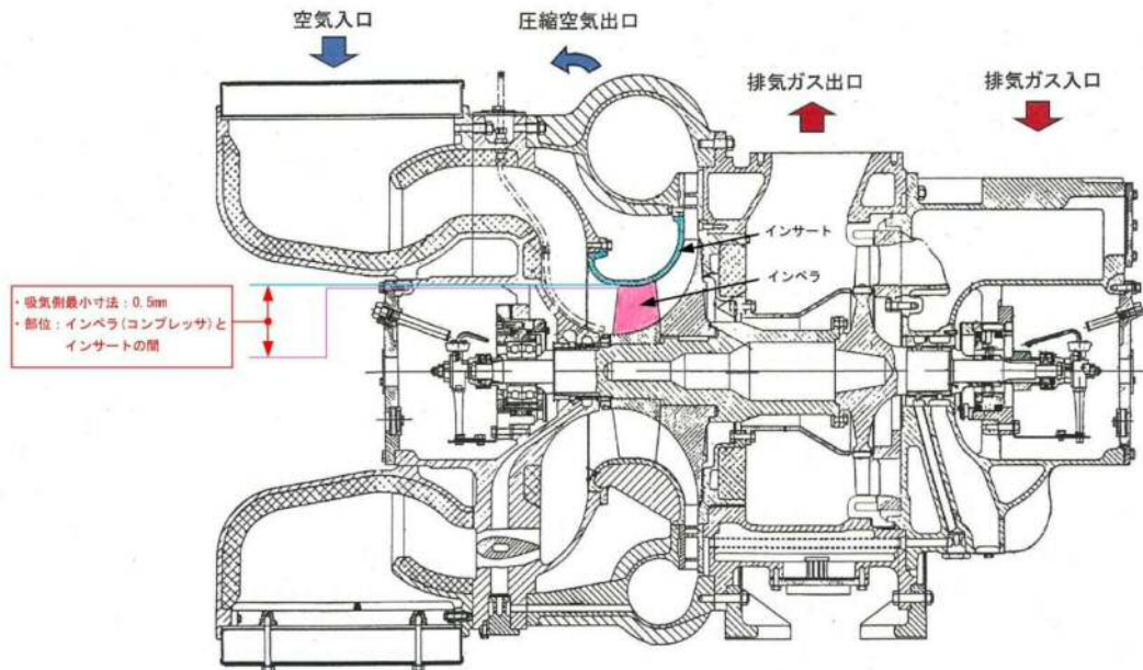
過給機断面
