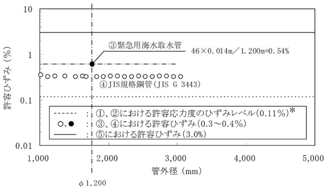
注記* : ①, ②における許容応力のひずみレベルは, 許容応力度/ヤング係数で求めた 図 13.2-1 各規格, 基準類における許容ひずみの比較
