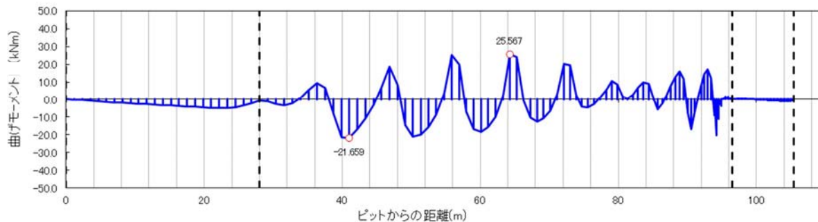
曲げモーメント図
