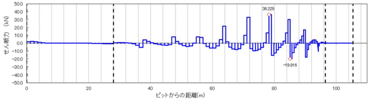
せん断力図
