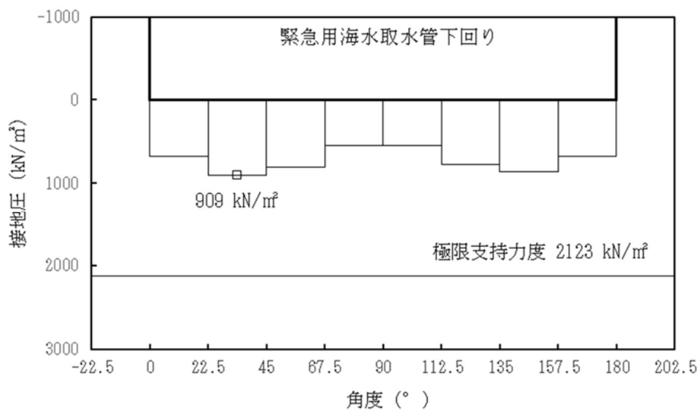
図 13.5-8 (9) ②-②断面の接地圧分布図 ( S_s-21 ) (検討ケース①：原地盤に基づく液状化強度特性を用いた解析ケース)
