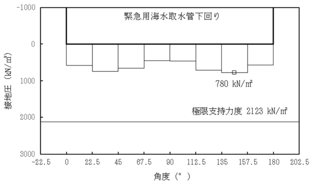
図 13.5-8 (15) ②-②断面の接地圧分布図 ( S_s-31 [H+, V+]) (検討ケース④: 敷地に存在しない豊浦標準砂の液状化強度特性により地盤を強制的に液状化させることを仮定した解析ケース)
