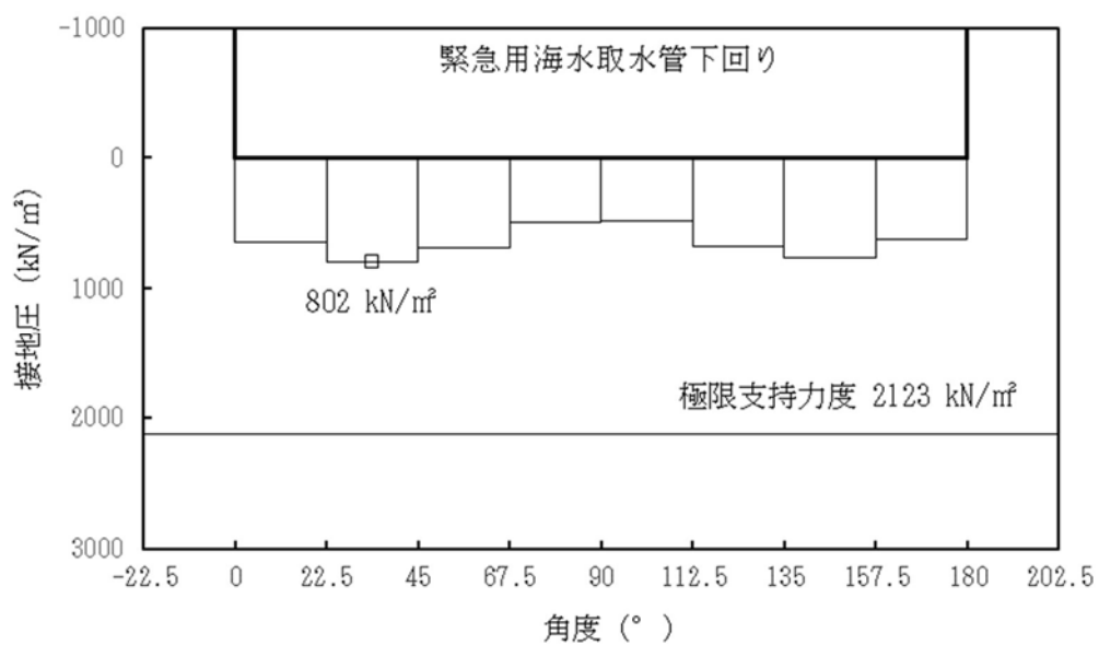
図 13.5-8 (8) ②-②断面の接地圧分布図 ( S_s-14 ) (検討ケース①：原地盤に基づく液状化強度特性を用いた解析ケース)
