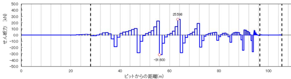
せん断力図
