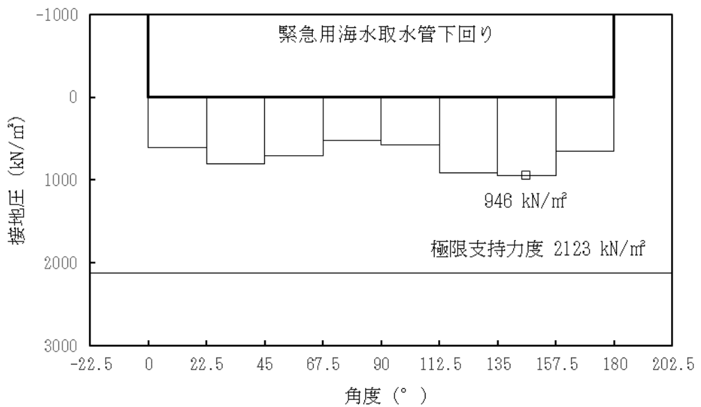
図 13.5-8 (14) ②-②断面の接地圧分布図 ( S_s-31 [H+, V+]) (検討ケース③: 地盤物性のばらつきを考慮 (-1 \sigma ) した解析ケース)
