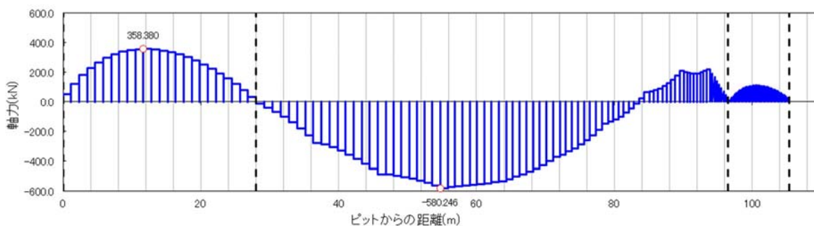
軸力図
