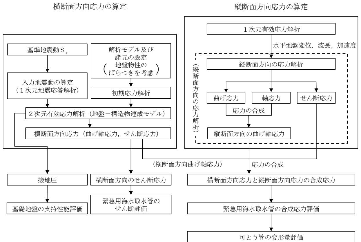
図 13.2-5 緊急用海水取水管の地震応答解析及び応力解析のフロー
