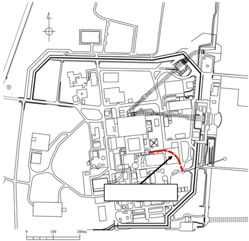
图 13.2-6 (1) 紧急用海水取水管 平面位置图 (全体图)
