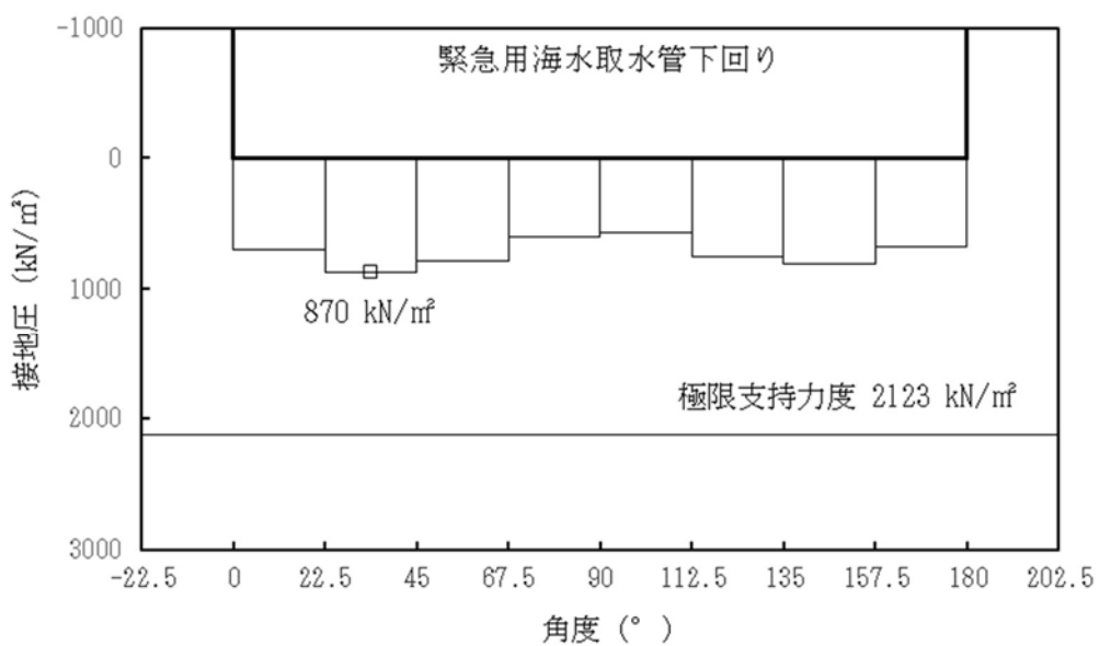
図 13.5-8 (2) ②-②断面の接地圧分布図 ( S_s-D1 [H+, V-]) (検討ケース①: 原地盤に基づく液状化強度特性を用いた解析ケース)
