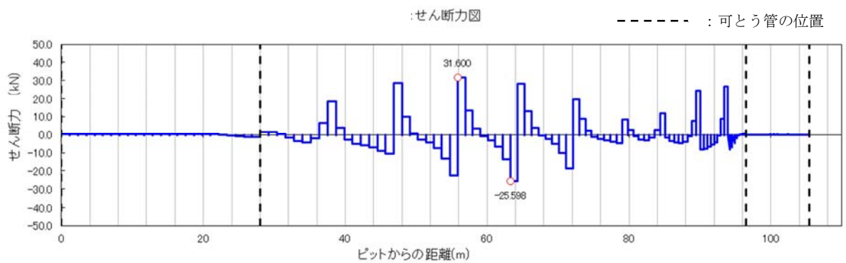
図 13.5-4 (6) 縦断面方向の断面力分布図 (軸応力最大ケース [位相 180°, 入射角 45°])
