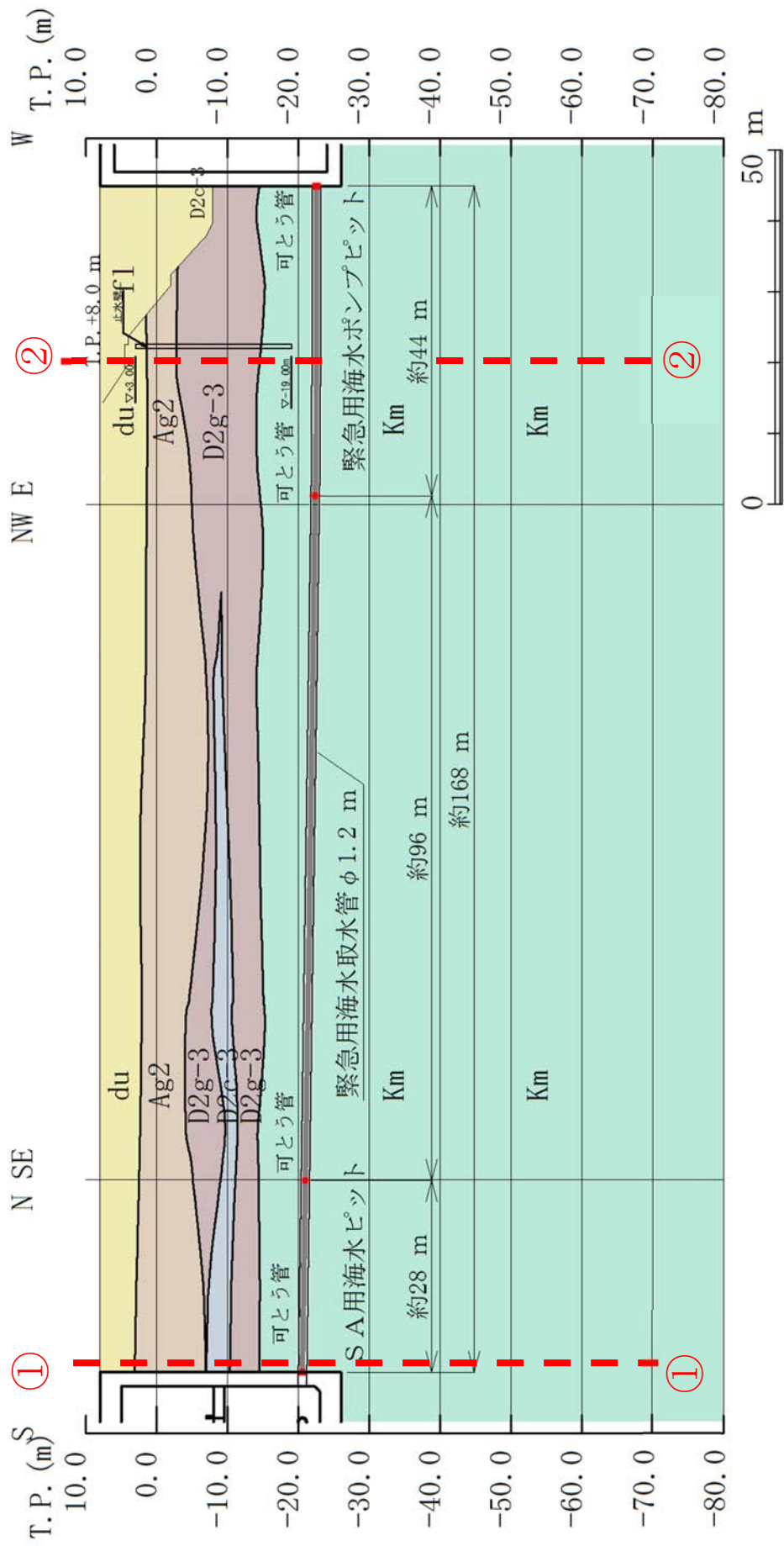
図 13.2-8 緊急用海水取水管 縦断面図 (A-A断面)
