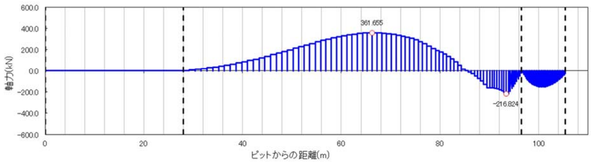
軸力図
