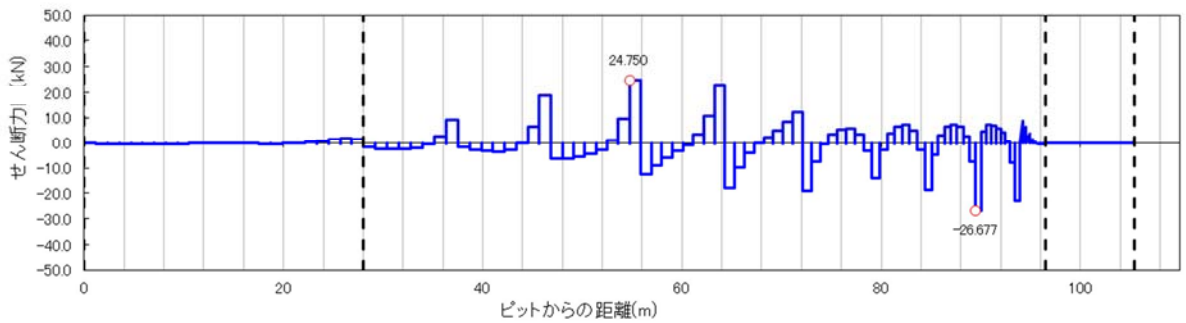
せん断力図
