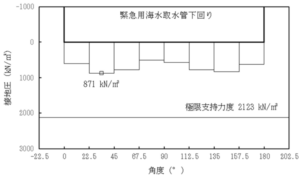
図 13.5-8 (12) ②-②断面の接地圧分布図 ( S_s-31 [H-, V+]) (検討ケース①: 原地盤に基づく液状化強度特性を用いた解析ケース)
