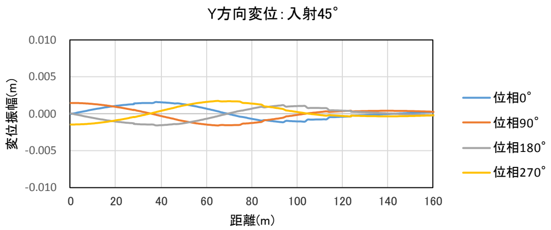
図 13.4-8 (2) 入力地盤変位 (軸応力最大ケース [入射角 45°])
