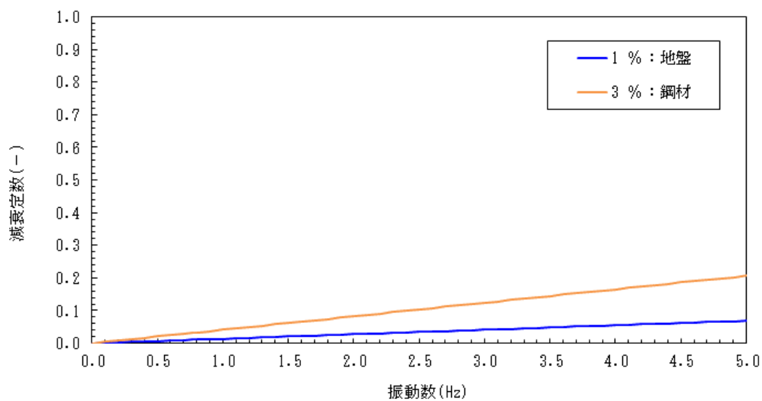
図 13-2(3) 設定した Rayleigh 減衰 (検討ケース③：地盤物性のばらつきを考慮 ( -1\sigma ) した解析ケース) (②-②断面)
