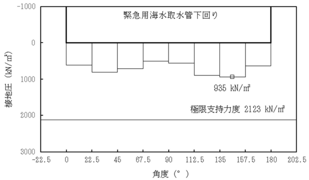
図 13.5-8 (17) ②-②断面の接地圧分布図 ( S_s-31 [H+, V+]) (検討ケース⑥: 地盤物性のばらつきを考慮 ( +1\sigma ) して非液状化の 条件を仮定した解析ケース)
