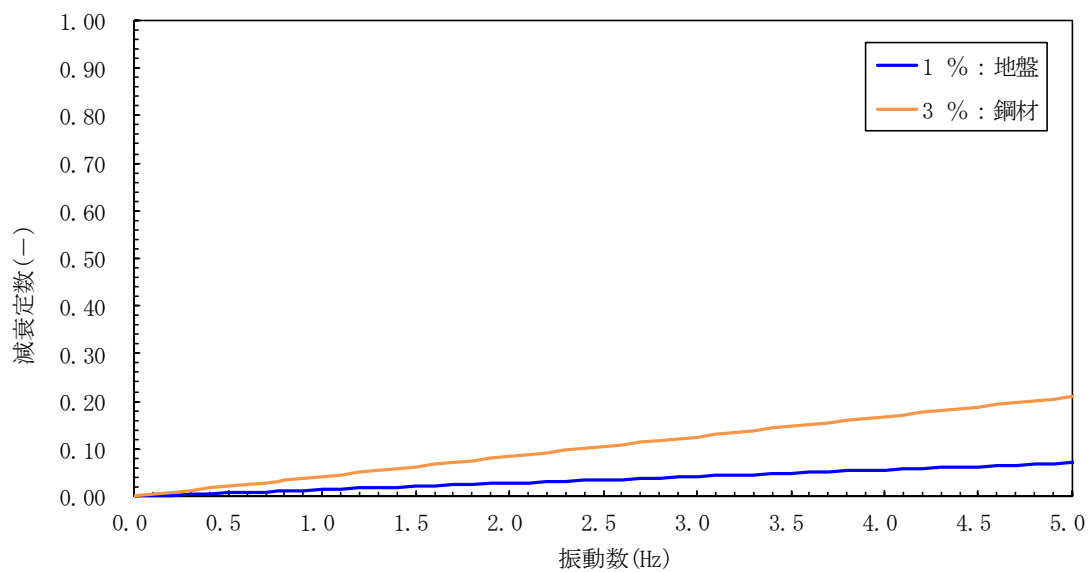
図 13-2(4) 設定した Rayleigh 減衰 (検討ケース④：敷地に存在しない豊浦標準砂の液状化強度特性により 地盤を強制的に液状化させることを仮定した解析ケース) (②-②断面)
