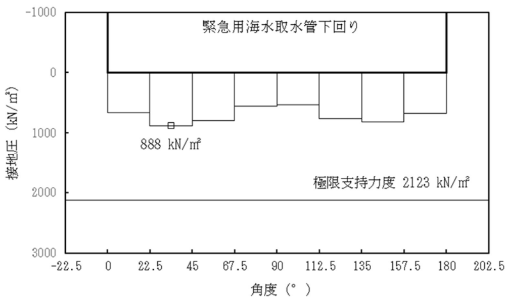
図 13.5-8 (1) ②-②断面の接地圧分布図 ( S_s-D1 [H+, V+]) (検討ケース①: 原地盤に基づく液状化強度特性を用いた解析ケース)
