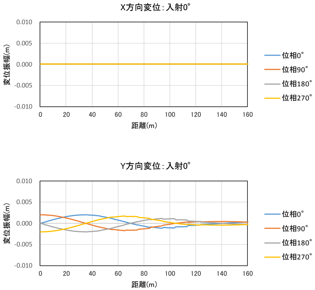
図 13.4-8 (1) 入力地盤変位 (曲げ応力最大ケース [入射角 0^\circ ])
