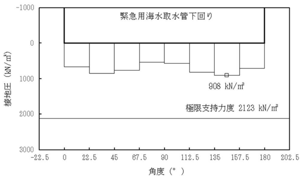
図 13.5-8 (10) ②-②断面の接地圧分布図 ( S_s-22 ) (検討ケース①：原地盤に基づく液状化強度特性を用いた解析ケース)
