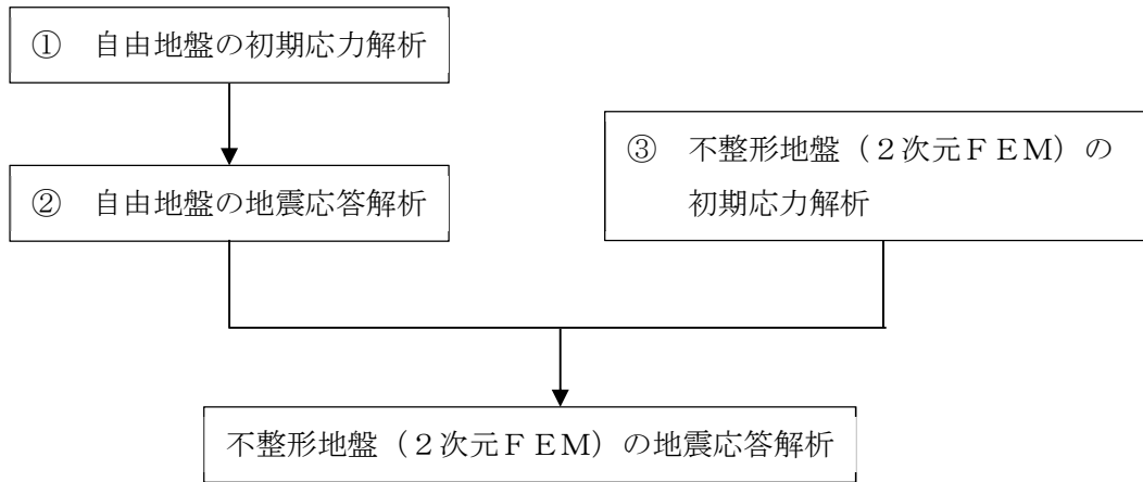
図 13.3-3 自由地盤の初期応力解析から不整形地盤 (2次元FEM) の地震応答解析までのフロー
