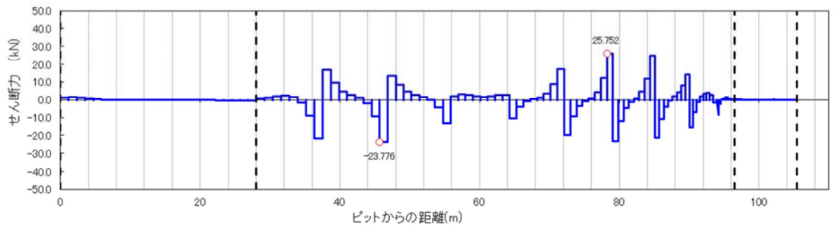
図 13.5-4 (8) 縦断面方向の断面力分布図 (軸応力最大ケース [位相 270°, 入射角 45°])
