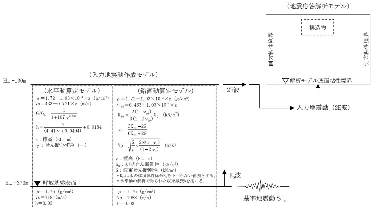
図 13.3-11 入力地震動算定の概念図
