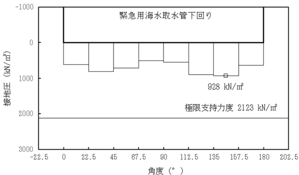
図 13.5-8 (16) ②-②断面の接地圧分布図 ( S_s-31 [H+, V+]) (検討ケース⑤: 原地盤において非液状化の条件を仮定した解析ケース)
