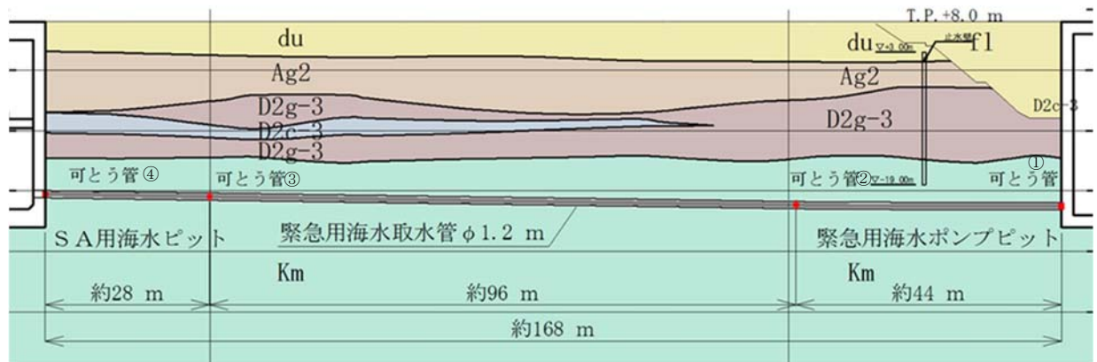
図13-4 可とう管位置図
