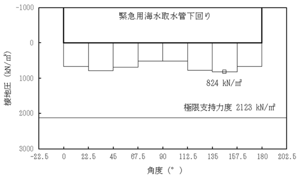
図 13.5-8 (6) ②-②断面の接地圧分布図 ( S_s-12 ) (検討ケース①: 原地盤に基づく液状化強度特性を用いた解析ケース)
