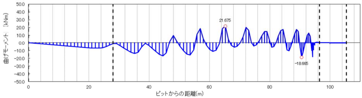
曲げモーメント図
