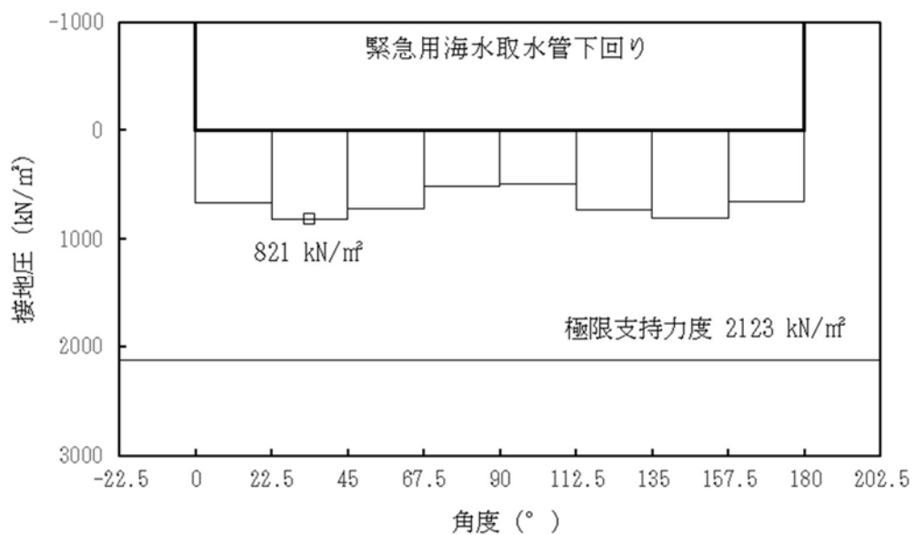
図 13.5-8 (7) ②-②断面の接地圧分布図 ( S_s-13 ) (検討ケース①：原地盤に基づく液状化強度特性を用いた解析ケース)
