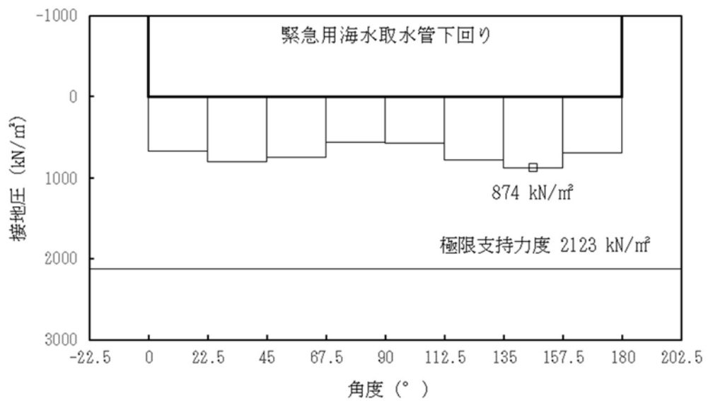
図 13.5-8 (4) ②-②断面の接地圧分布図 ( S_s-D1 [H-, V-]) (検討ケース①: 原地盤に基づく液状化強度特性を用いた解析ケース)
