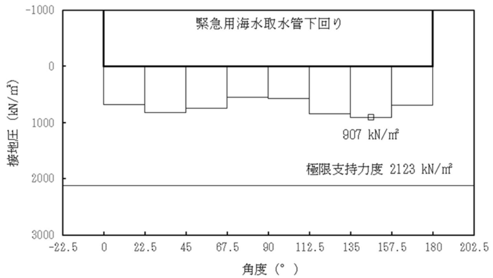
図 13.5-8 (3) ②-②断面の接地圧分布図 ( S_s-D1 [H-, V+]) (検討ケース①: 原地盤に基づく液状化強度特性を用いた解析ケース)
