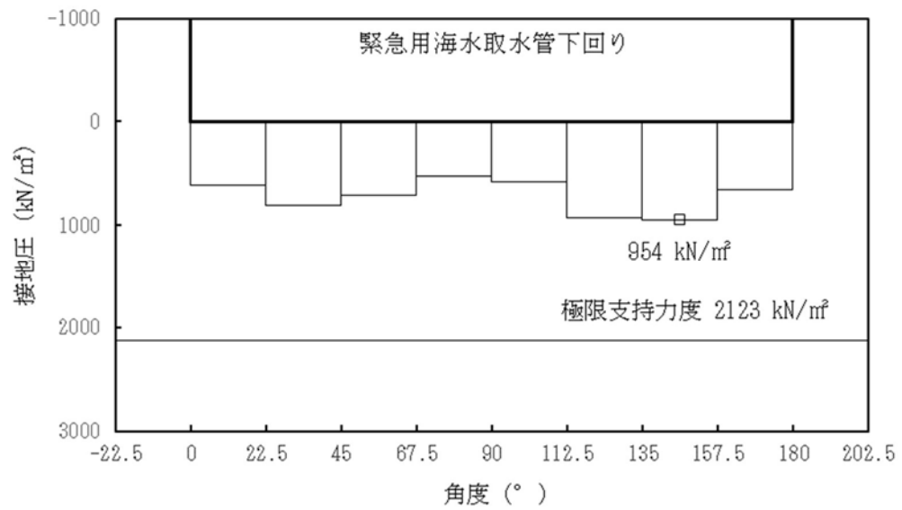
図 13.5-8 (11) ②-②断面の接地圧分布図 ( S_s-31 [H+, V+]) (検討ケース①: 原地盤に基づく液状化強度特性を用いた解析ケース)
