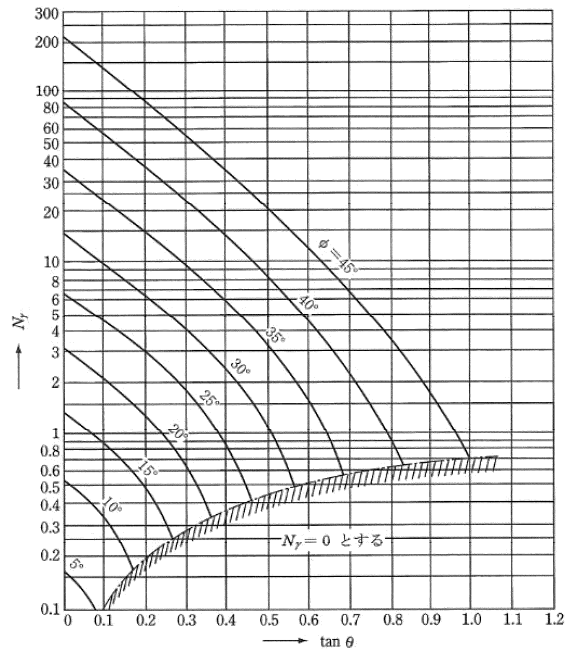
図 13.2-12 支持力係数 N_y を求めるグラフ
