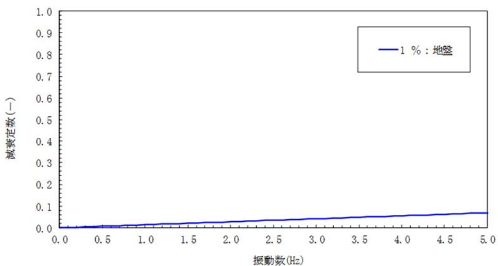
図 13-3(2) 設定した Rayleigh 減衰 (検討ケース②：地盤物性のばらつきを考慮 (+1σ) した解析ケース) (②-②断面)
