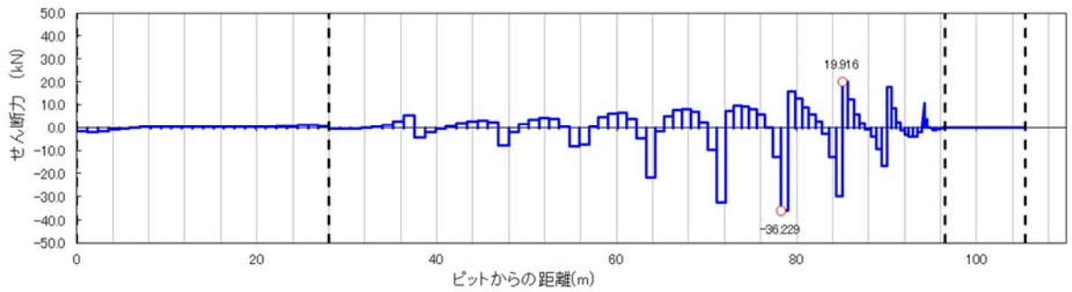
図 13.5-4 (3) 縦断面方向の断面力分布図 (曲げ応力最大ケース [位相 90°, 入射角 0°])
