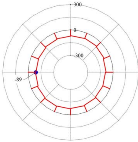
軸力図 (kN/m)
