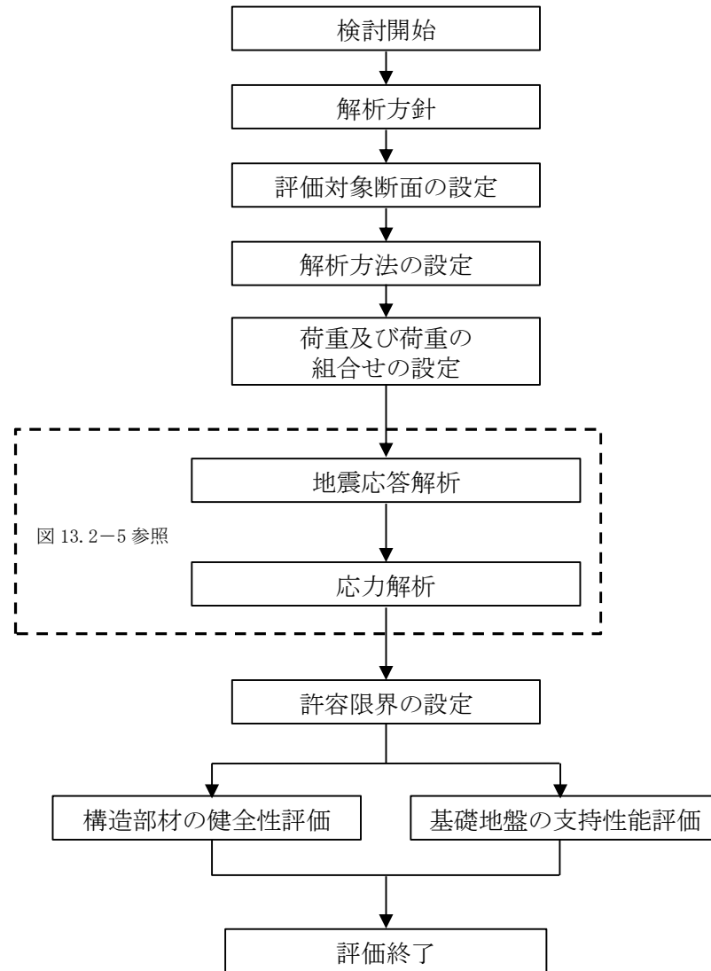
図 13.2-4 緊急用海水取水管の耐震評価フロー
