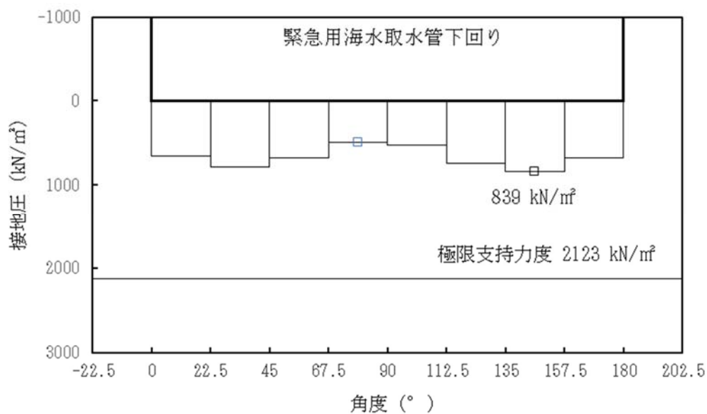
図 13.5-8 (5) ②-②断面の接地圧分布図 ( S_s-11 ) (検討ケース①: 原地盤に基づく液状化強度特性を用いた解析ケース)
