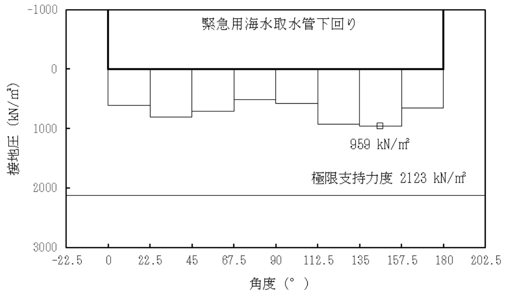
図 13.5-8 (13) ②-②断面の接地圧分布図 ( S_s-31 [H+, V+]) (検討ケース②: 地盤物性のばらつきを考慮 (+1 \sigma ) した解析ケース)
