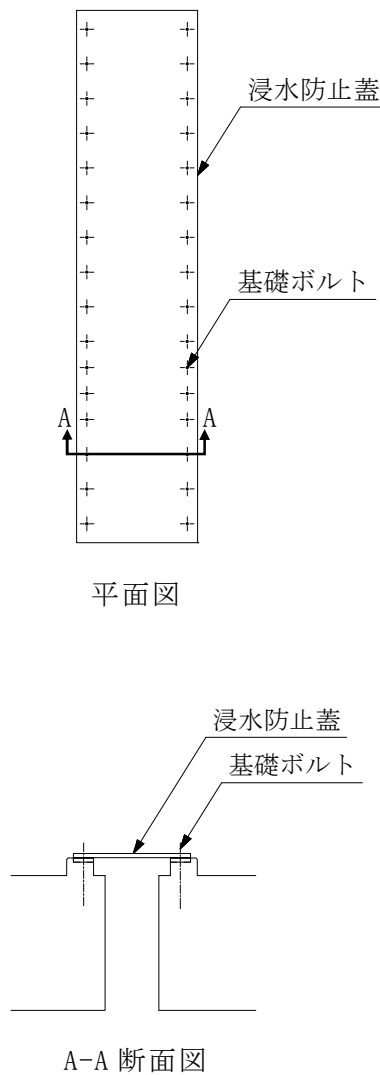
図 3-1 評価部位（蓋 1, 10）
