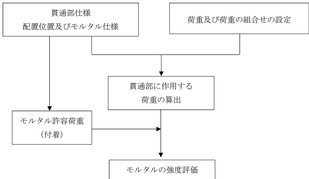
図 2-6 モルタルの強度評価フロー
