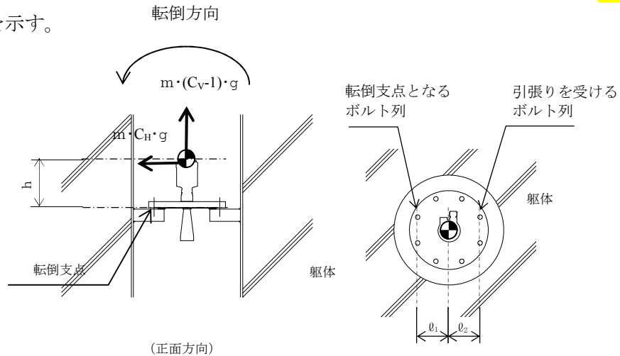
図 5.4-1 計算モデル
