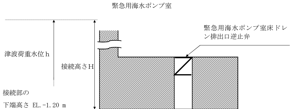
図5-1 緊急用海水ポンプ室床ドレン排出口逆止弁の動水圧の算出に用いるHの設定
