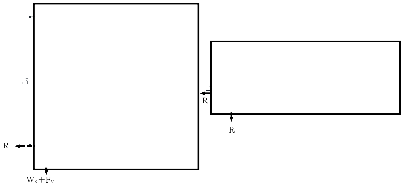
図4.4-1 ヒンジ部に生じる荷重の例
