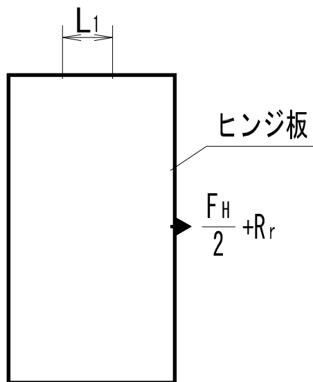
図 8.4-2 ヒンジ板に生じる荷重の例
