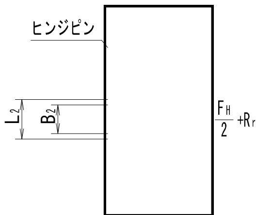
図 8.4-3 ヒンジピンに生じる荷重の例
