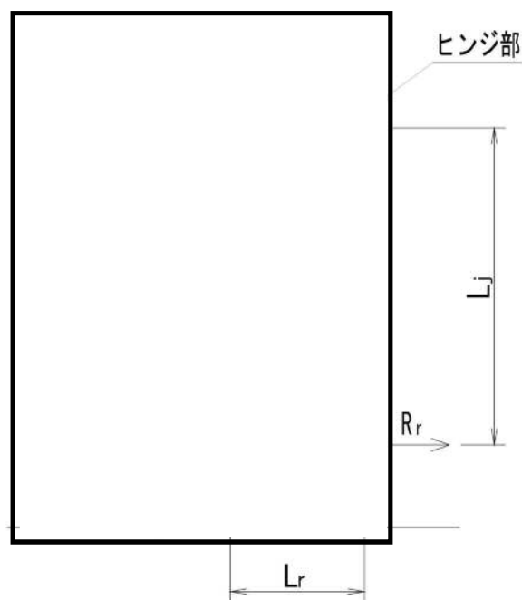
図 5.4-1 ヒンジ部に生じる荷重の例
