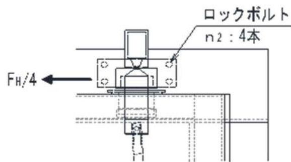
図10.4-7 ロックボルトに生じる荷重の例
