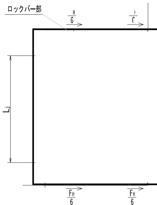
図 8.4-5 ロックバー部に生じる荷重の例
