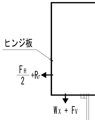
図 6.4-2 ヒンジ板に生じる荷重の例
