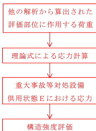
図2-1 胴アンカー部の強度評価フロー
