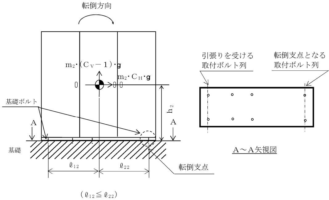
図2-3(1) 計算モデル (直立形 長辺方向転倒の場合)
