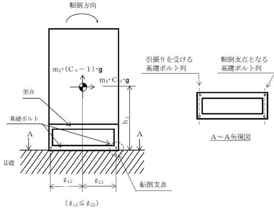
図1-2(1) 計算モデル
