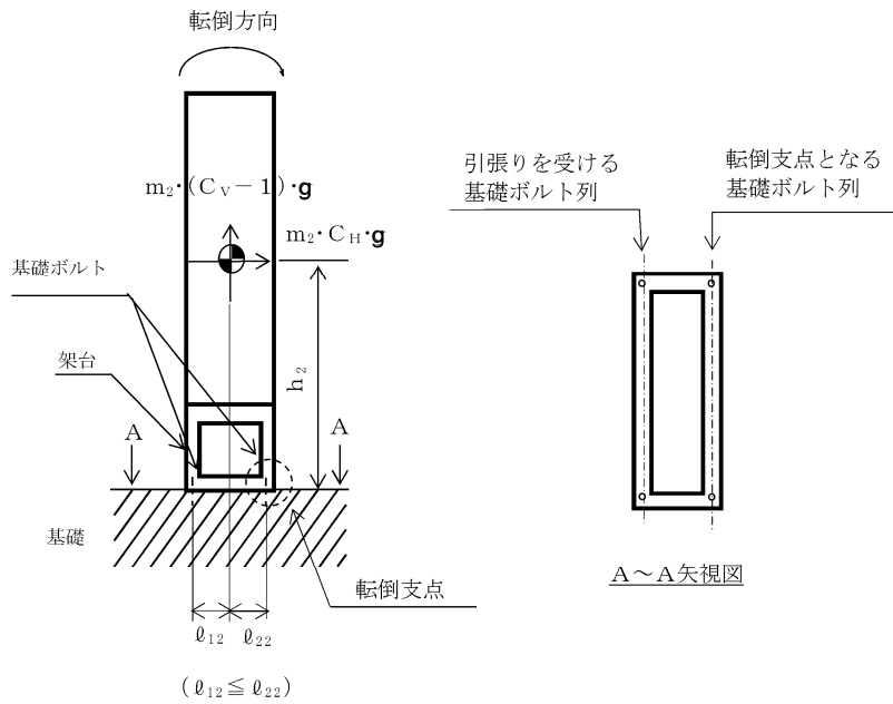
図1-2(2) 計算モデル
