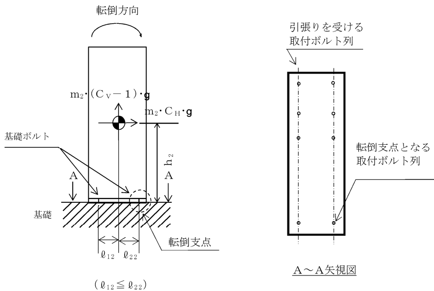
図2-3(2) 計算モデル (直立形 短辺方向転倒の場合)
