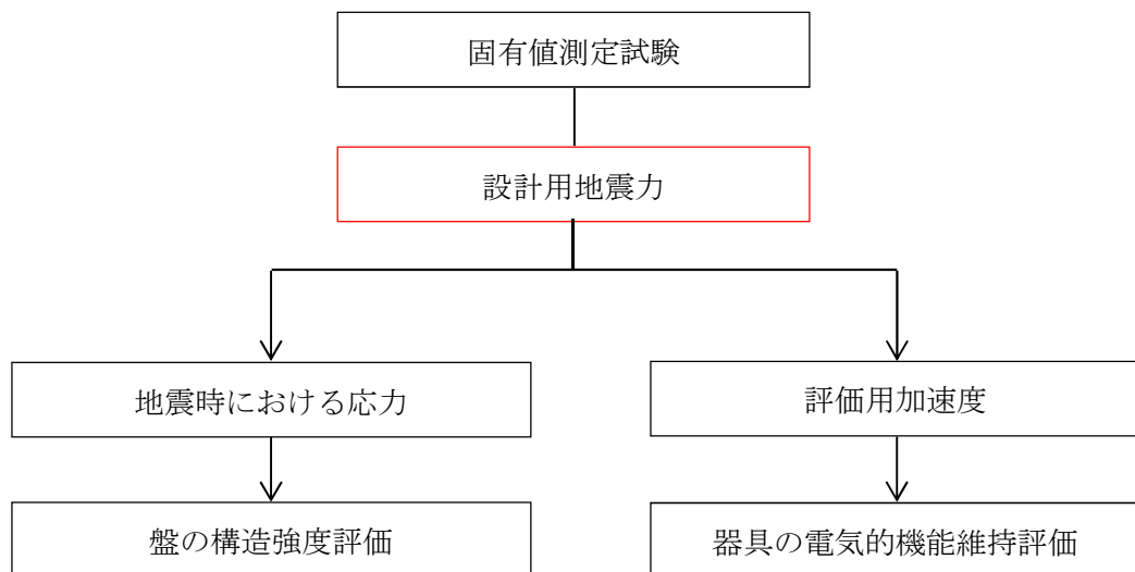
図 2-1 盤の耐震評価フロー
