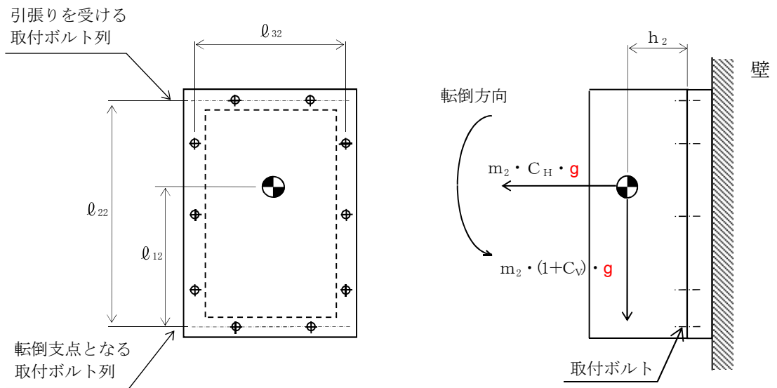
図 5-5(3) 計算モデル (壁掛形 水平方向転倒の場合)
