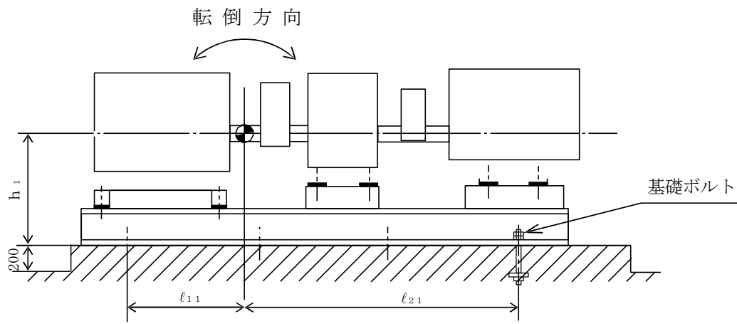
A~A矢視図 (基礎ボルト)
