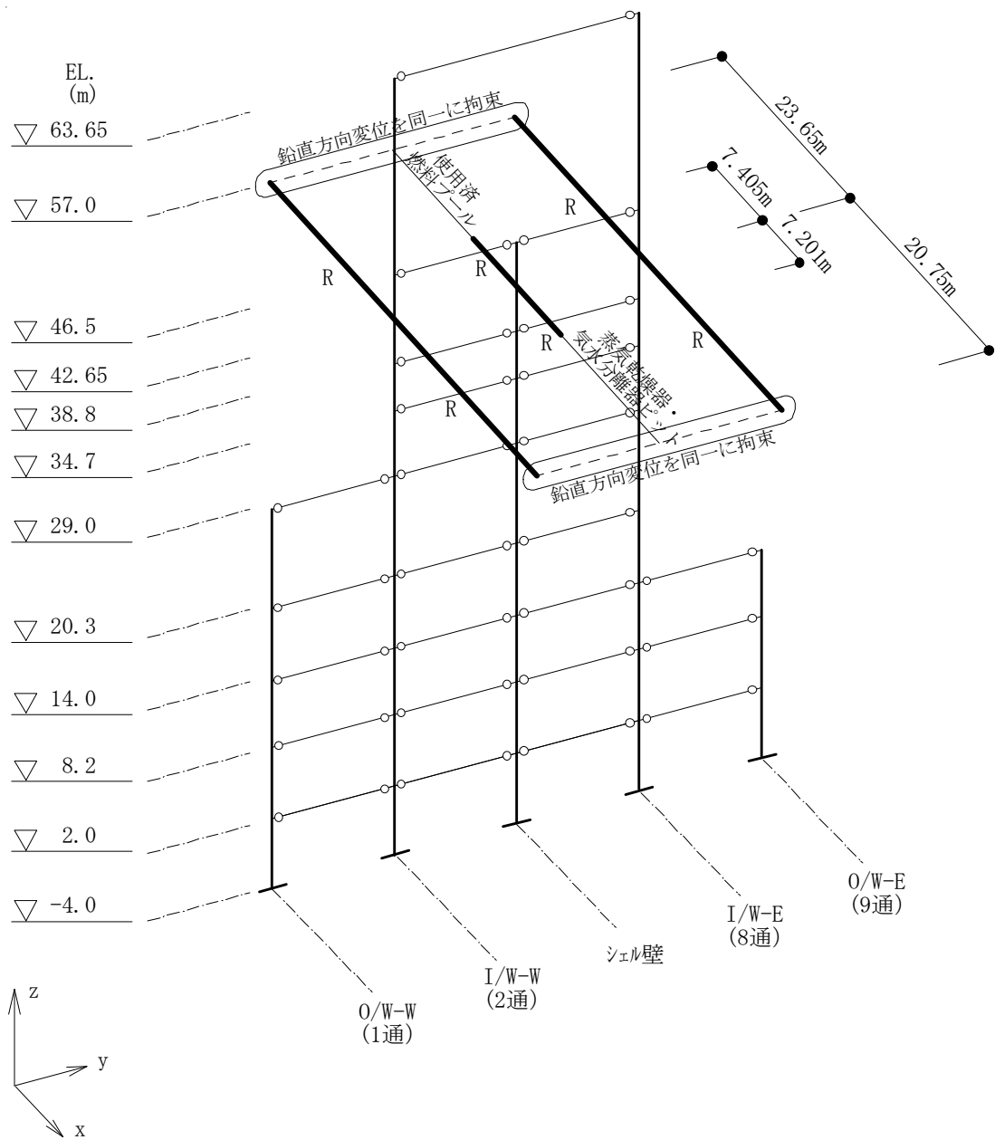
(a) NS 方向モデル
