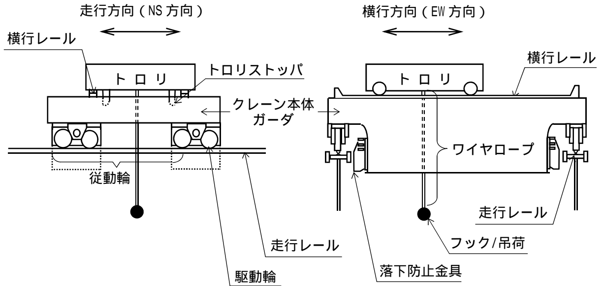
図 4-1 構造概要図
