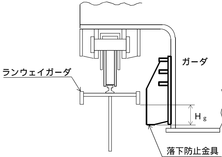
図 4-10 許容浮上り量 H_g の概要図
