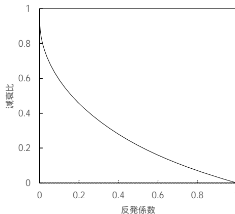
図 4-3 反発係数と減衰比の関係
