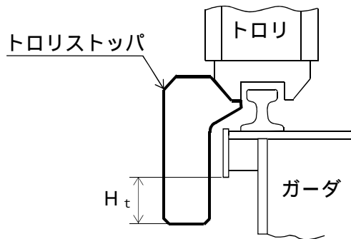
図 4-11 許容浮上り量 H_t の概要図
