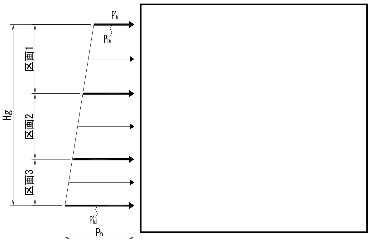
縦桁に生じる荷重の例
