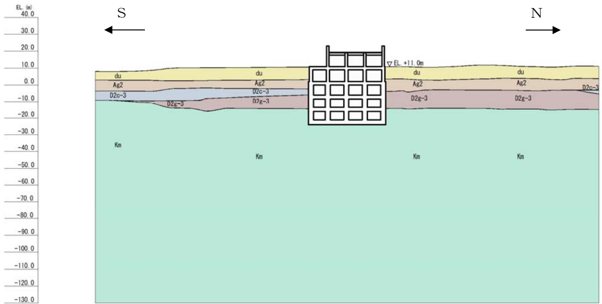
第3-2図 電源装置置場の評価対象断面図（南北方向断面）
