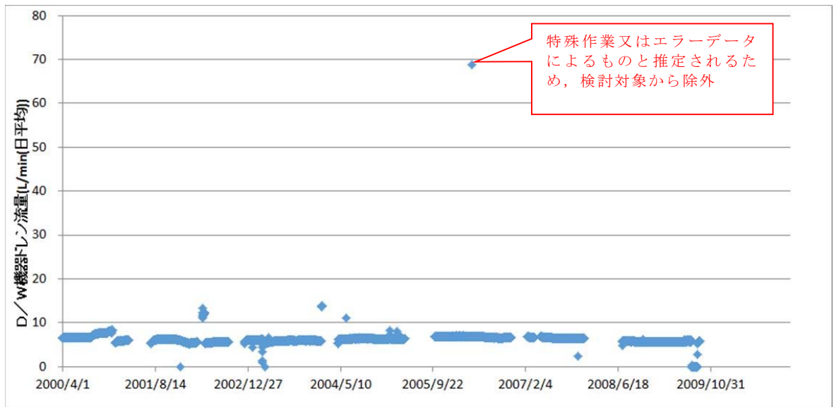
第 1 図 通常運転中のドライウェル機器ドレン流量計の実績データ
