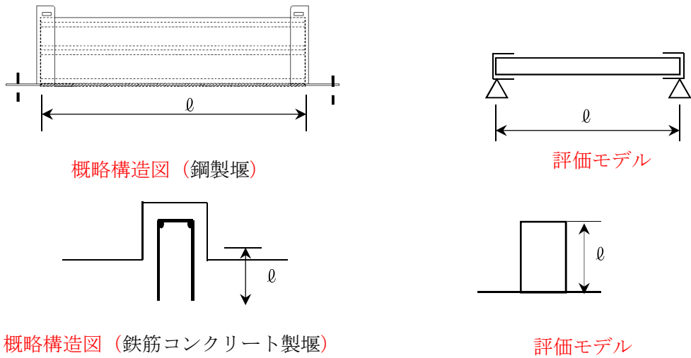
図3-1 鉄筋コンクリート製堰及び鋼製堰の評価モデル図
